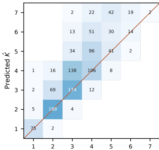
RoPE-TOA+Bias
