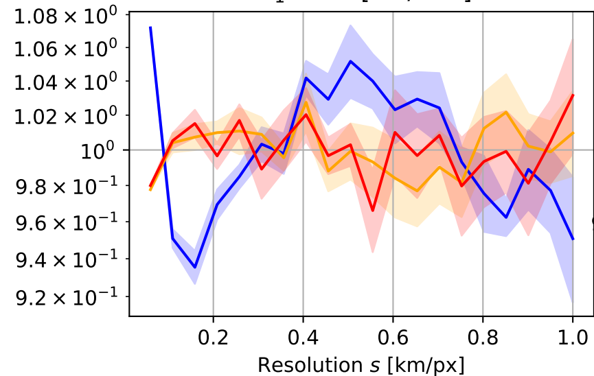
m_1 error [km/km 2 ]
