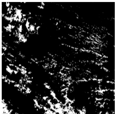
0.06 km/px - (5000, 5000)
