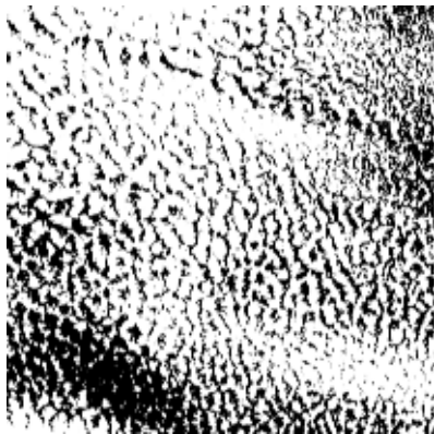
0.06 km/px - (5000, 5000)
