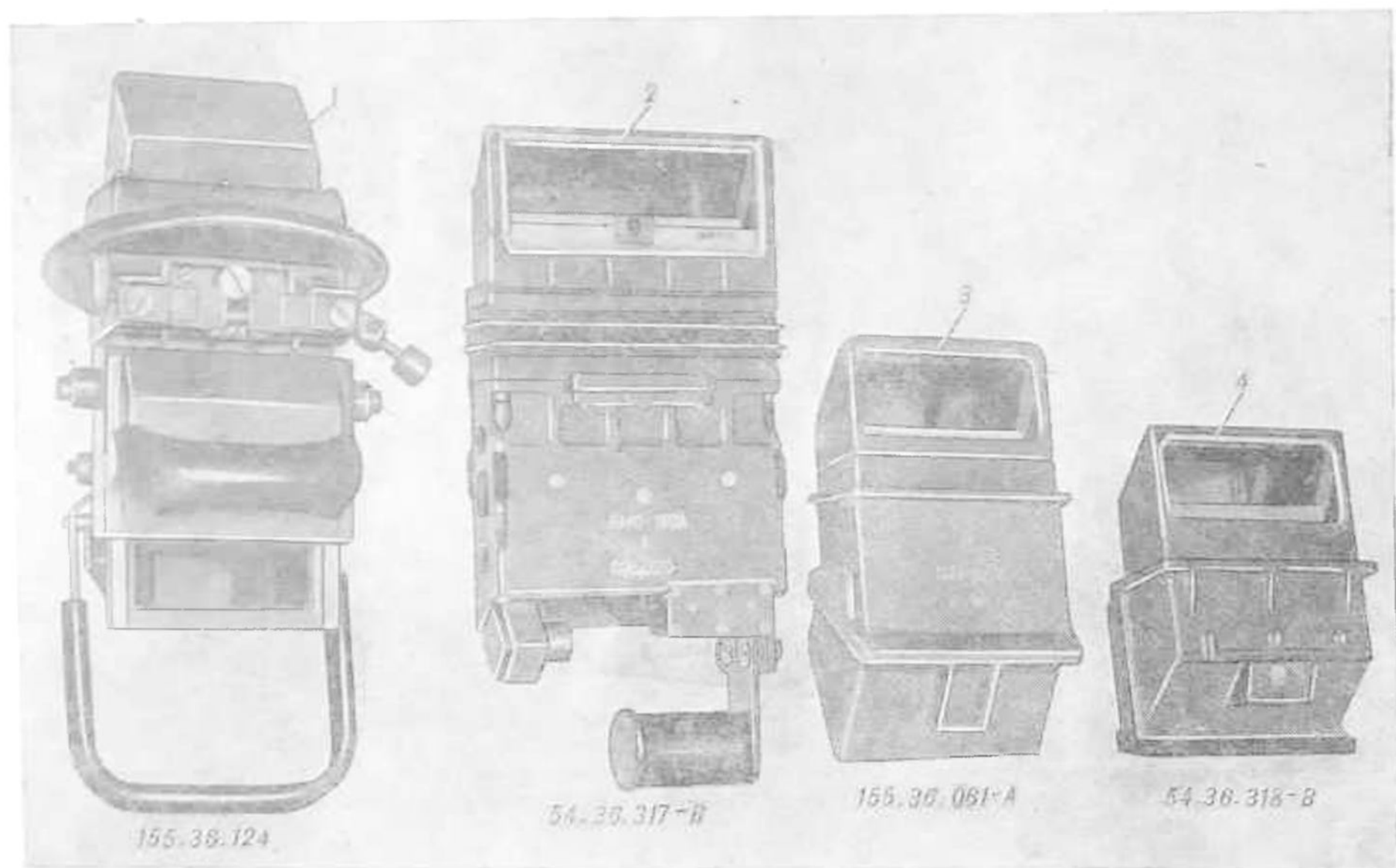
Рис. 130. Призменные приборы наблюдения
