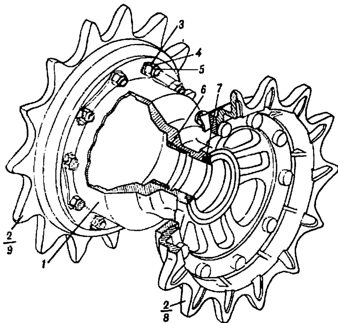
Рис. 30. Ведущее колесо (54.11сб-4Г для гусеницы с открытым шарниром и 613.11сб-5 для гусеницы с резинометаллическим шарниром)
