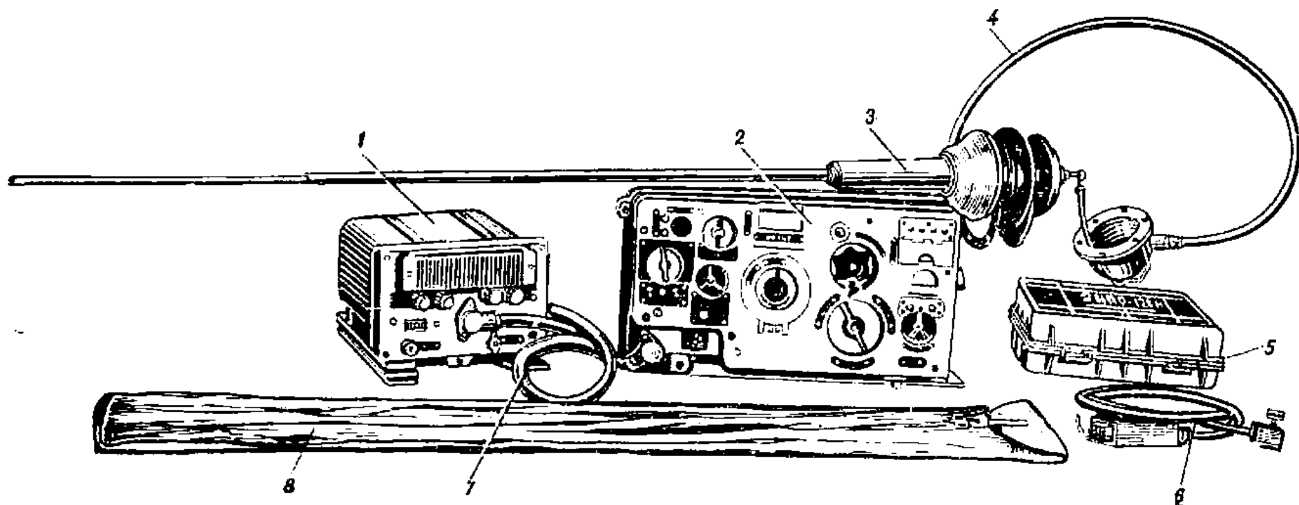
Рис. 117. Комплект радиостанции Р-123М и нагрудный переключатель
