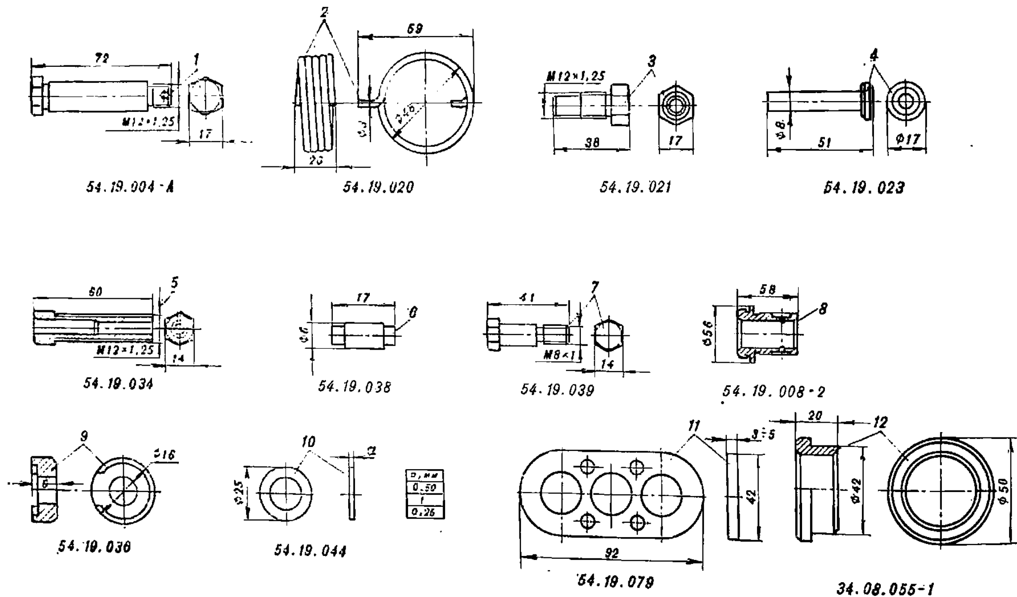
Рис. 46. Детали привода управления коробкой передач
