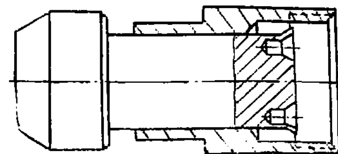
Рис. 184. Гайка для выбивания пальцев (613.28.44сб-А)
