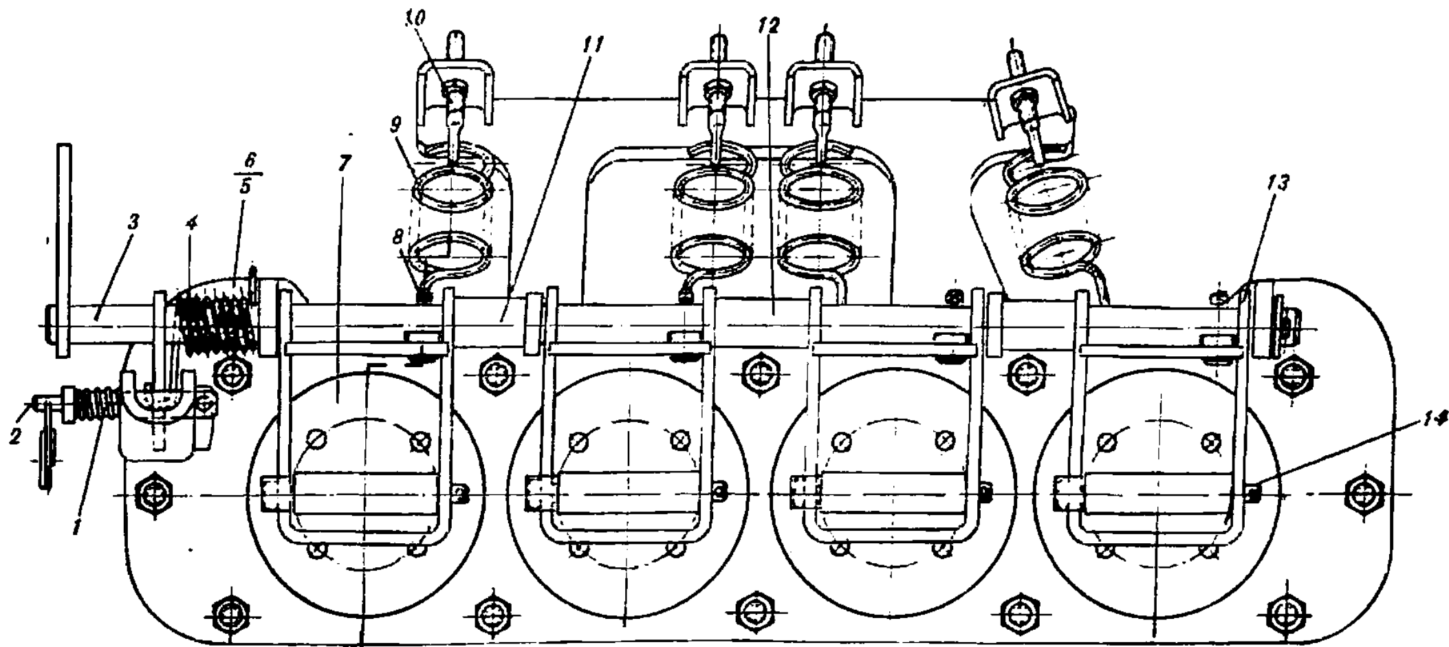
Рис. 160. Клапаны выпускные (54.83.21с6-1А)
