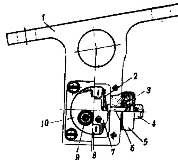
Рис. 52. Кронштейн (155.21.16сб-1)
