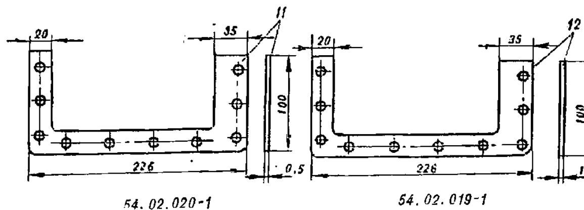
Рис. 5. Детали крепления системы охлаждения
