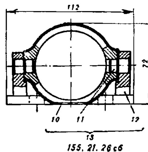
Рис. 53. Узлы привода управления главным фрикционом
