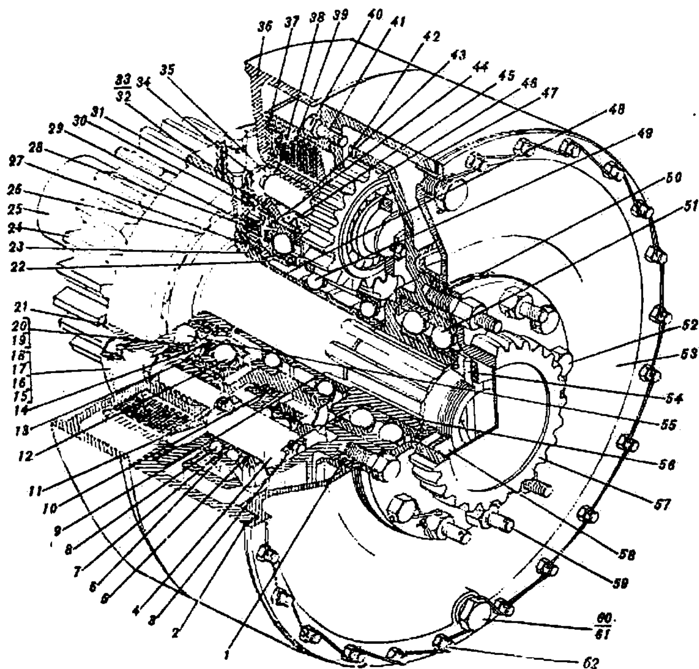
Рис. 27. Планетарный механизм поворота левый и правый (155.09сб-А)
