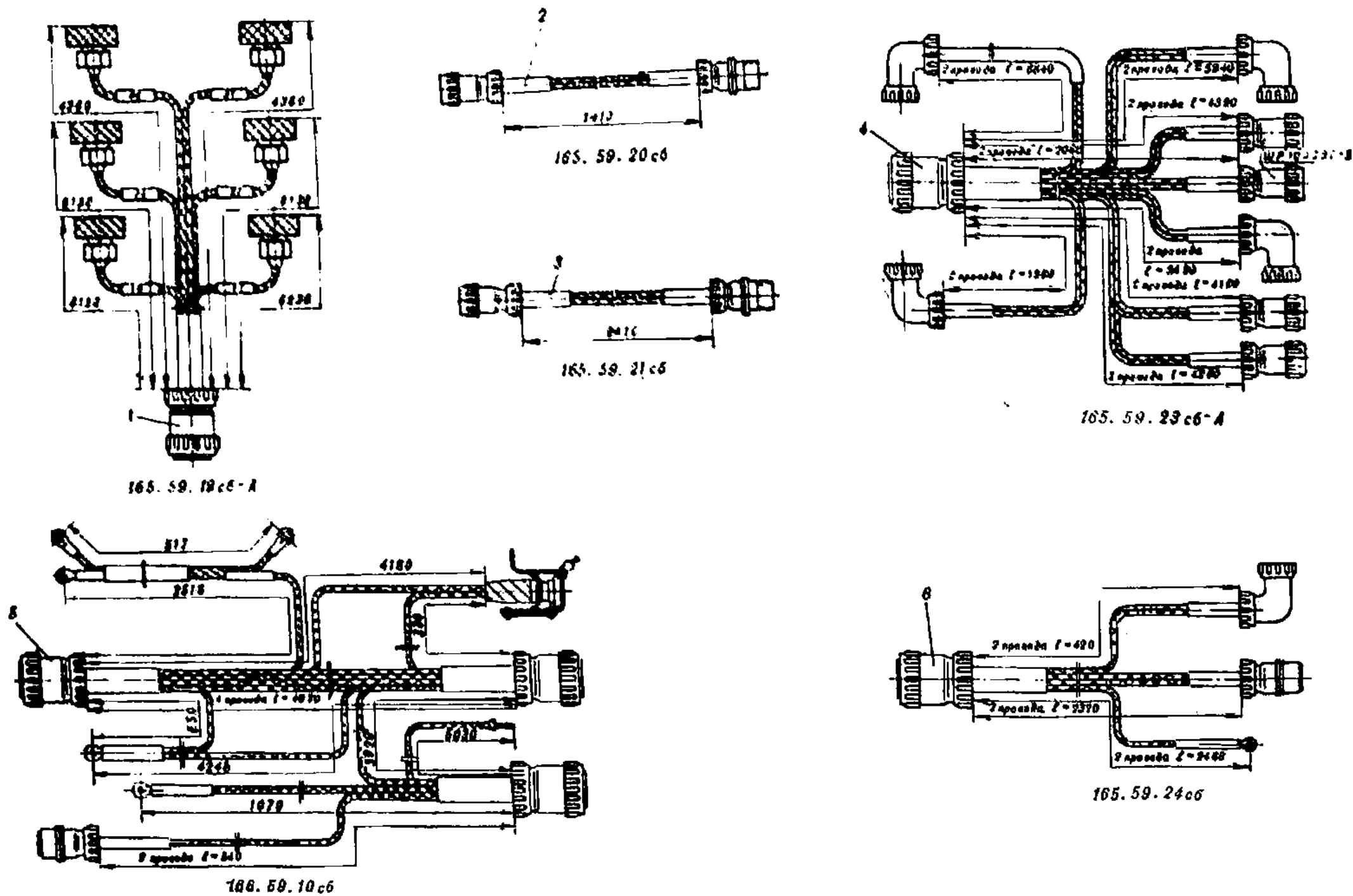
Рис. 154. Кабели системы противопожарного оборудования
