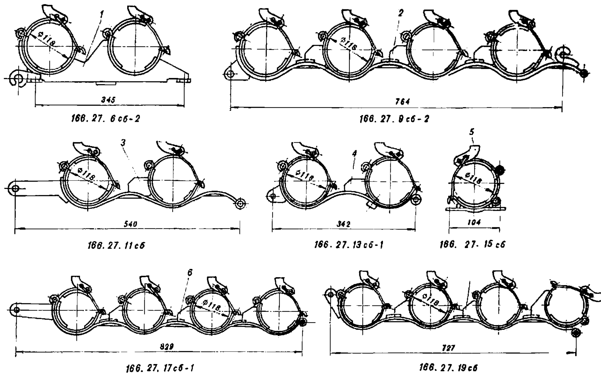
Рис. 69. Стеллажи боекомплекта
