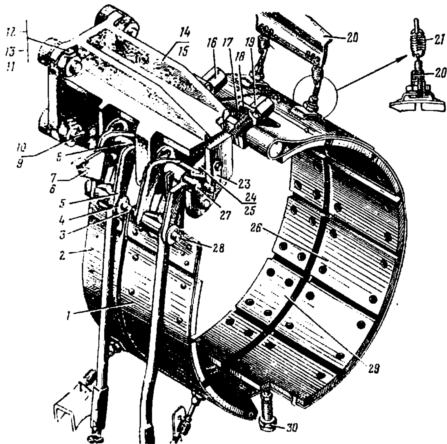
Рис. 29. Тормоза планетарного механизма поворота (165.10сб)
