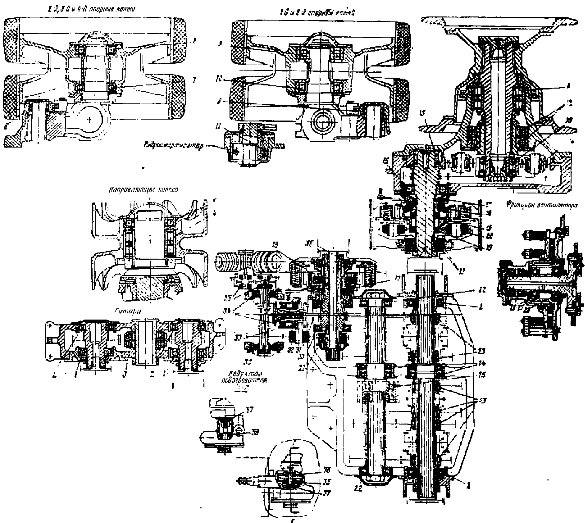
Рис. 162. Подшипники, шарики и ролики механизмов силовой передачи, ходовой части и подогревателя
