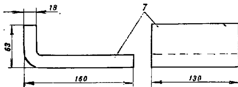
Рис. 8. Детали системы смазки
