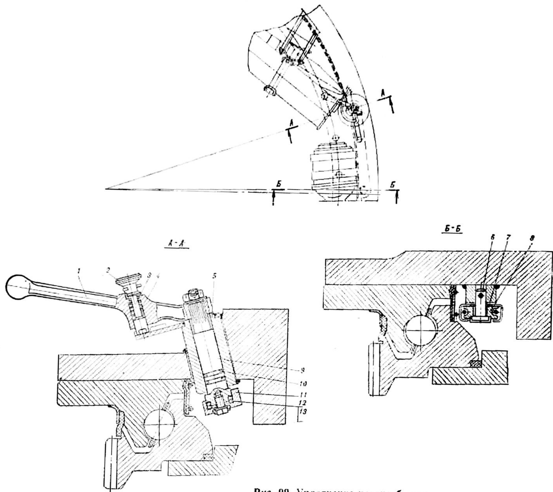
Рис. 99. Уплотнение погона башни
