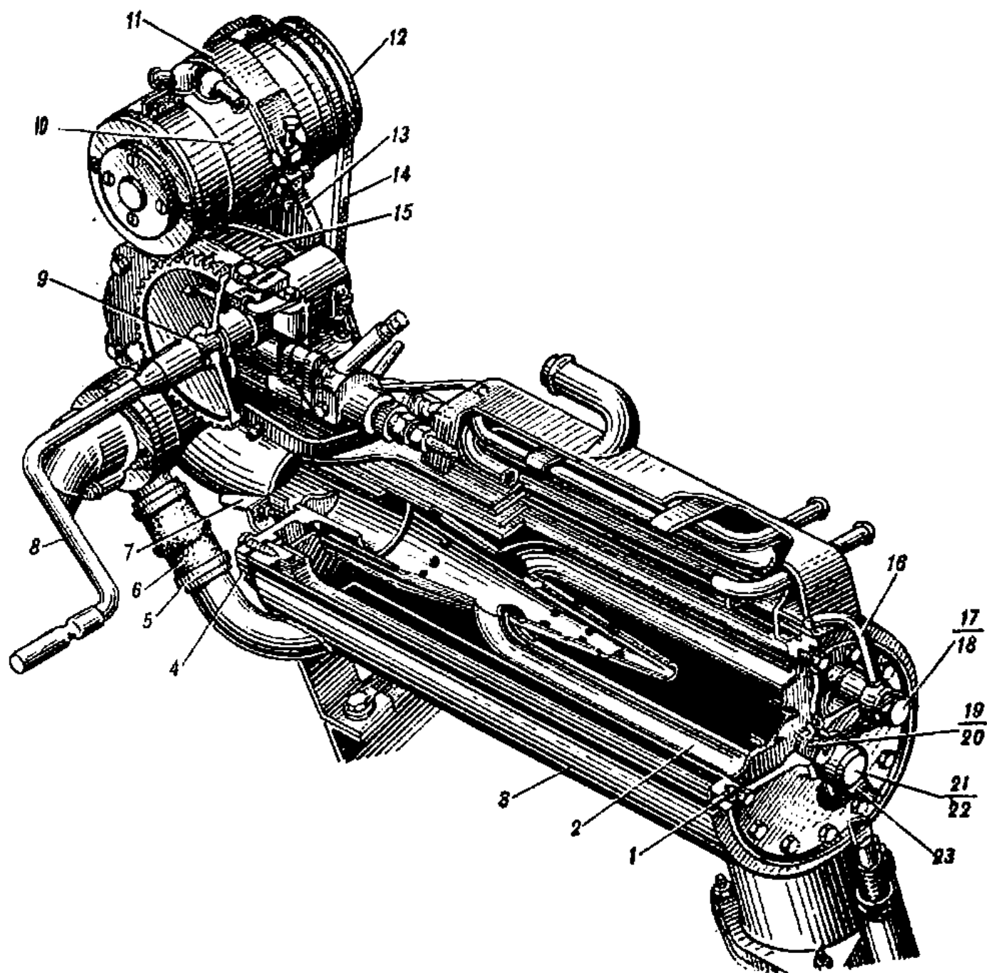
Рис. 143. Форсуночный подогреватель (166.42сб-А)
