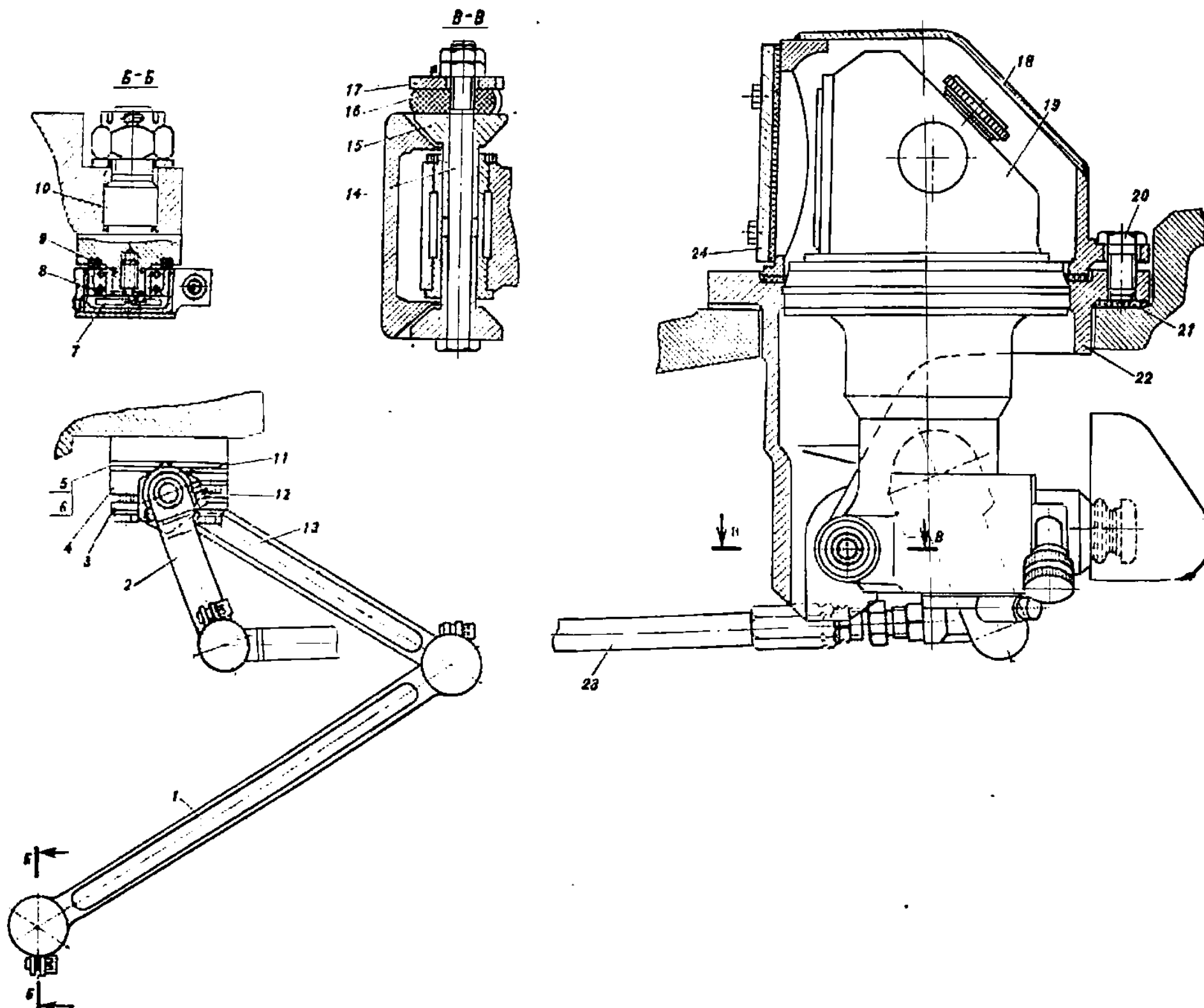
Рис. 107. Установка прибора ТПН (166.31.10сб)
