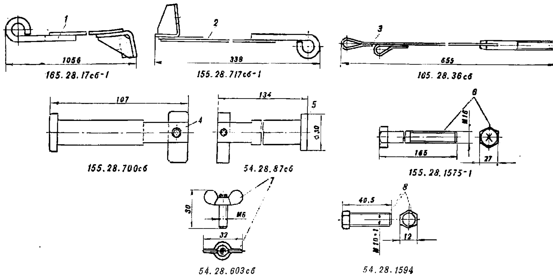
Рис. 76. Детали крепления оборудования
