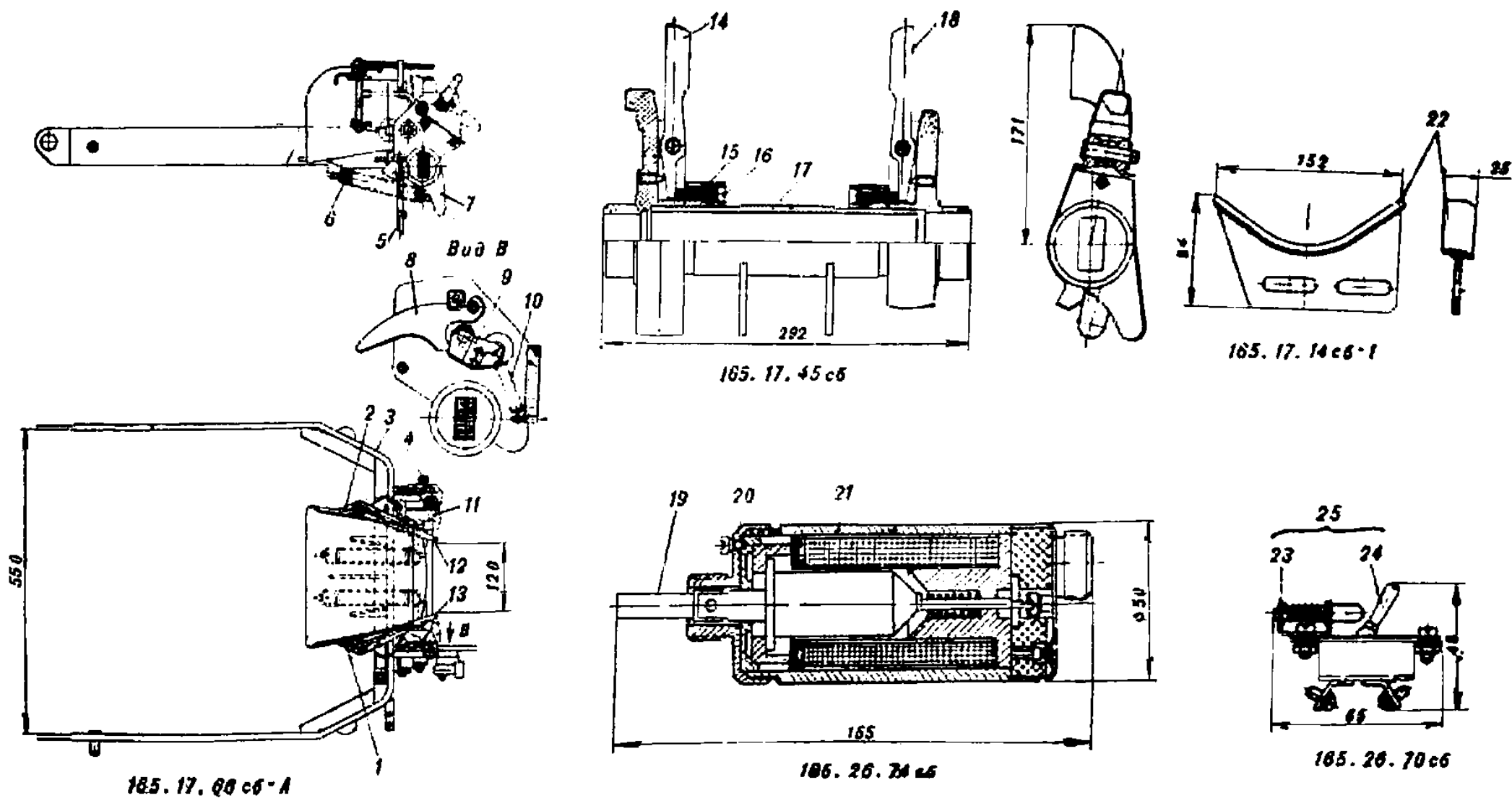
Рис. 40. Узлы механизма выброса гильз
