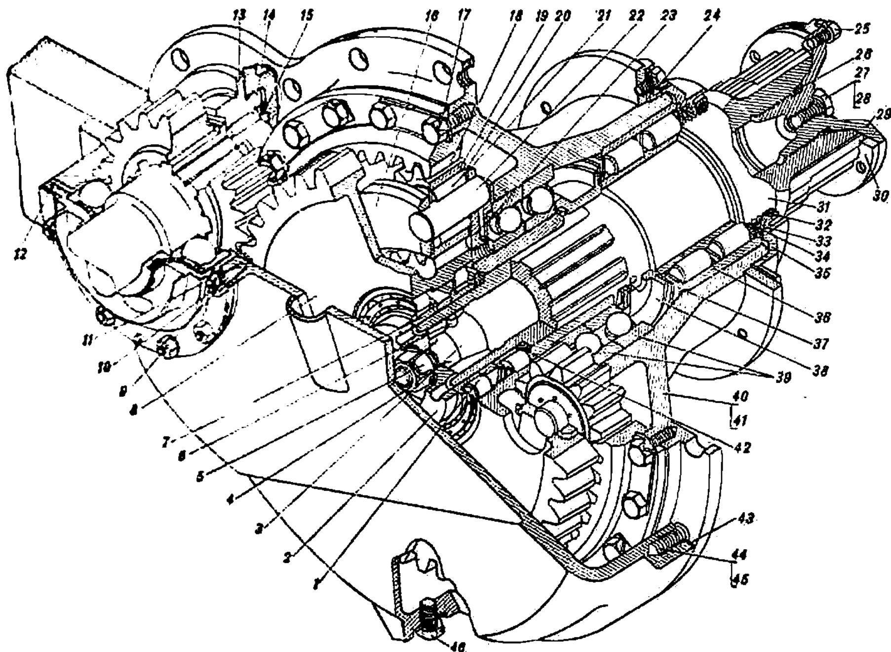
Рис. 37. Планетарная бортовая передача (левая 155.16.16сб-Б и правая 155.16.17сб-Б)
