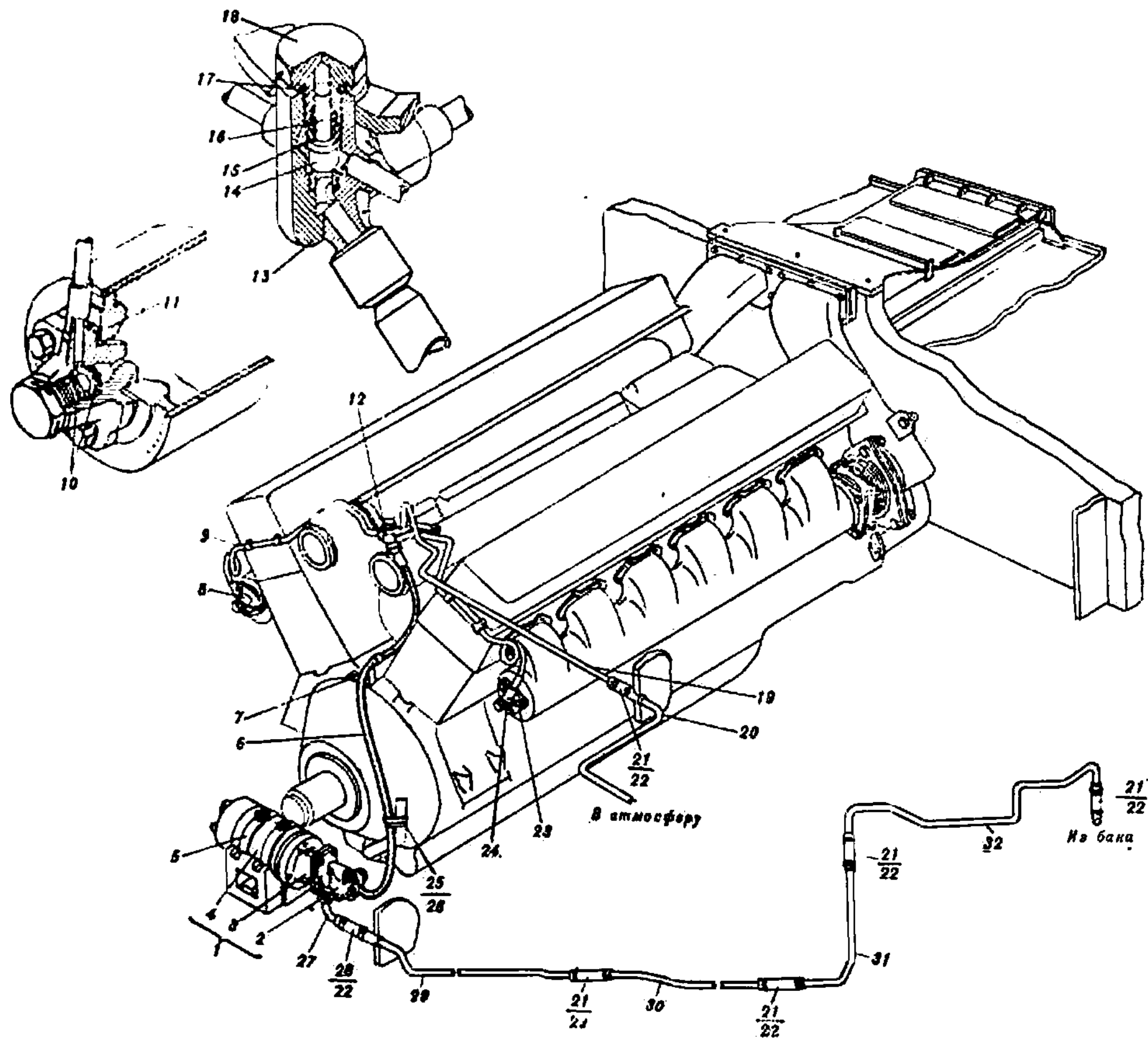
Рис. 152. Система термической дымовой аппаратуры (165.58сб-2)
