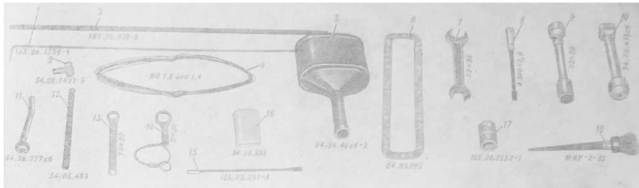
Рис. 80. Инструмент и принадлежности экипажа
