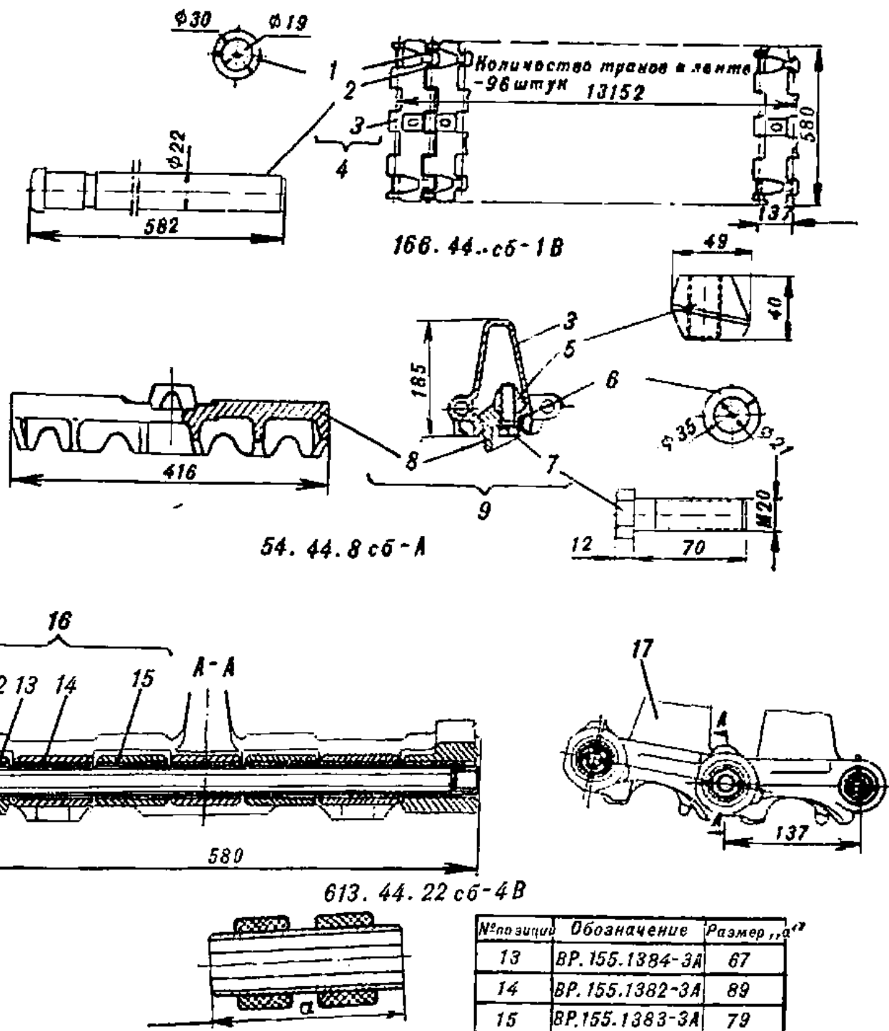
Рис. 147. Гусеница
