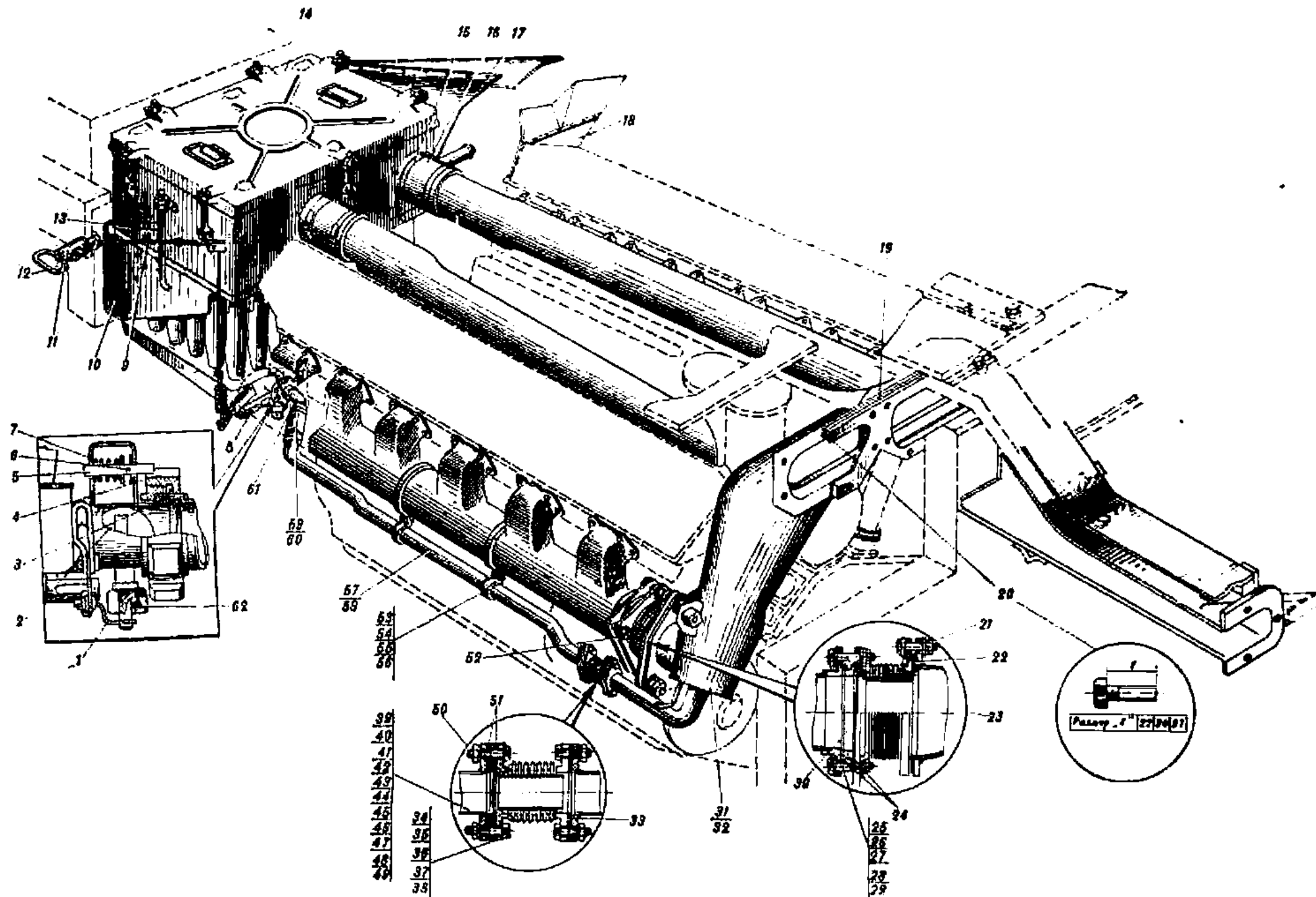
Рис. 9. Установка воздухоочистителя (165.04сб-1А) и выпускного трубопровода (155.06сб-А)
