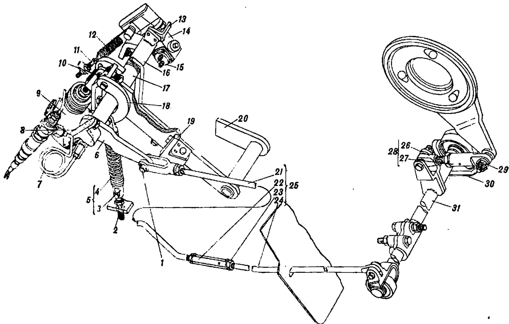
Рис. 50. Привод управления главным фрикционом (165.21с6-4)
