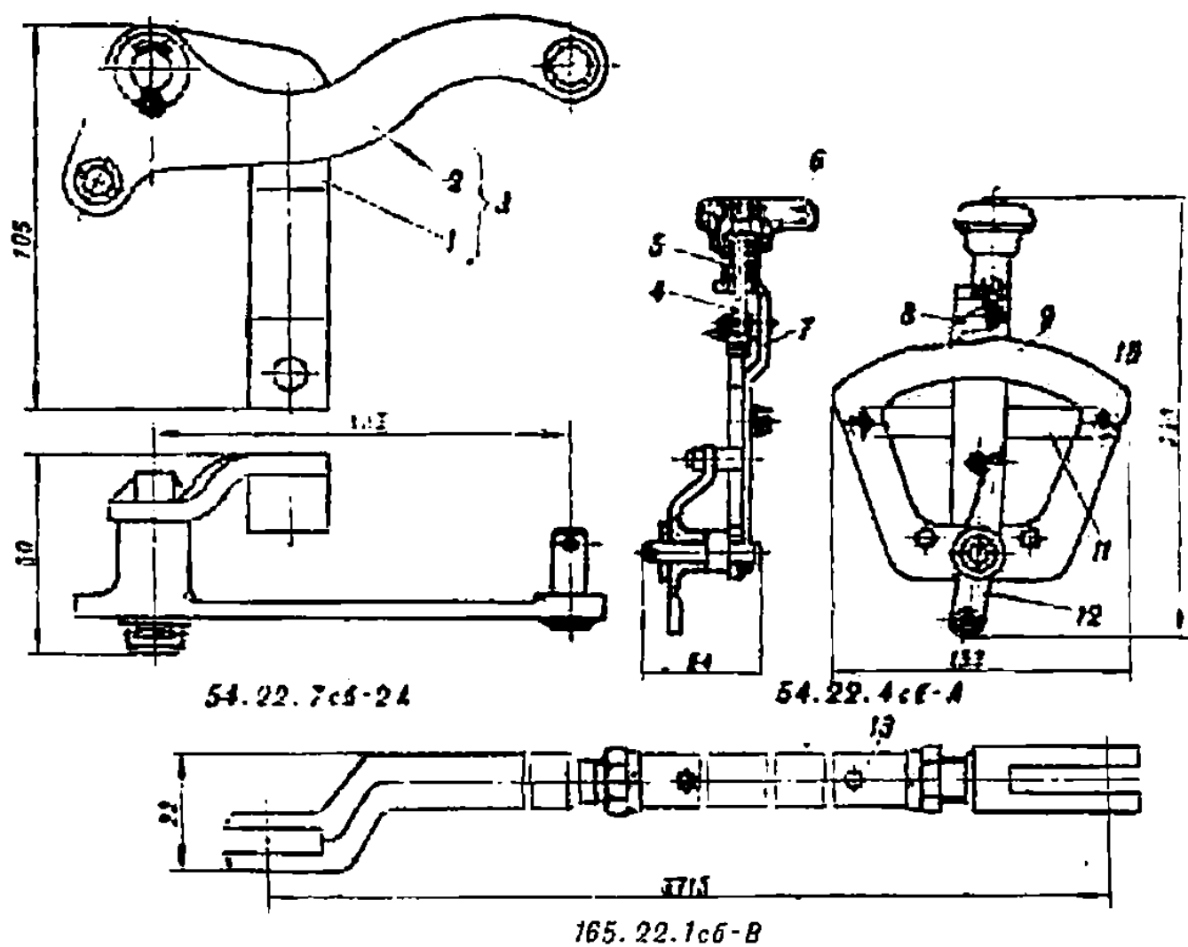
Рис. 56. Узлы и детали привода к топливному насосу
