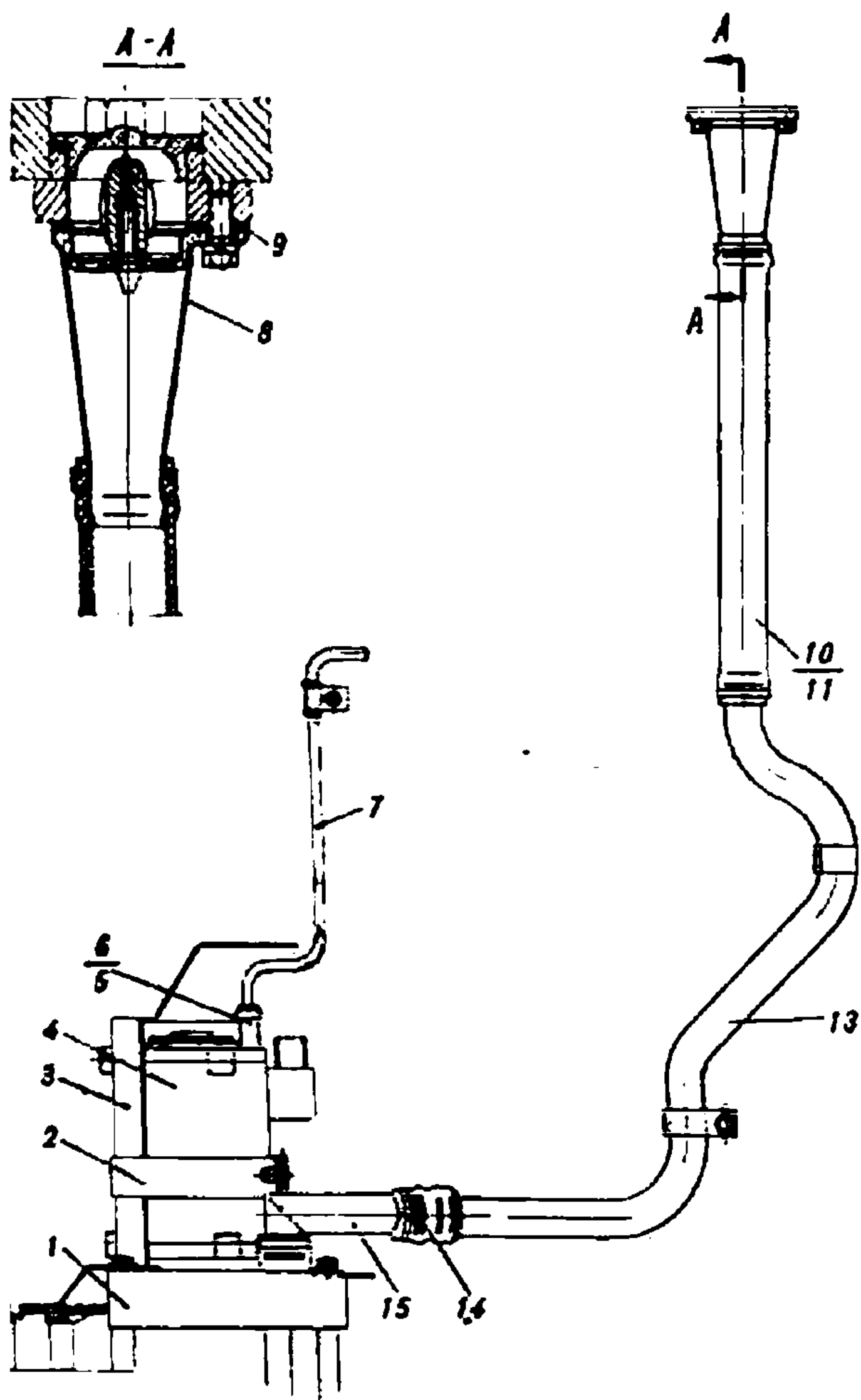
Рис. 158. Установка насоса (165.83.1сб-3Б)
