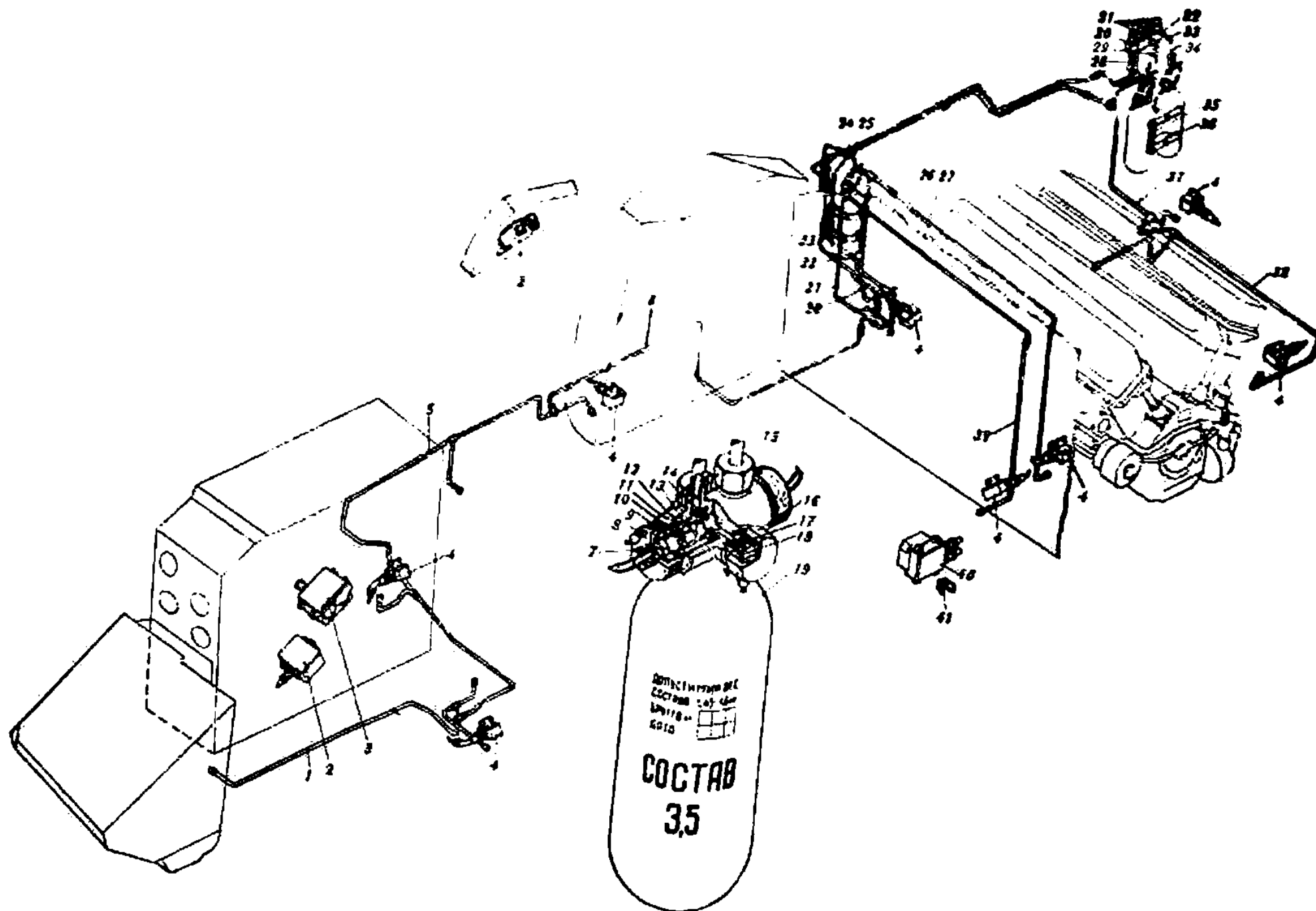
Рис. 153. Противопожарное оборудование (165.59сб-1)
