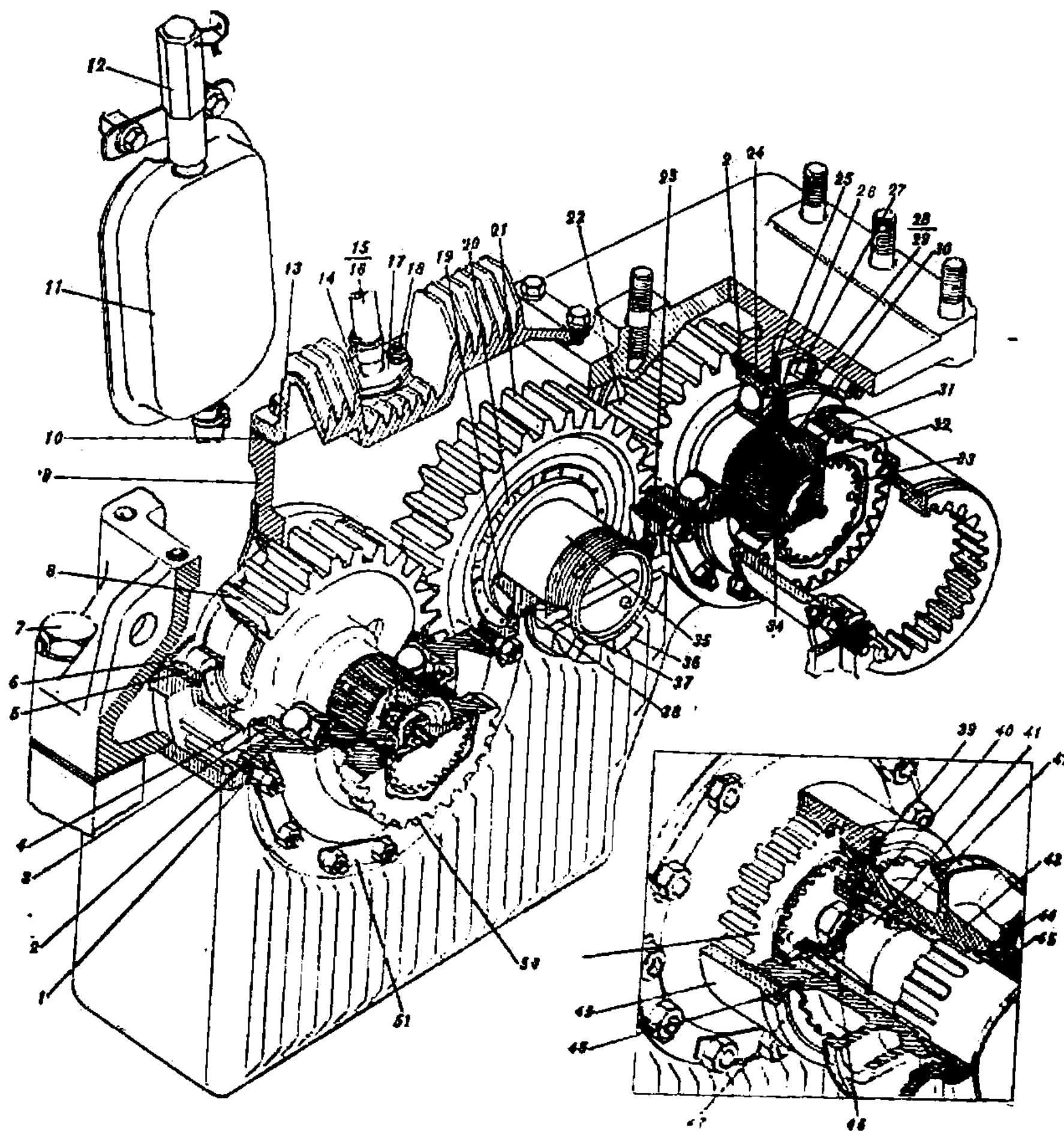
Рис. 140. Гитара (54.40сб-4А)
