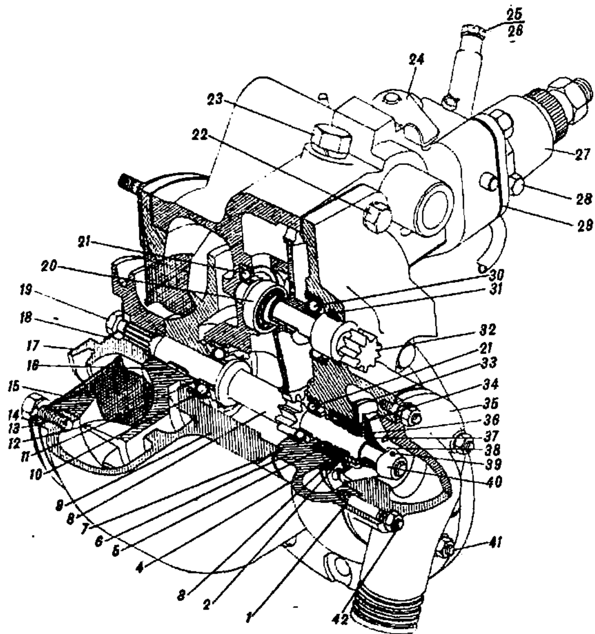
Рис. 144. Редуктор подогревателя (166.42.1сб-А).
