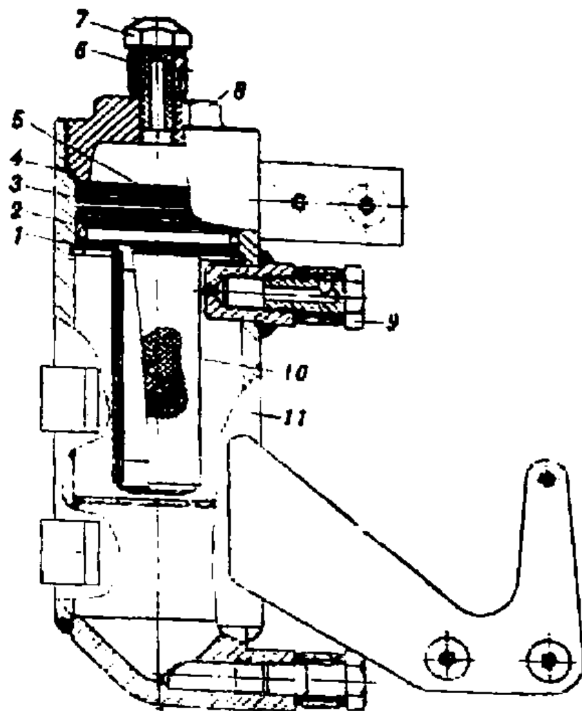
Рис. 135. Влагомаслоотделитель (155.38.10сб-2В)
