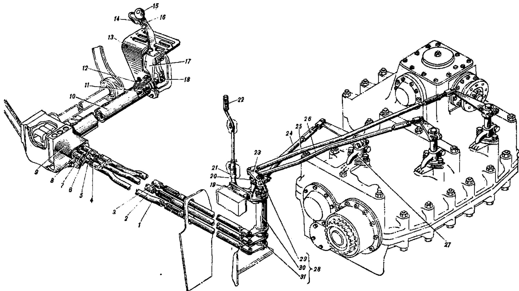
Рис. 45. Привод управления коробкой передач (165.19сб-3)
