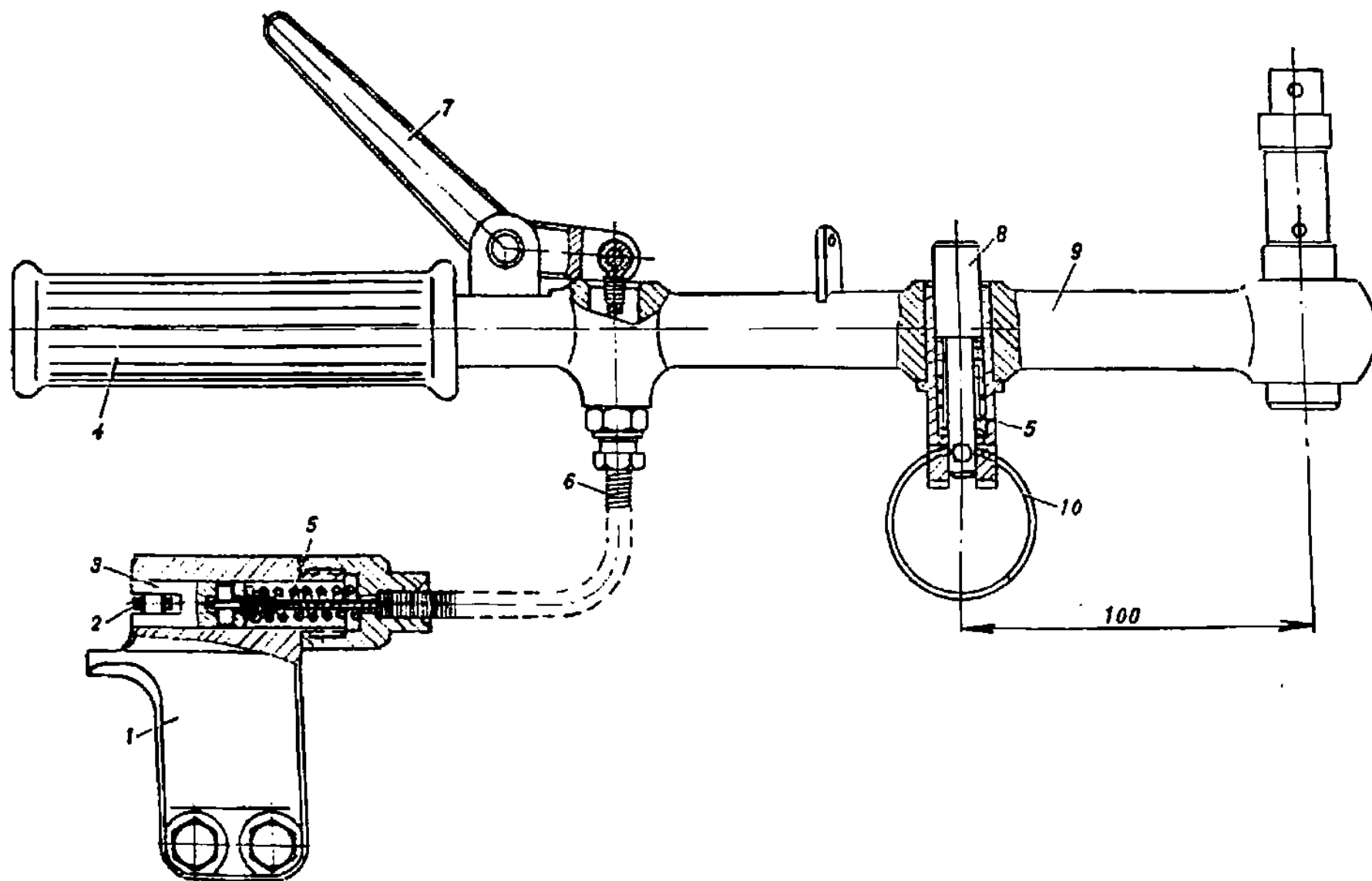
Рис. 115. Рукоятка (155.32.5с6-1А)
