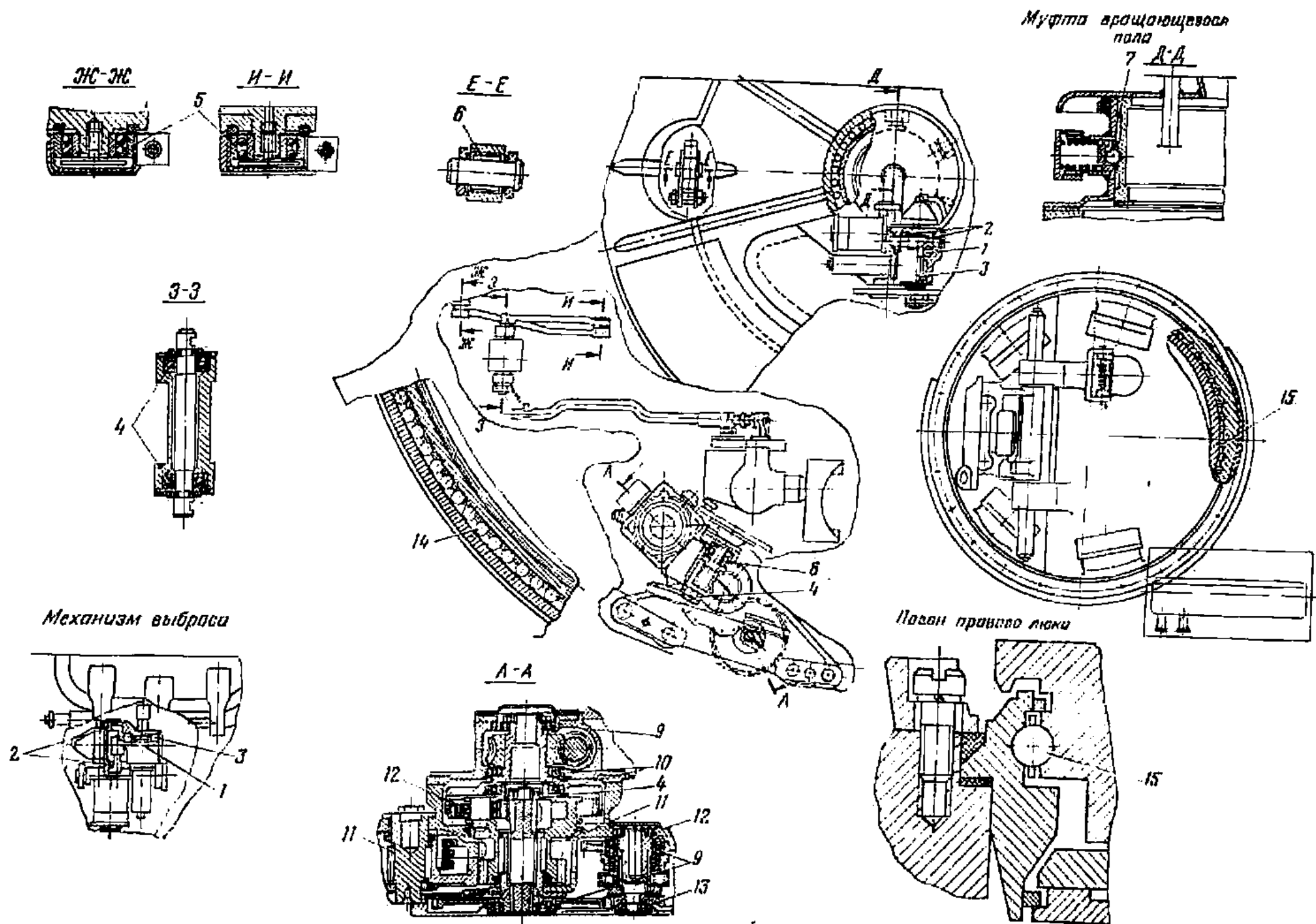
Рис. 164. Подшипники, шары и ролики в механизмах башни
