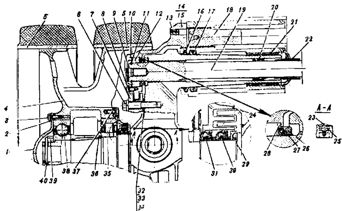
Рис. 32. Подвеска с передним (задним) опорным катком (165.12.4сб-А)
