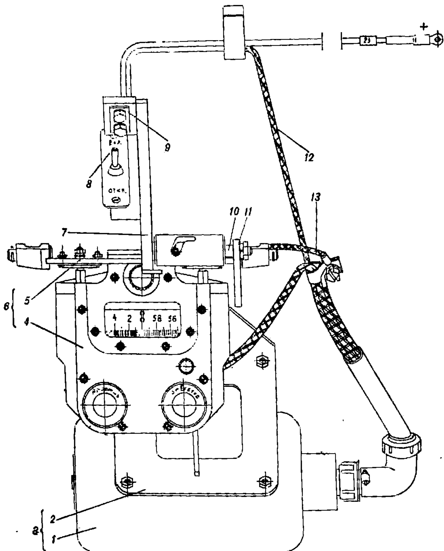
Рис. 155. Установка гирополукомпаса ГПК-59 и ПАГ-1Ф (54.75сб-2)
