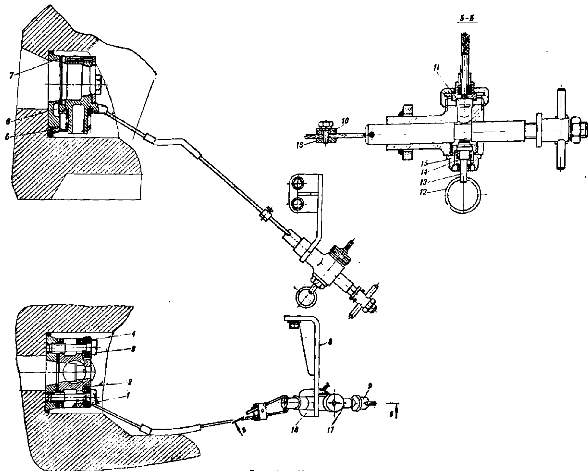
Рис. 108. Установка механизма защиты ТИИС (166.31.26с6-2)
