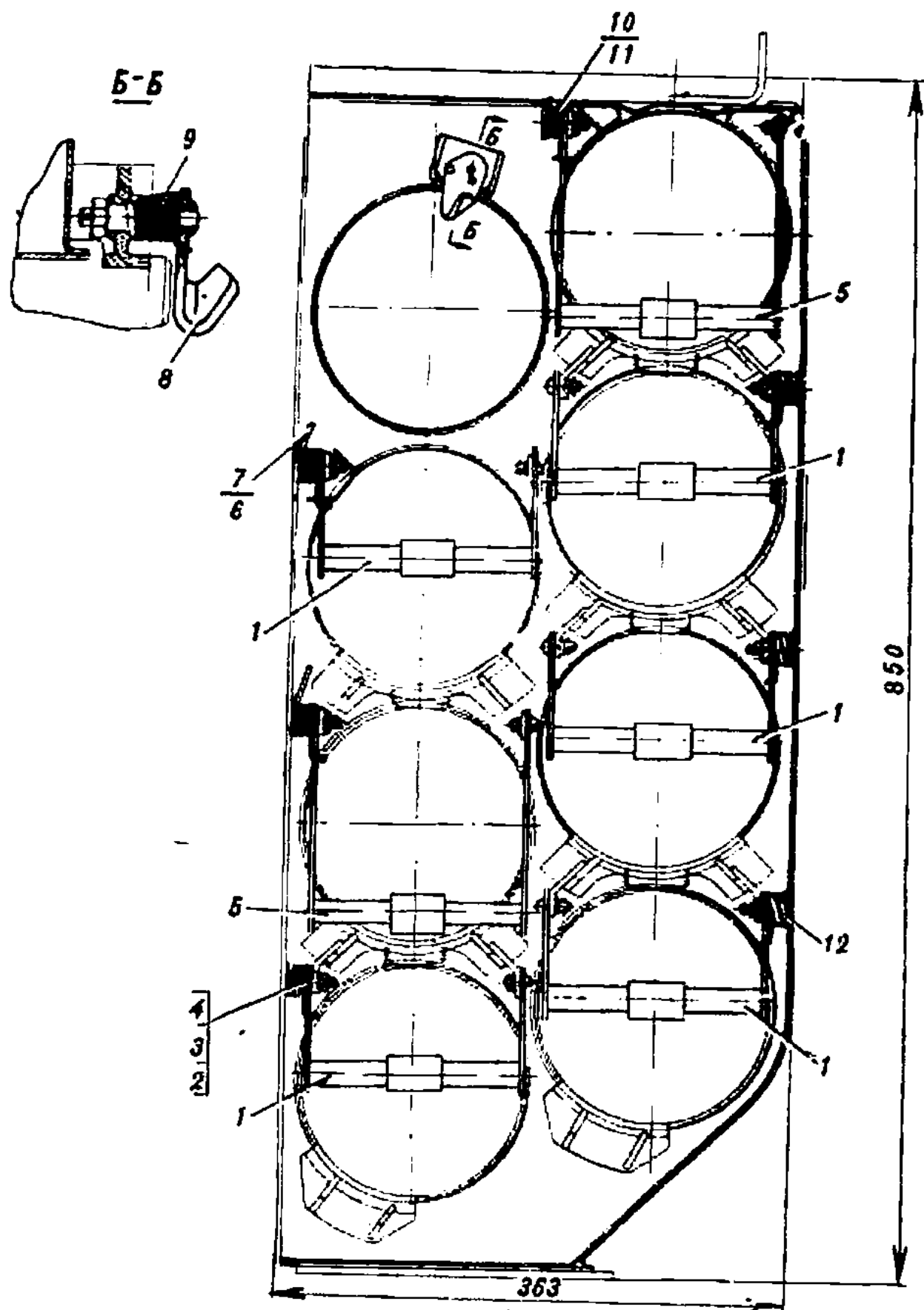
Рис. 71. Установка опор и защелок на баке-стеллаже правом (166.27.43сб-А) и левом (166.27.44сб-А)
