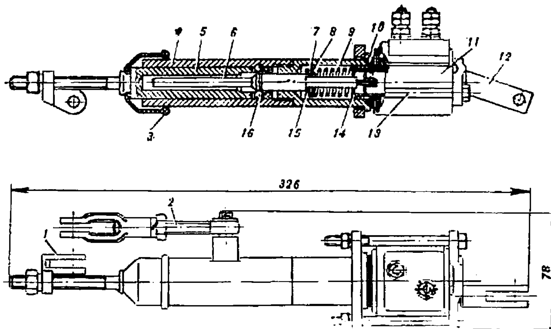
Рис. 55. Механизм остановки двигателя (155.22.15с6-1)
