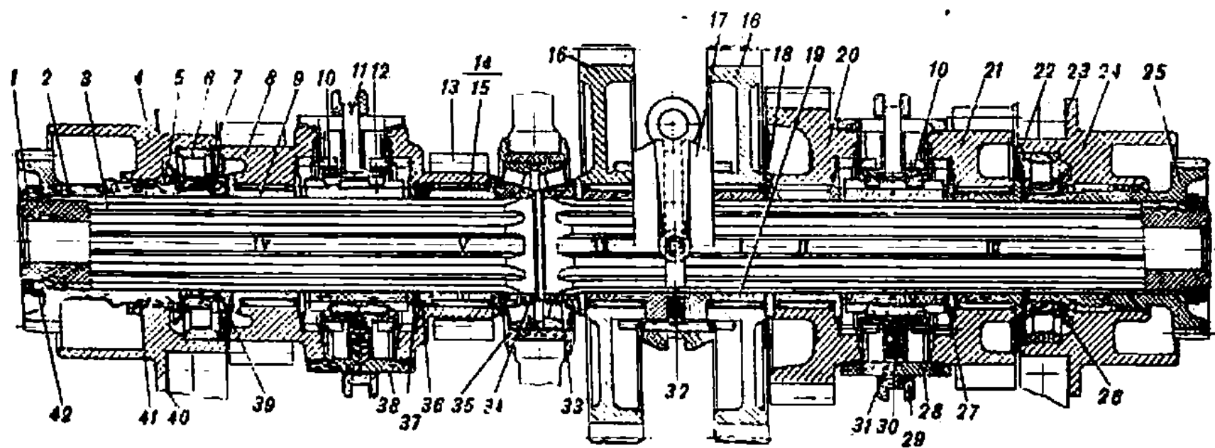
Рис. 23. Вал главный
