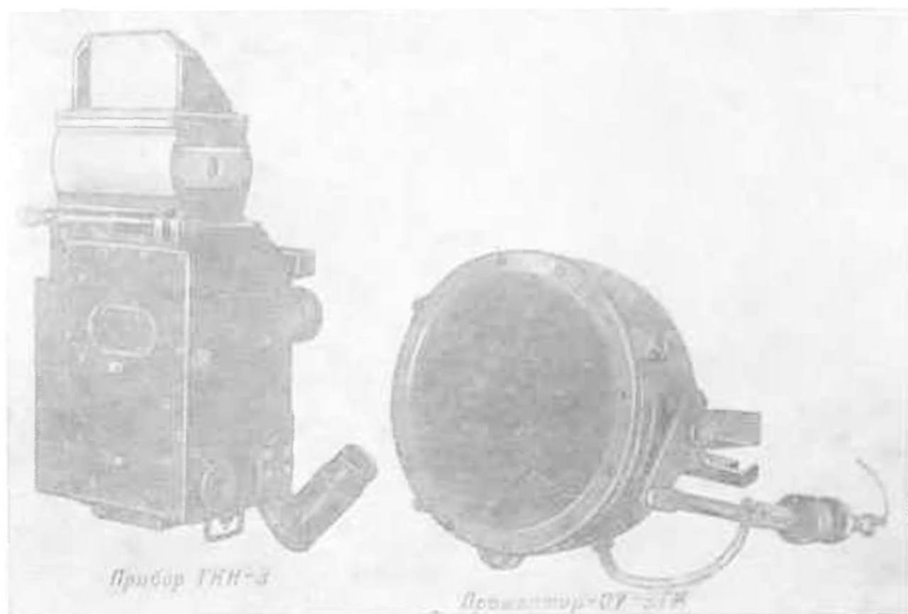
Рис. 129. Комплект прибора командира ТКН-3 (166.36.007). с ЗИП
