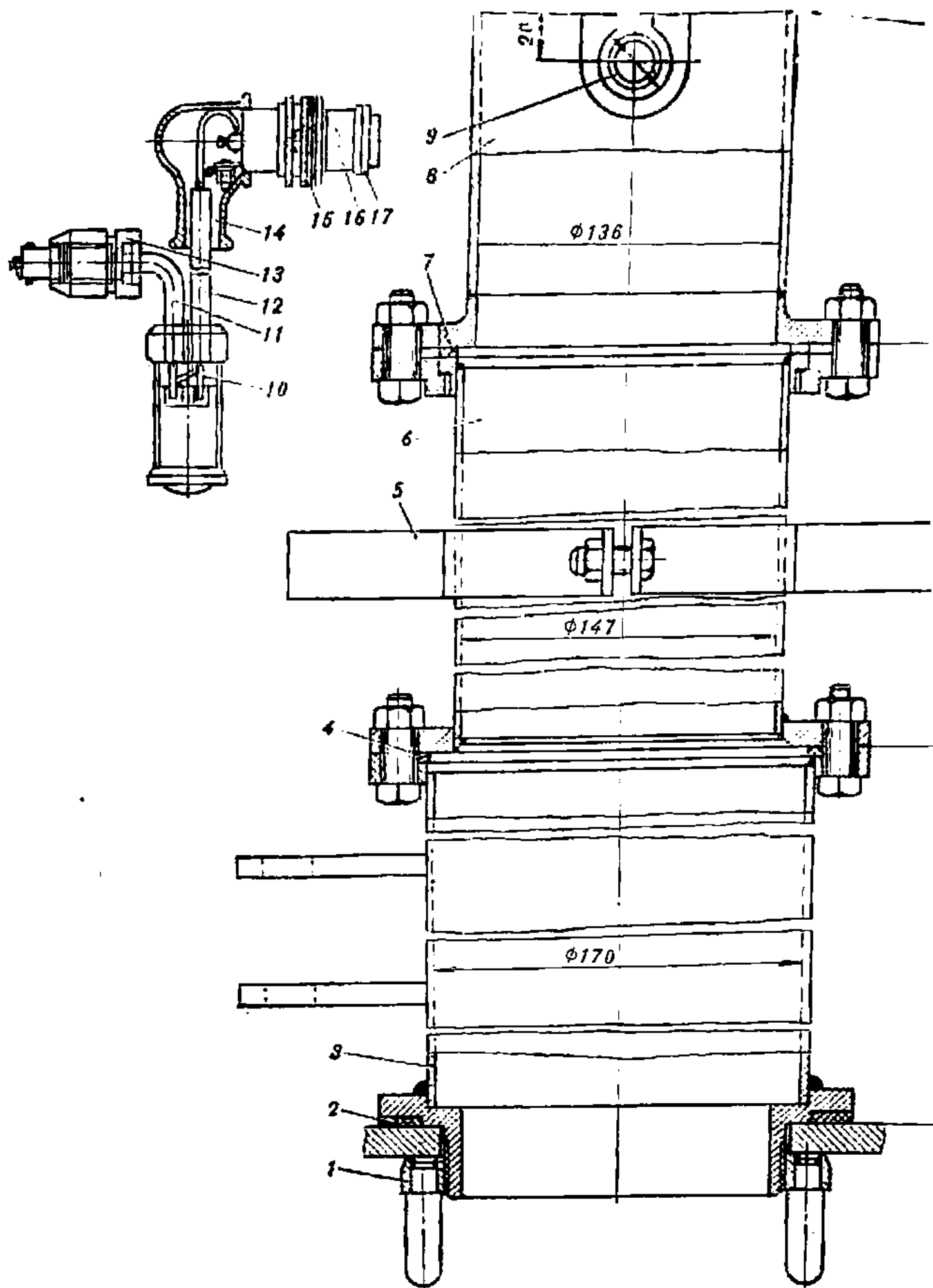
Рис. 156. Труба воздухопитающая (54.83.9сб-1А)
