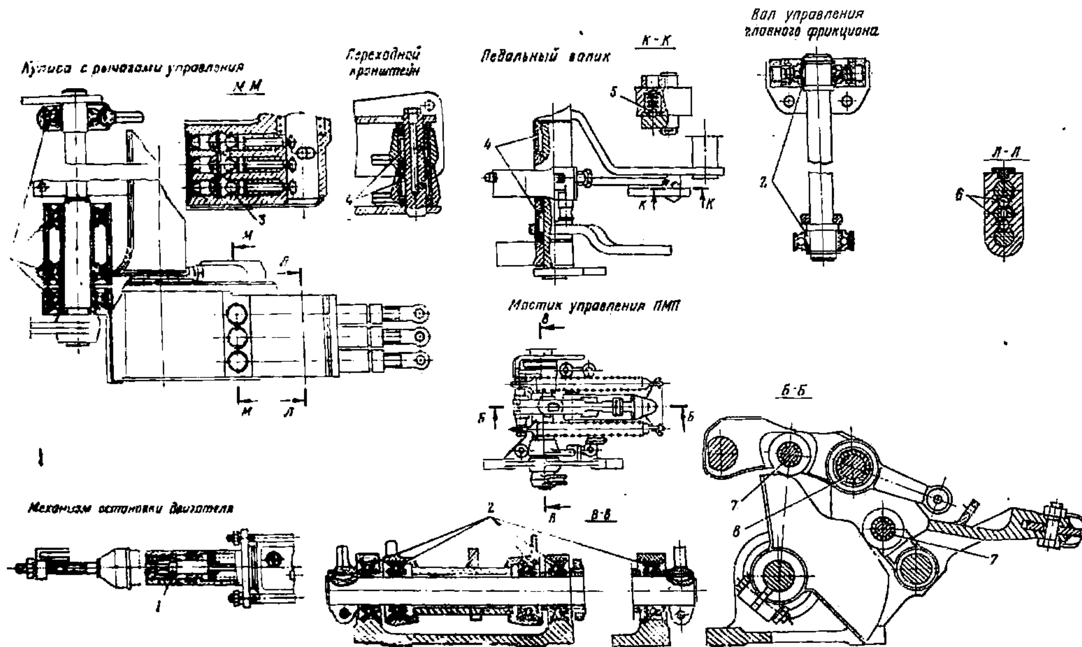
Рис. 163. Подшипники, шарики и ролики механизмов управления
