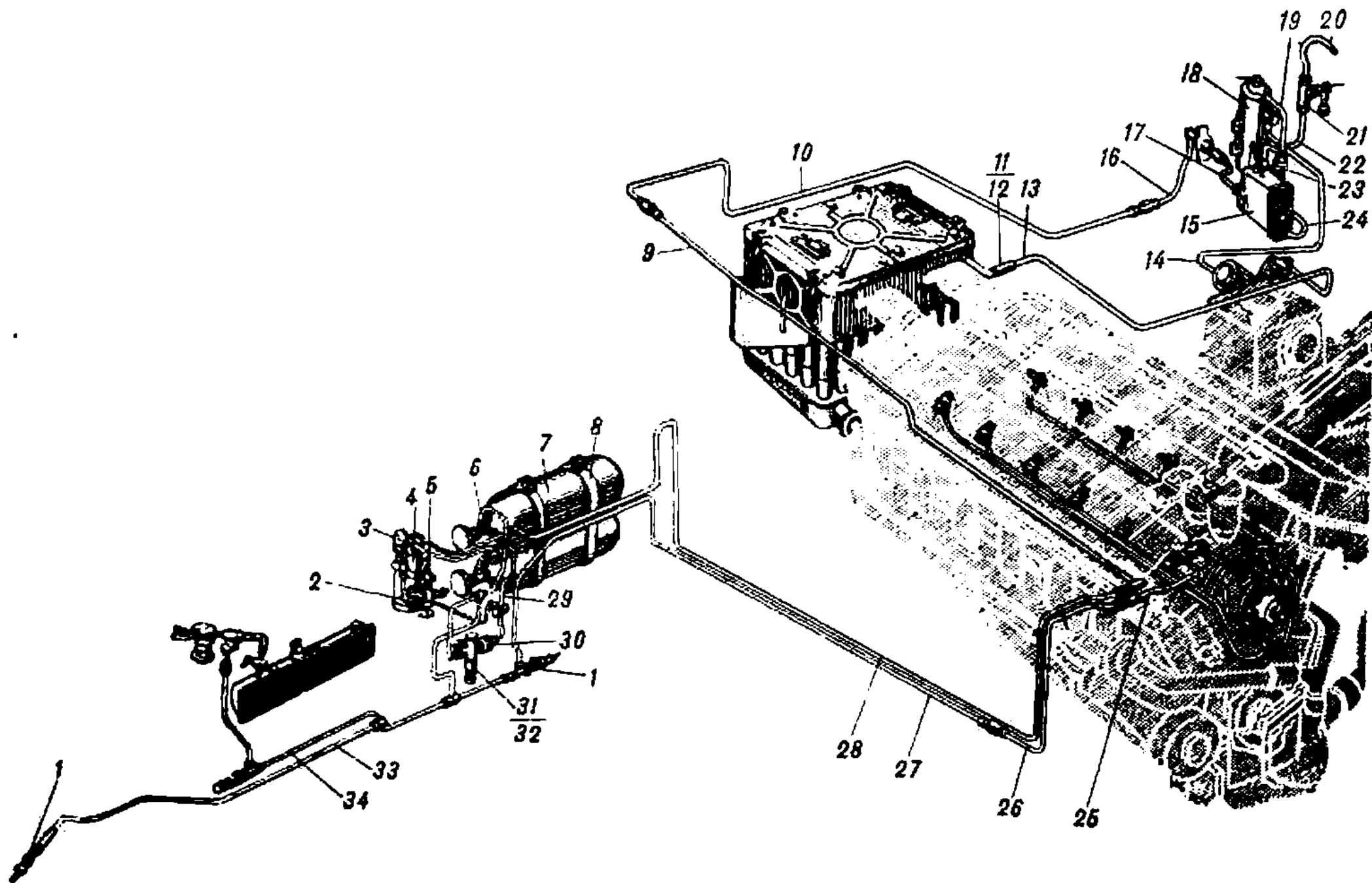
Рис. 133. Воздушная система (166.38сб-1)
