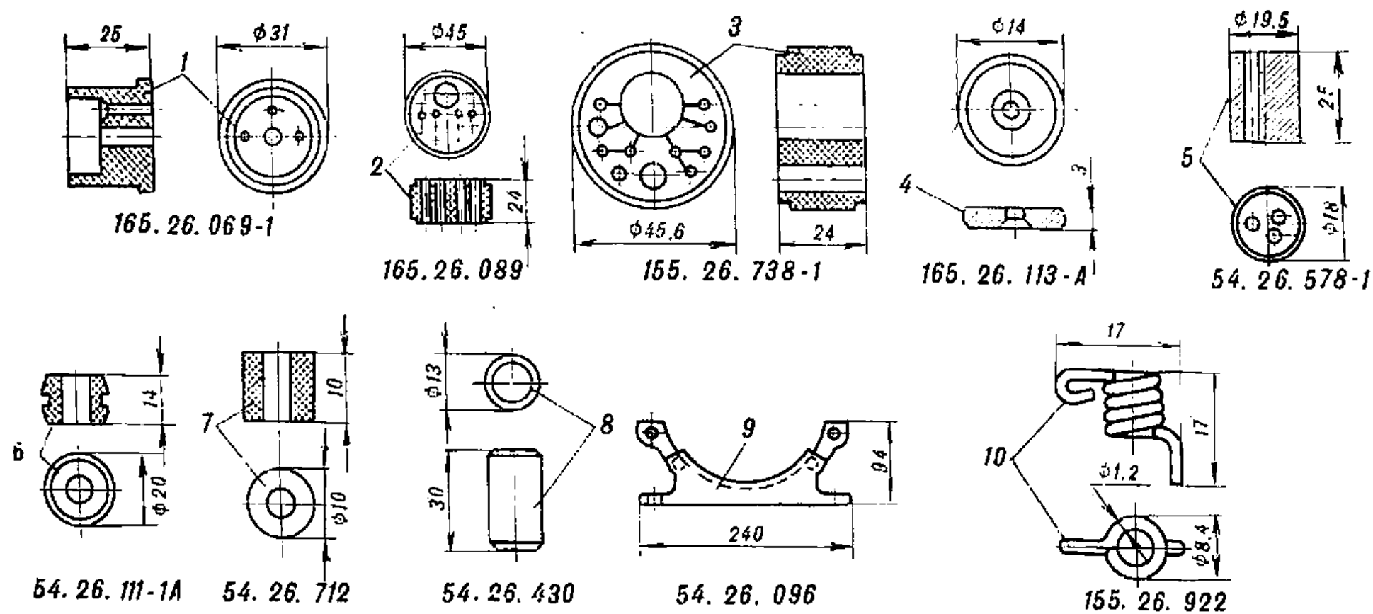
Рис. 66. Детали электрооборудования
