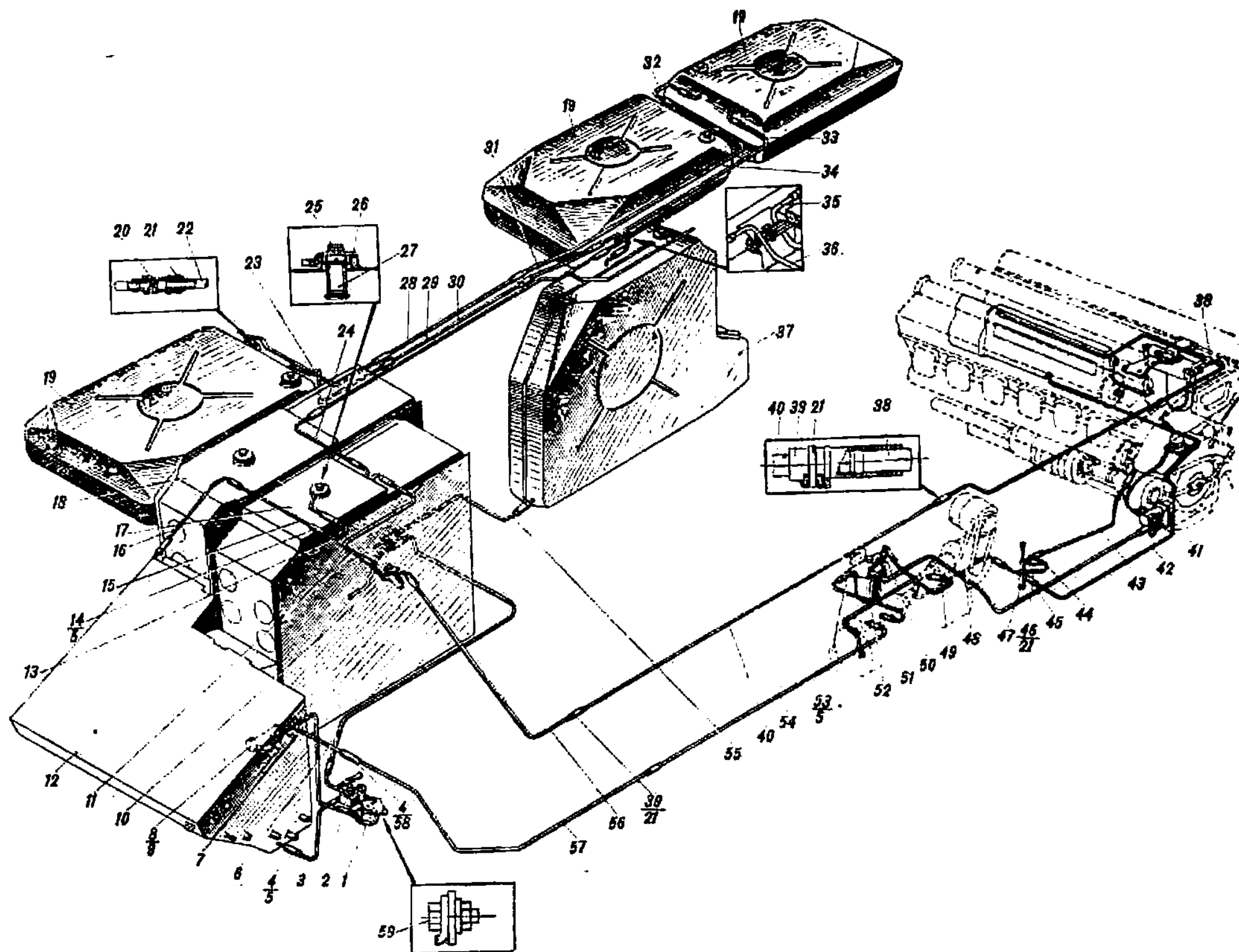
Рис. 11. Система питания топливом (165.05сб-4)
