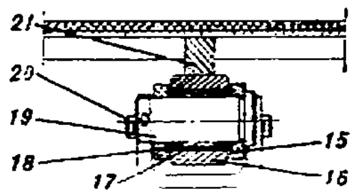
Рис. 88. Муфта (155.29.525с6-2)
