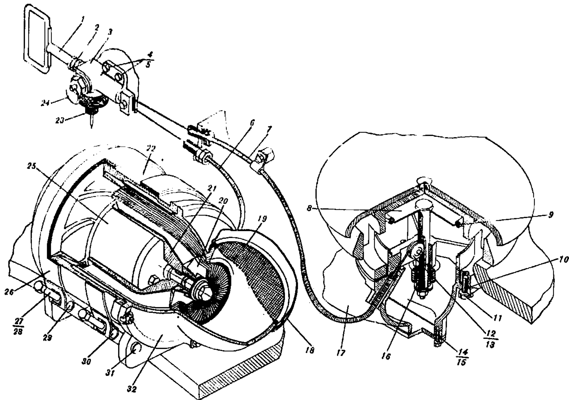
Рис. 100. Установка магнетателя (165.30.15сб-1)
