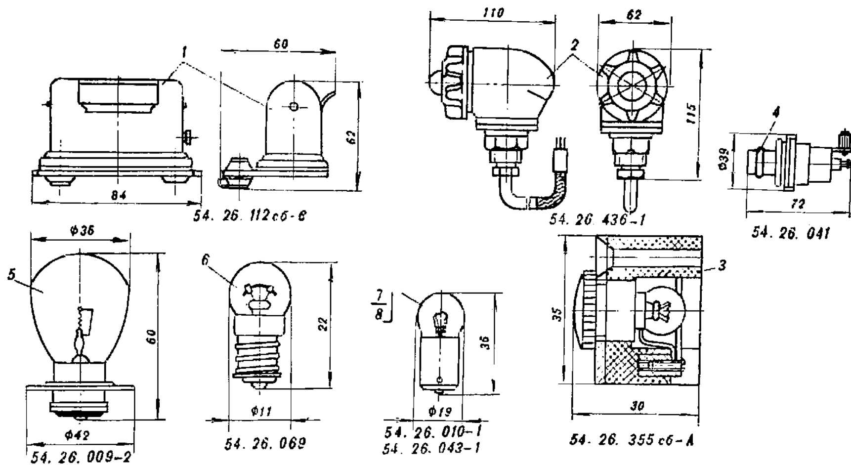
Рис. 63. Светильники
