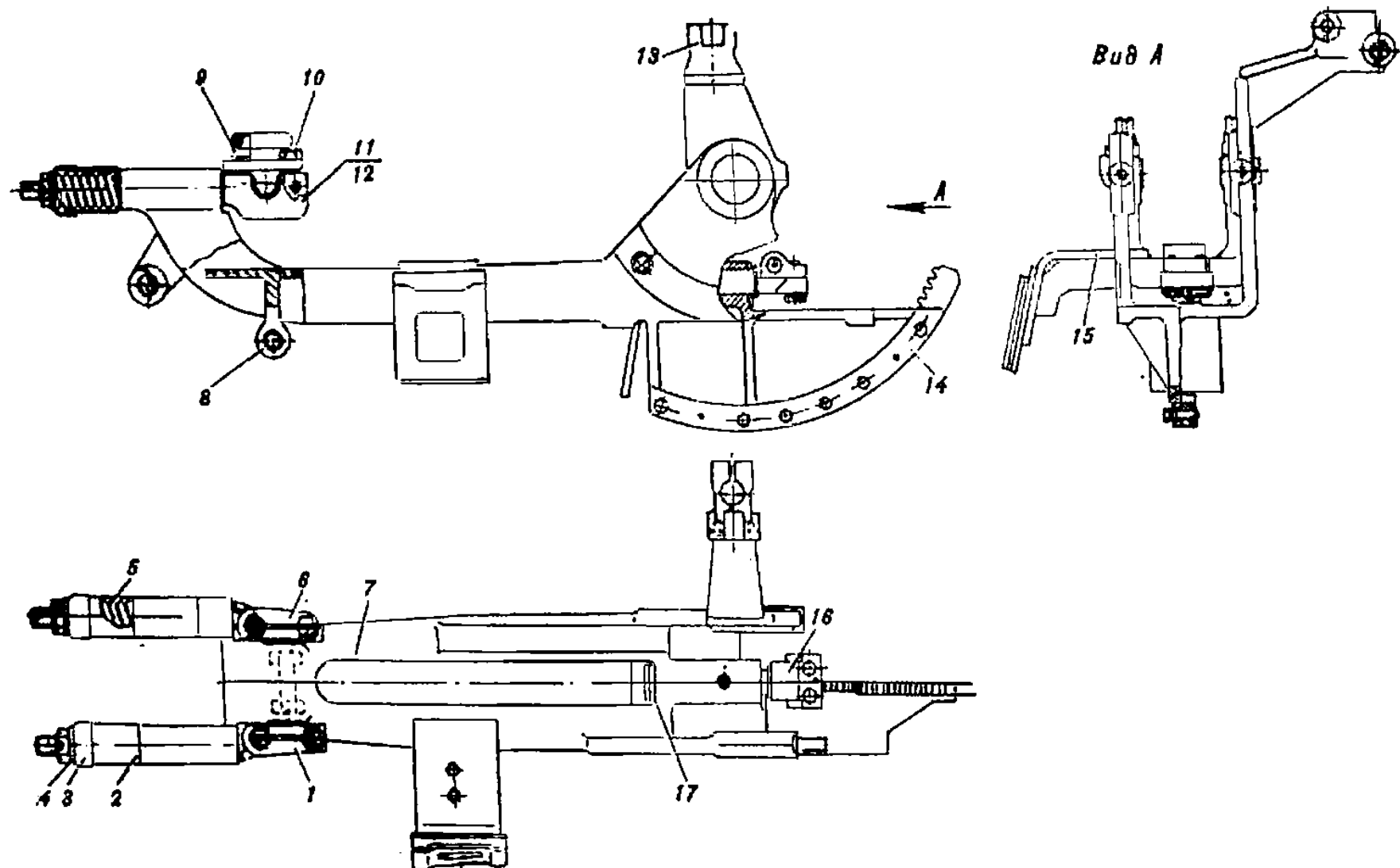
Рис. 113. Люлька (155.32.2сб)
