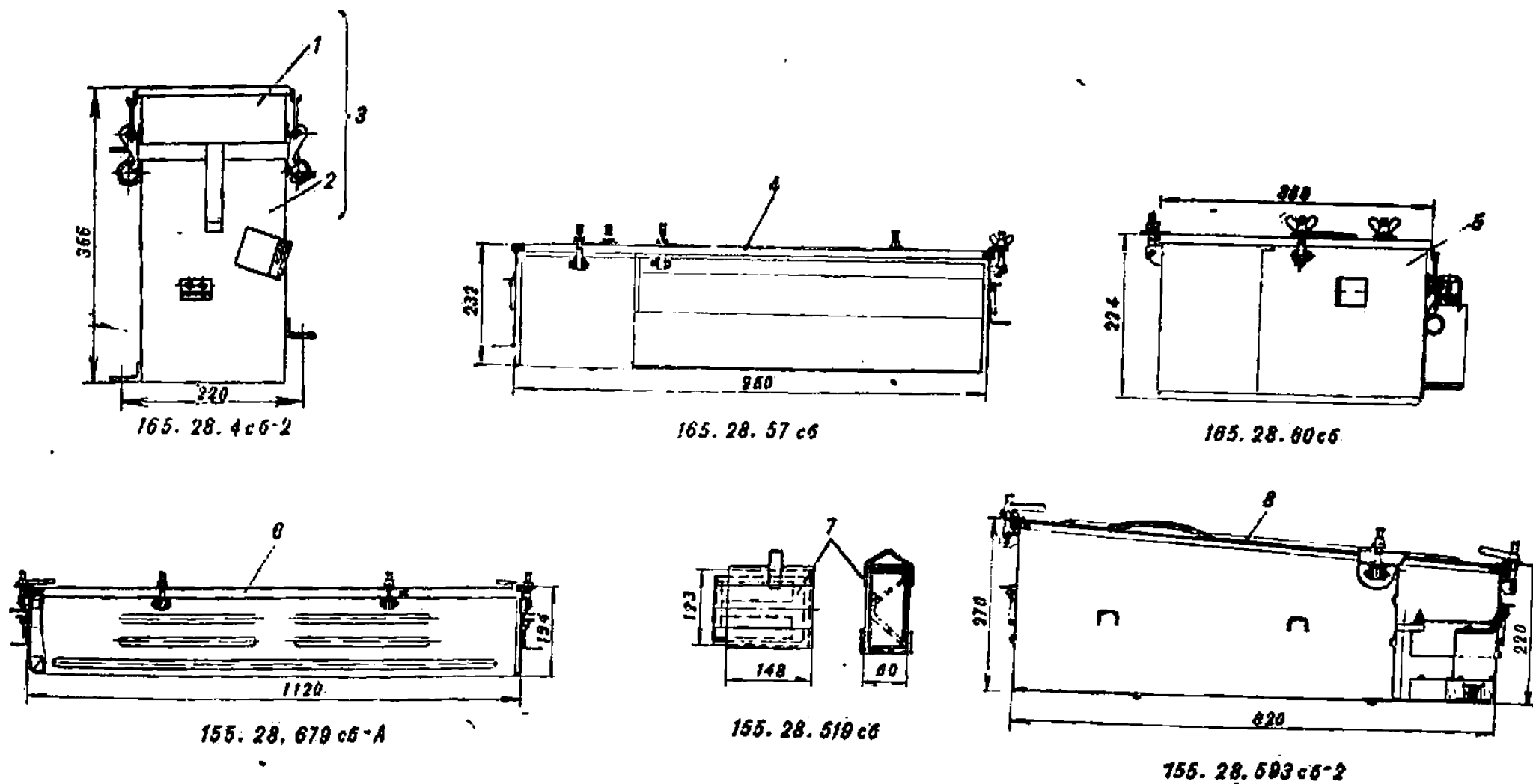
Рис. 74. Ящики и коробка для укладки ЗИП
