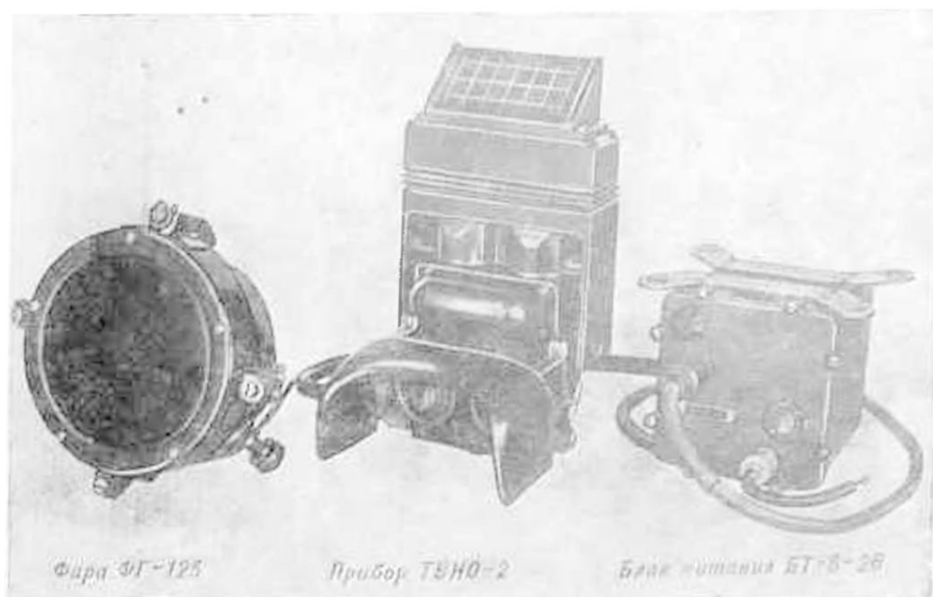
Рис. 128. Комплект ночного прибора механика ТВНО-2 . (54.36.334-А) с ЗИП
