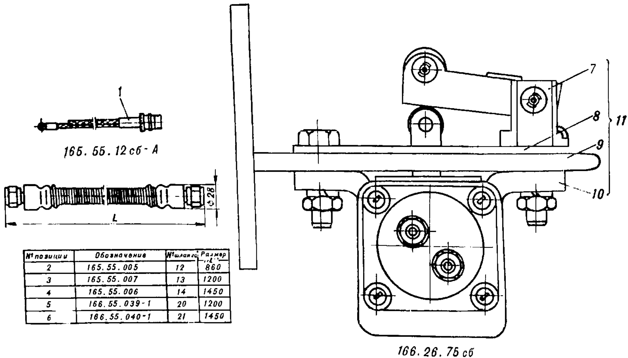
Рис. 150. Узлы и детали стабилизатора
