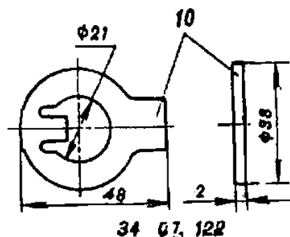
Рис. 141. Крепежные детали гитары
