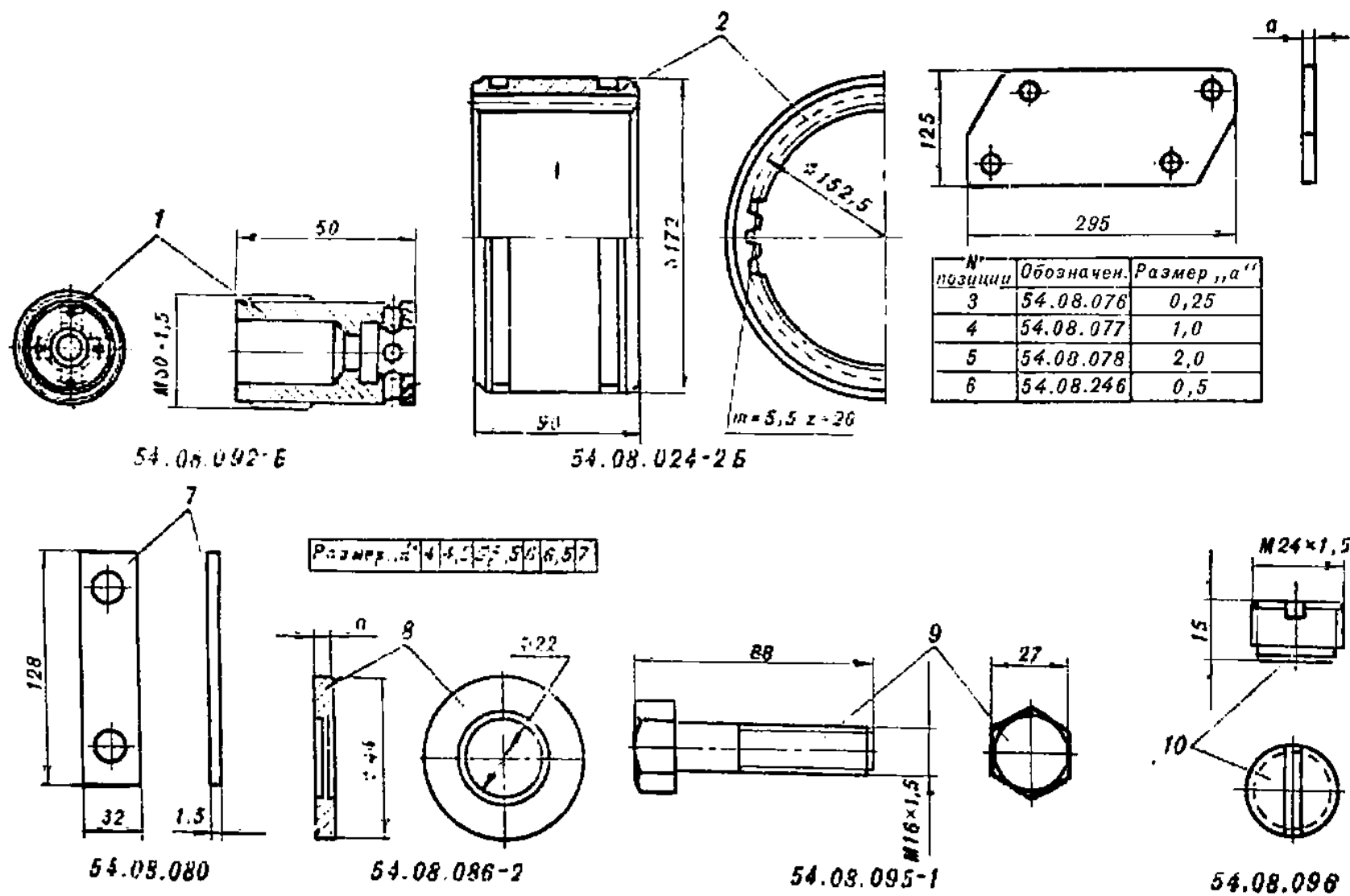
Рис. 25. Детали коробки передач
