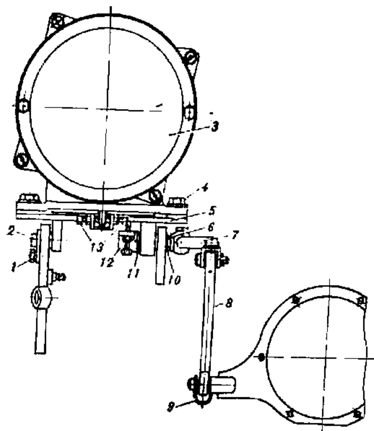
Рис. 103. Установка осветителя Л-2Г (165.31.13с6)
