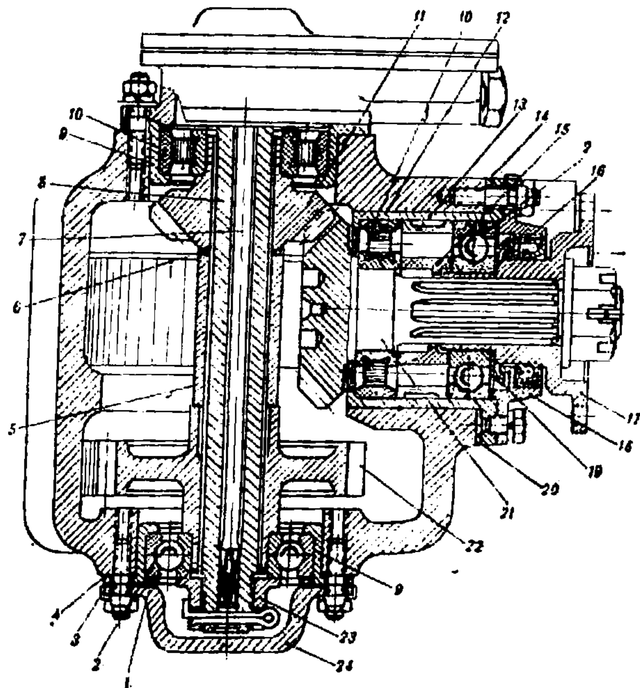
Рис. 24. Привод к вентилятору
