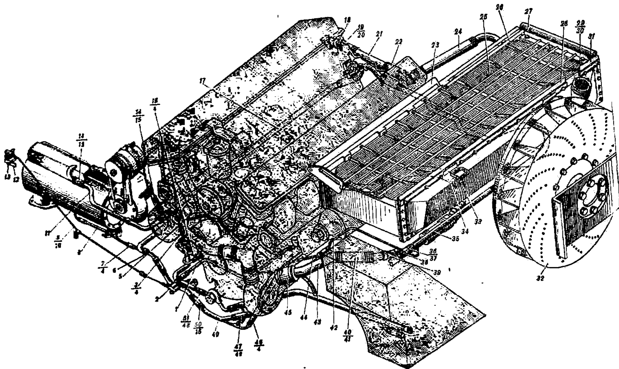
Рис. 2. Система охлаждения (165.02сб-3) и установка трассы подогрева (166.02.10сб)
