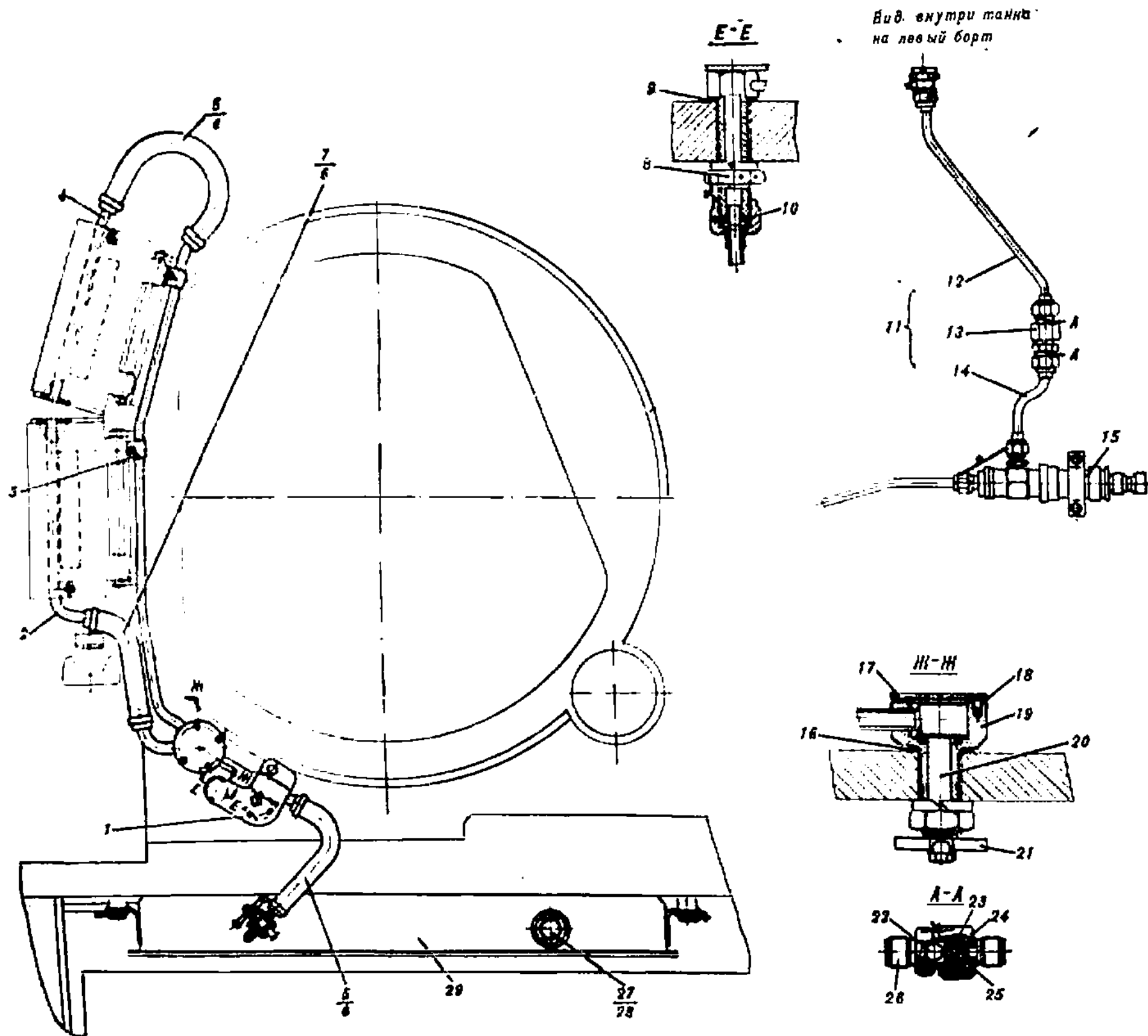
Рис. 127. Установка очистки смотровых приборов (166.36.1сб-А)
