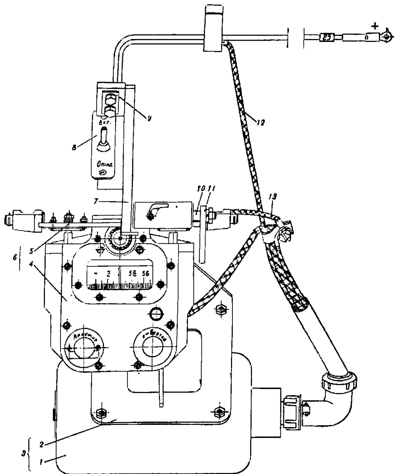
Рис. 185. Установка гиropolукомnаса ГПК-59 (54.75сб-2)
