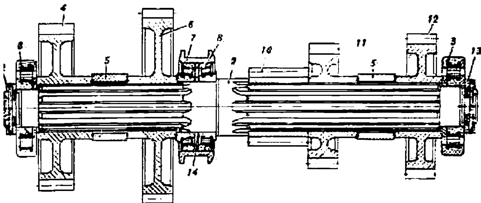
Рис. 21. Вал передаточный
