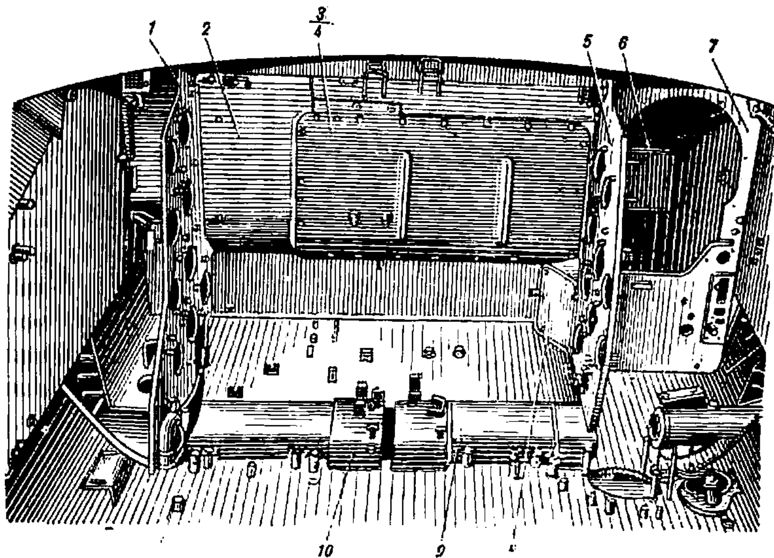
Рис. 85. Перегородка силового отделения
