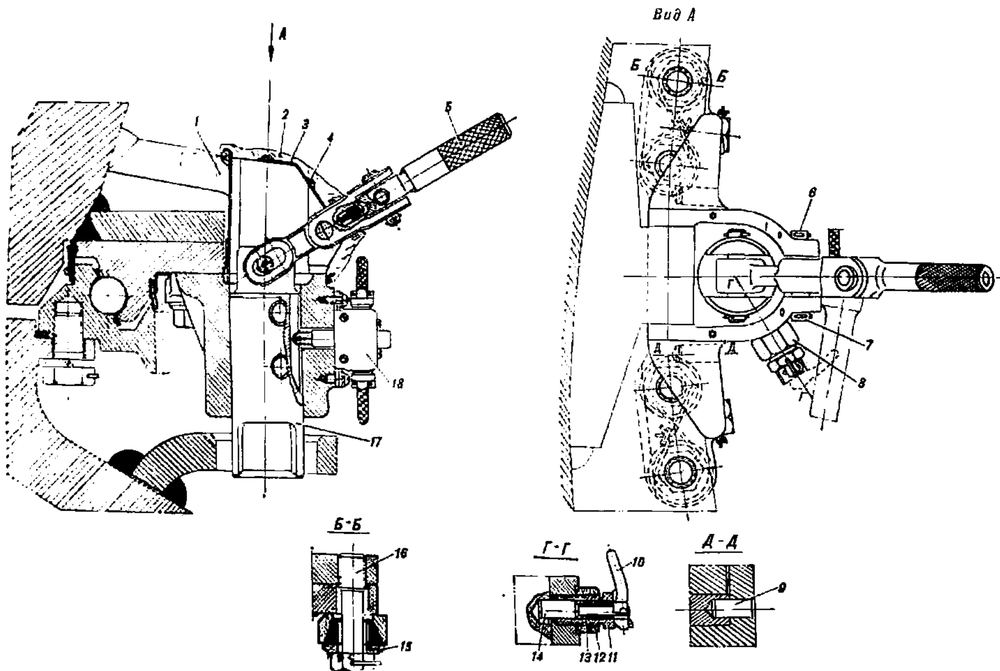
Рис. 96. Стопор башни (166.30.13сб).
