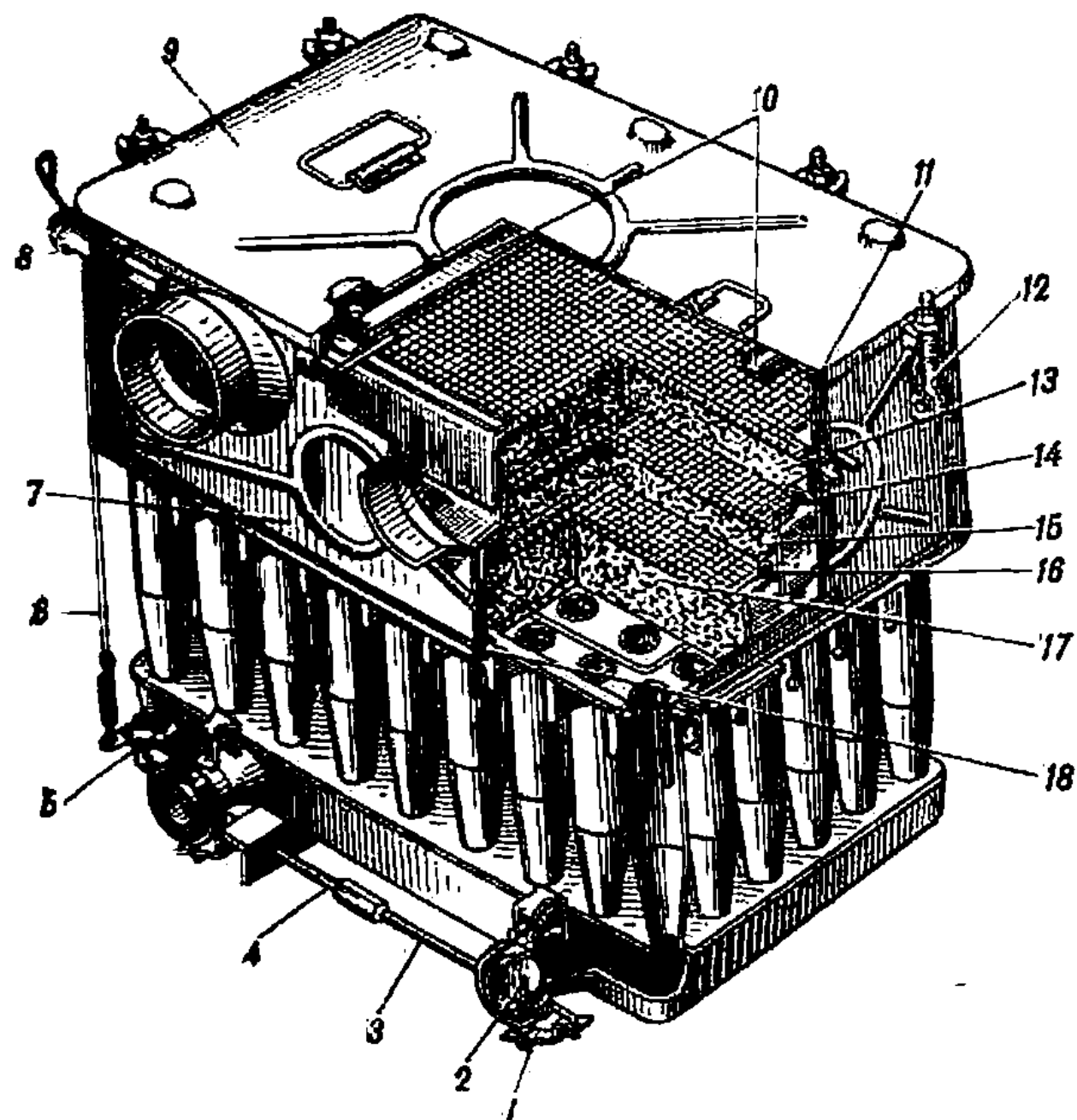
Рис. 10. Воздухоочиститель (54.04.35сб-5)
