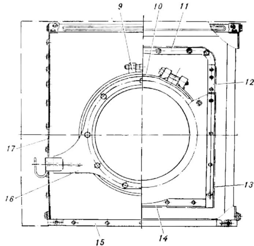
Рис. 105. Установка чехлов (166.31.2сб-1)
