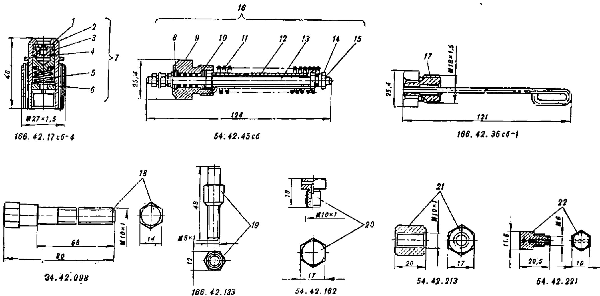
Рис. 146. Узлы и детали подогревателя
