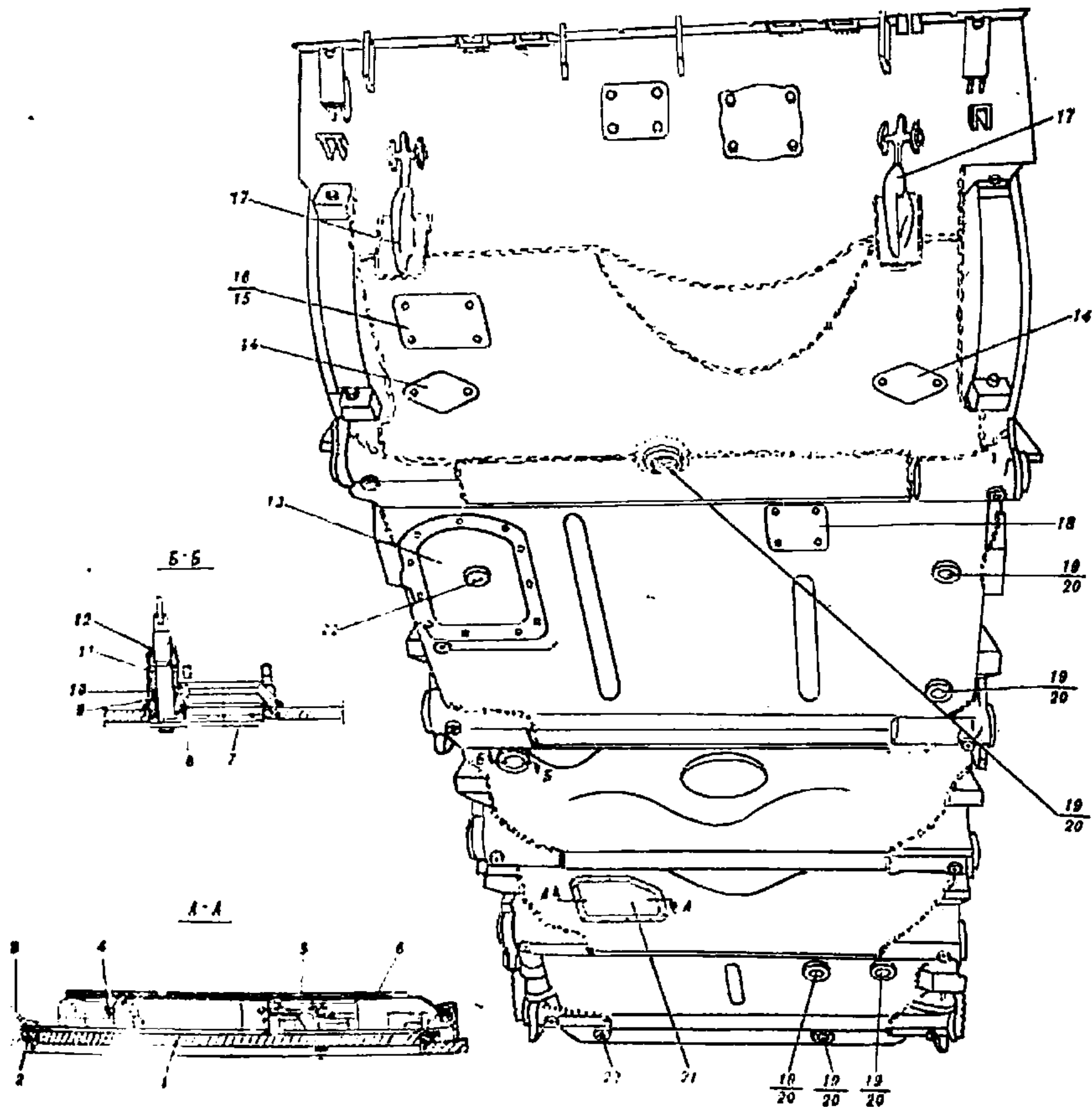
Рис. 84. Днище танка
