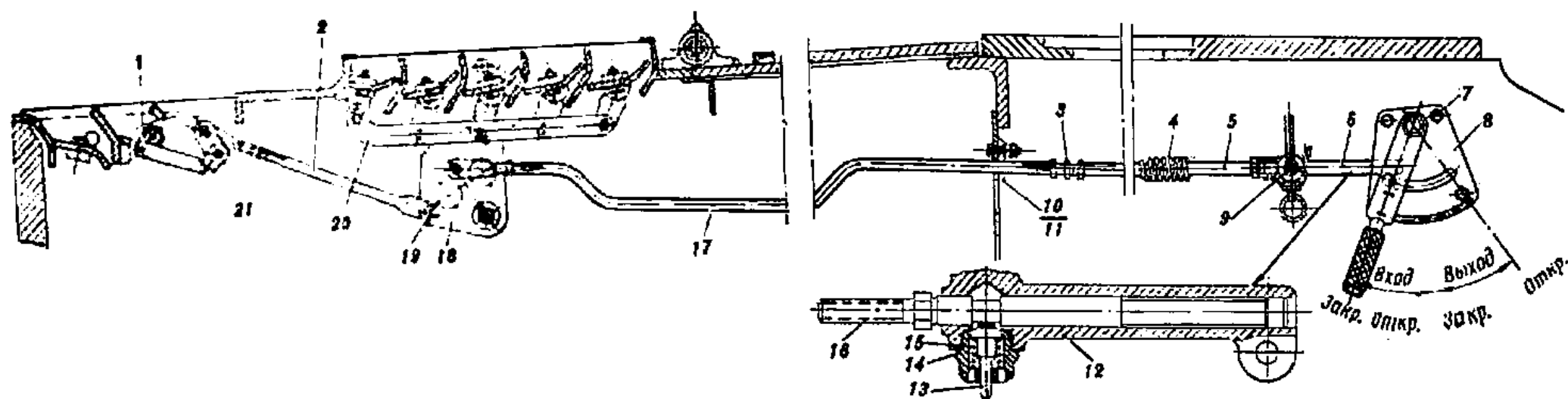
Рис. 91. Механизм привода жалюзи (155.29.457с6-2)
