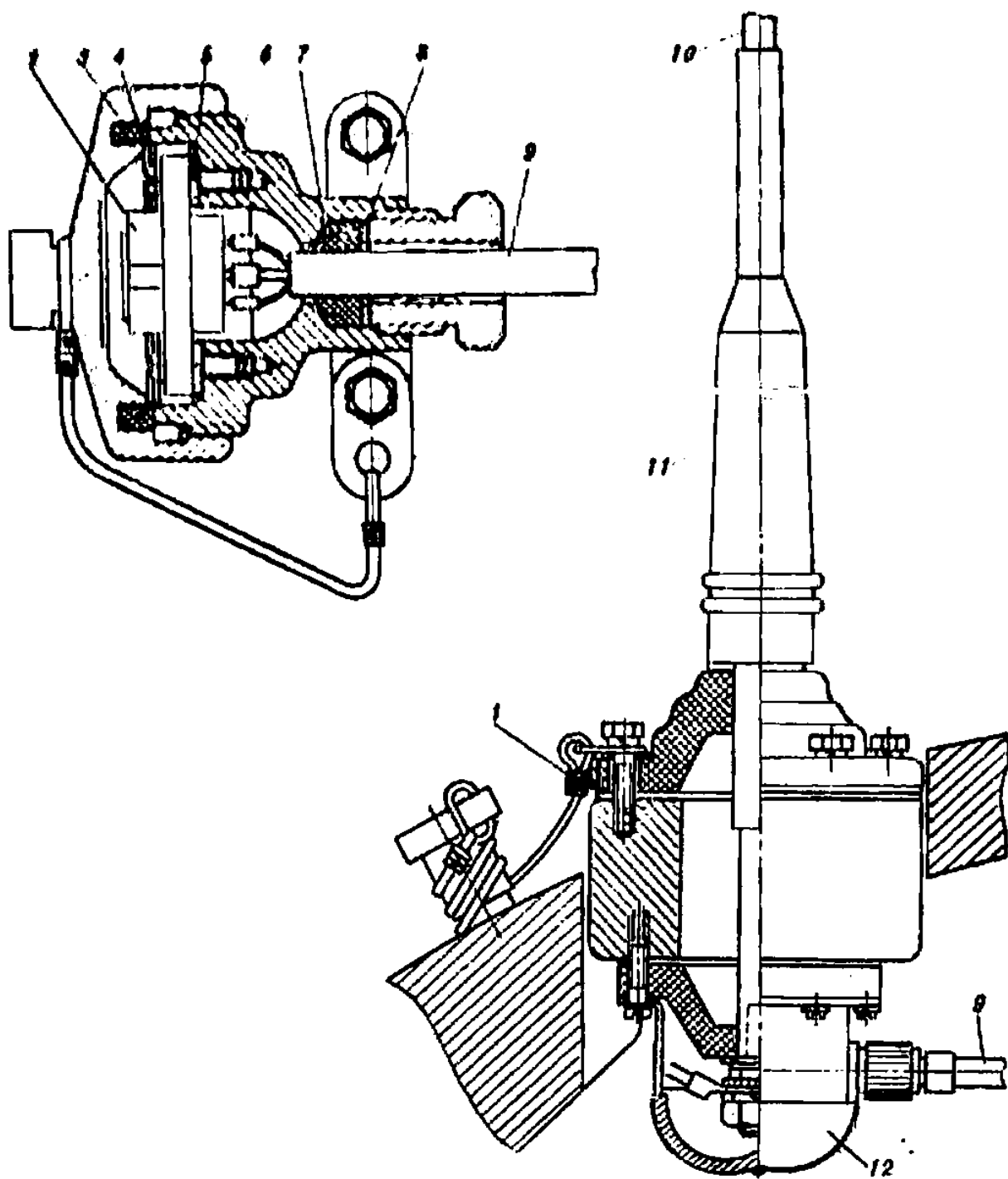
Рис. 119. Антенный ввод
