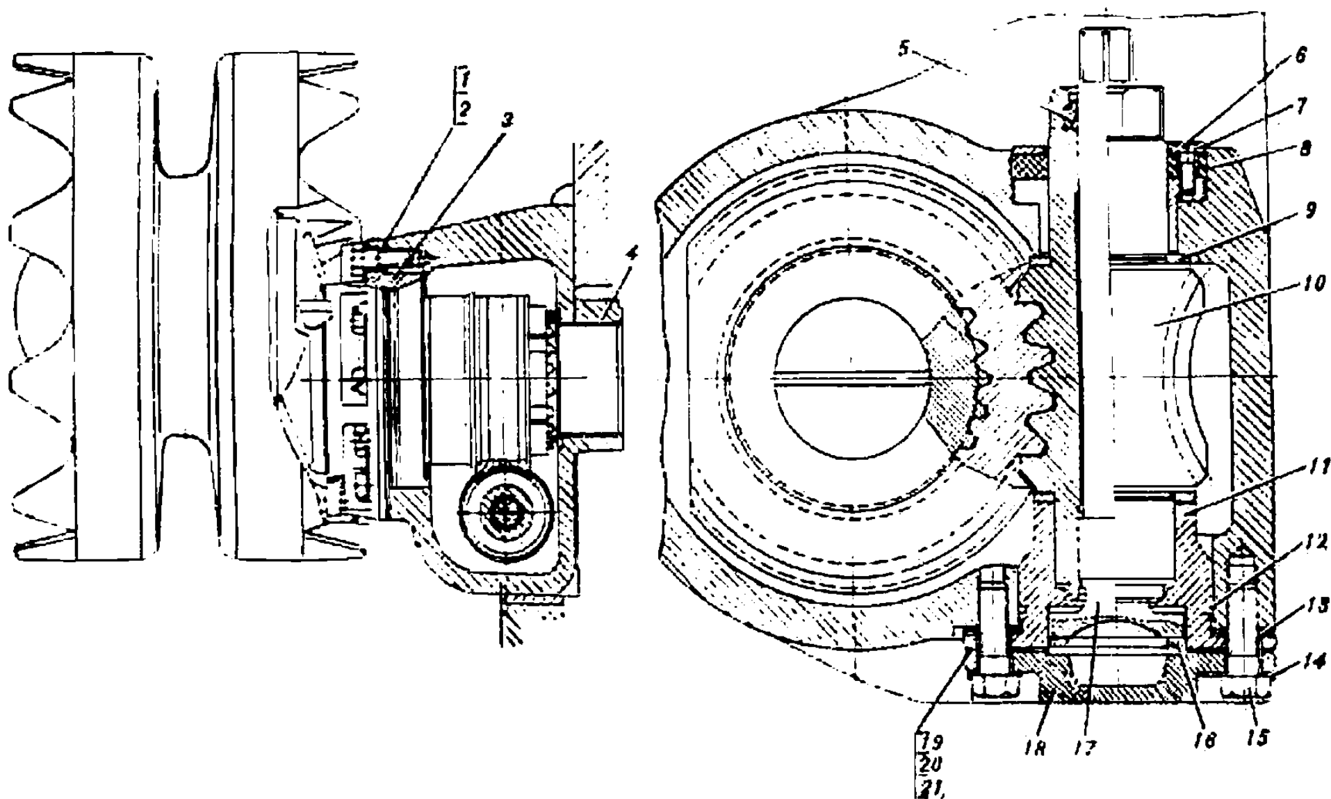
Рис. 36. Механизм натяжения гусеницы с направляющим колесом (155.15сб-3)
