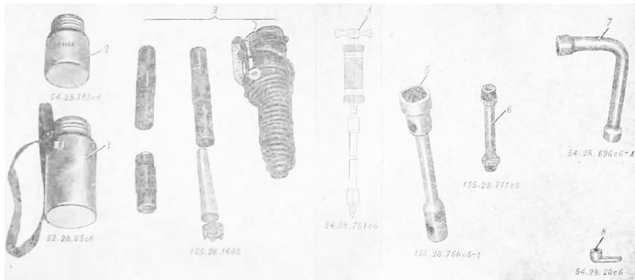
Рис. 79. Инструмент и принадлежности экипажа
