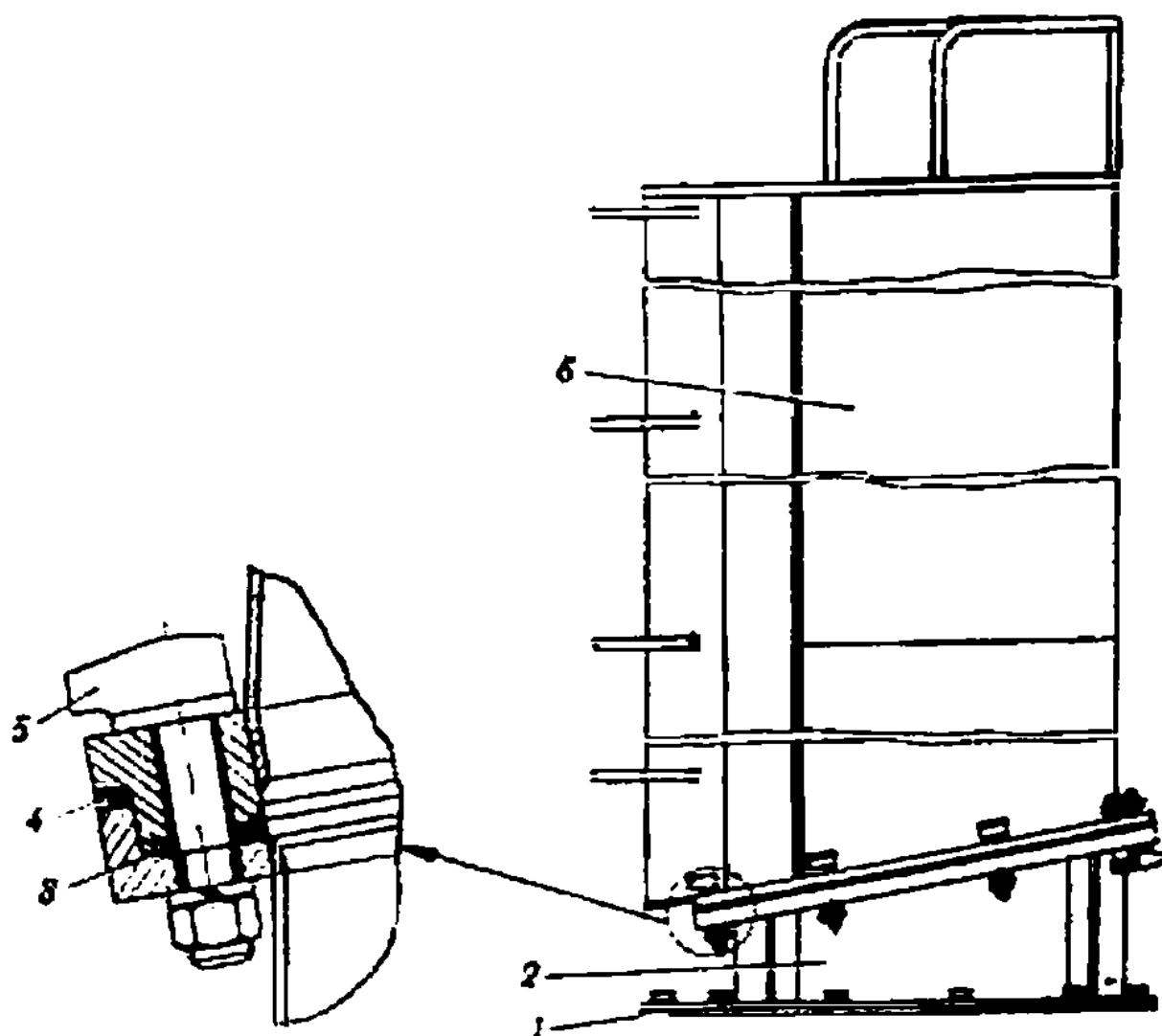
Рис. 157. Установка трубы лаза (166.83.25с6)
