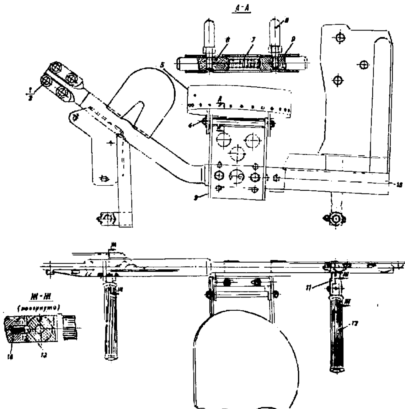
Рис. 125. Сиденье левое переднее (166.35.4с6)
