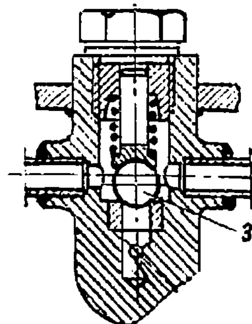
Клапаны ТДА
