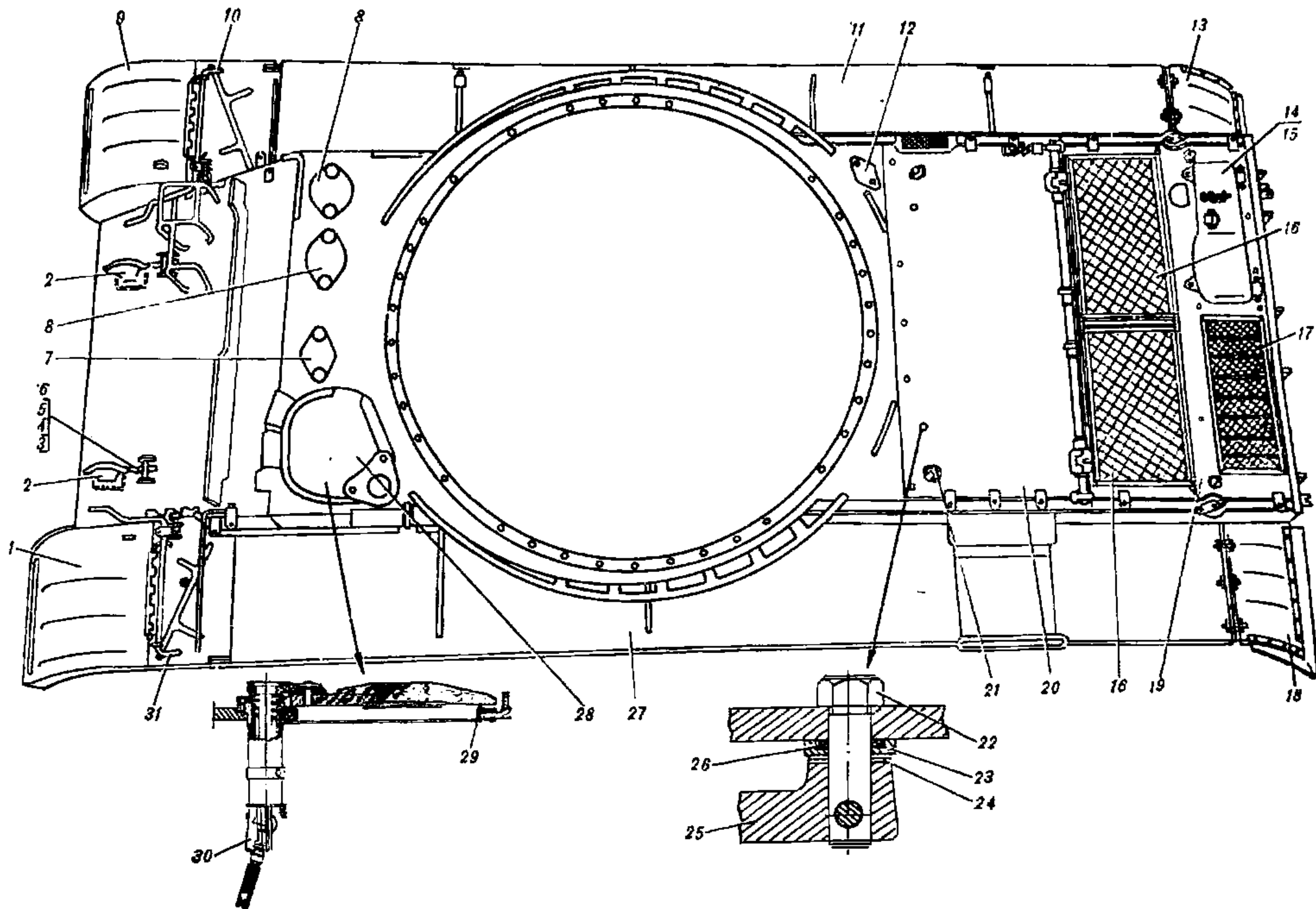
Рис. 83. Крыша
