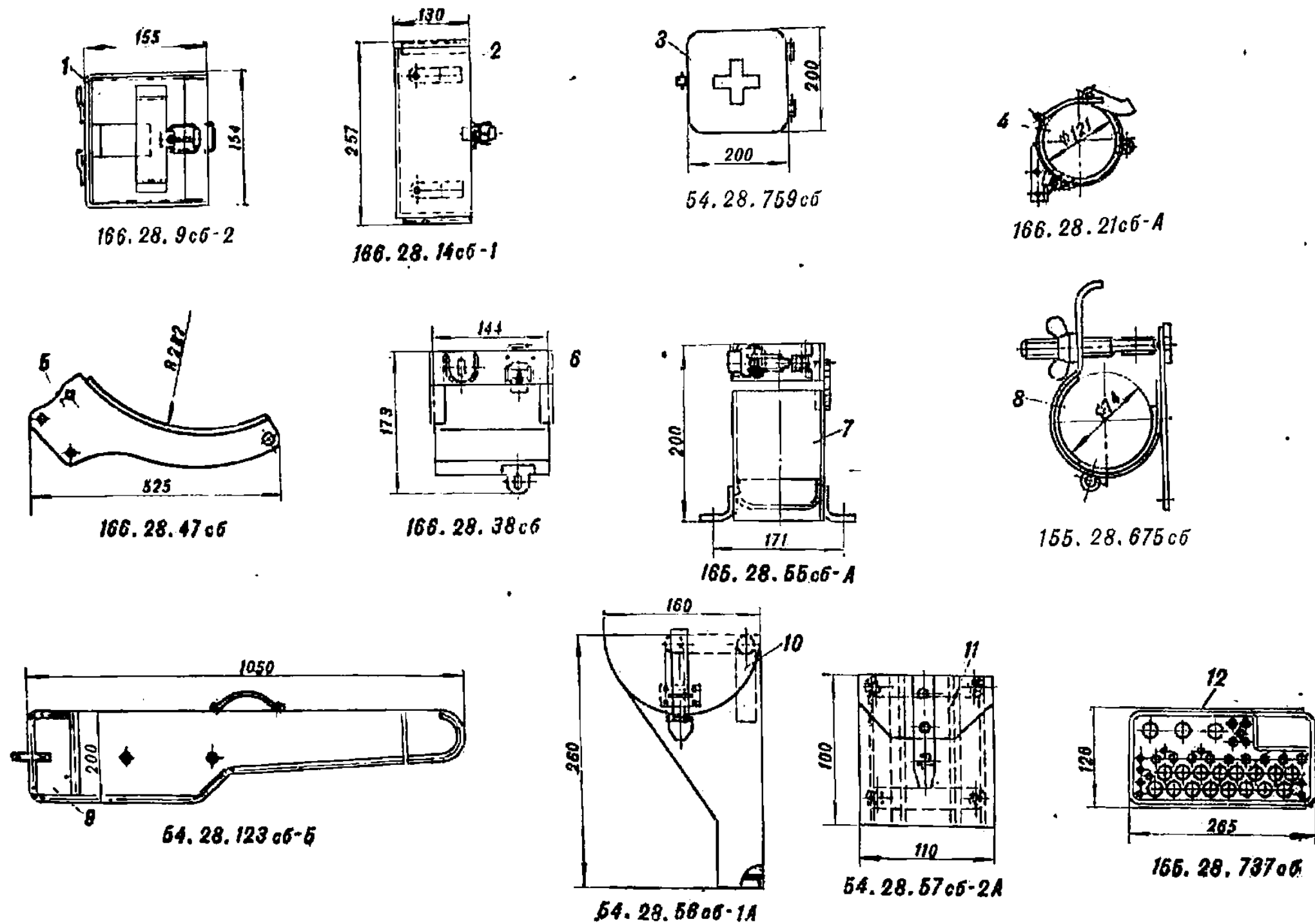
Рис. 75. Узлы крепления и укладки ЗИП
