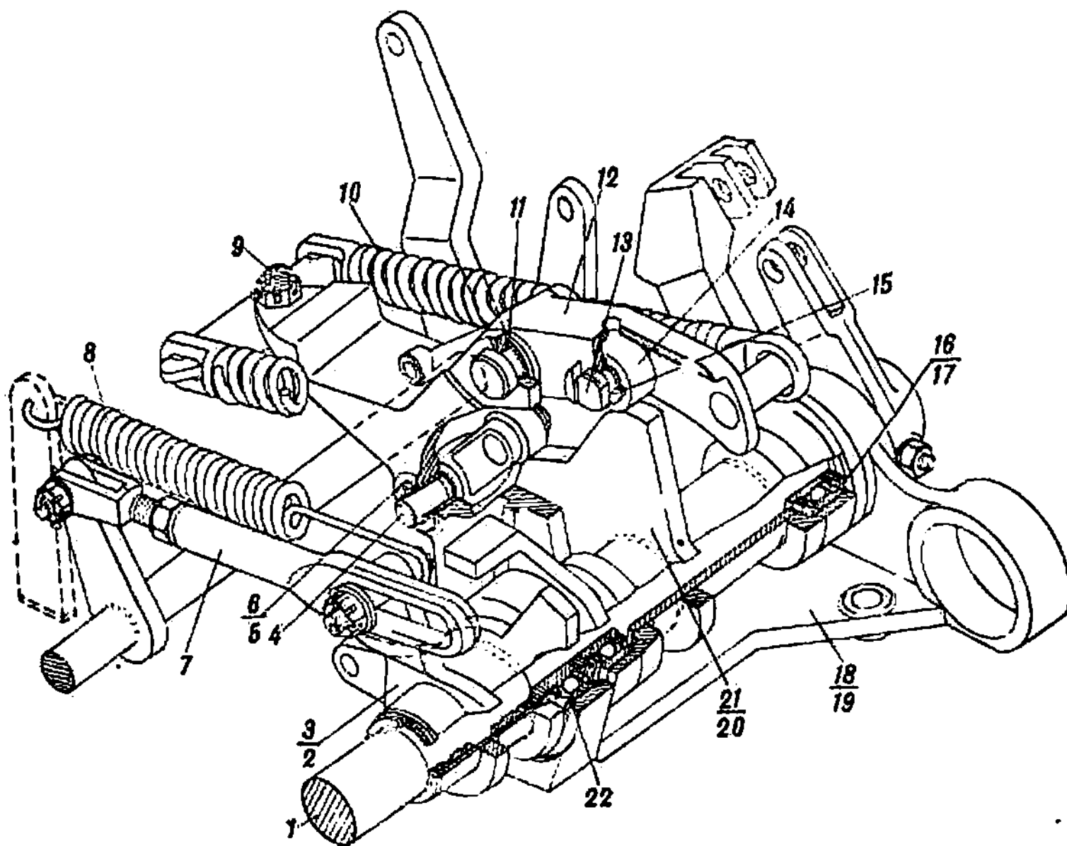
Рис. 48. Мостик управления механизма поворота (левого)
