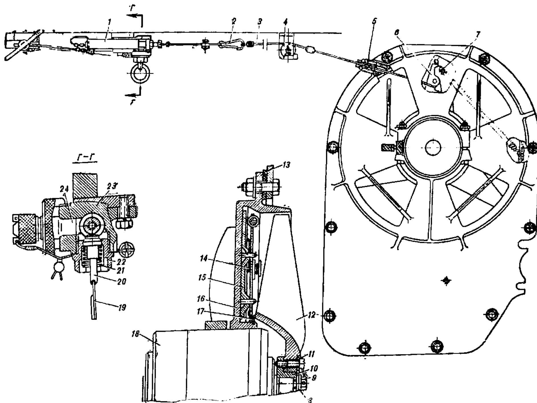
Рис. 101. Вентилятор (165.30.40сб)
