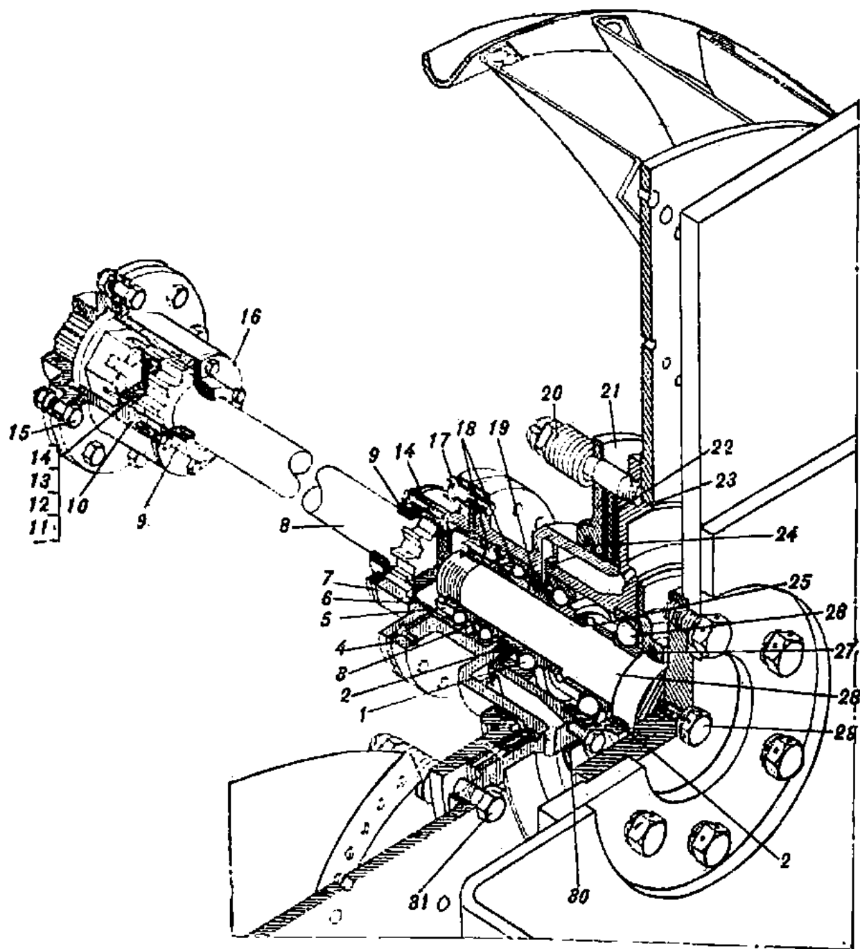
Рис. 142. Фрикцион вентилятора (54.41сб-1А)
