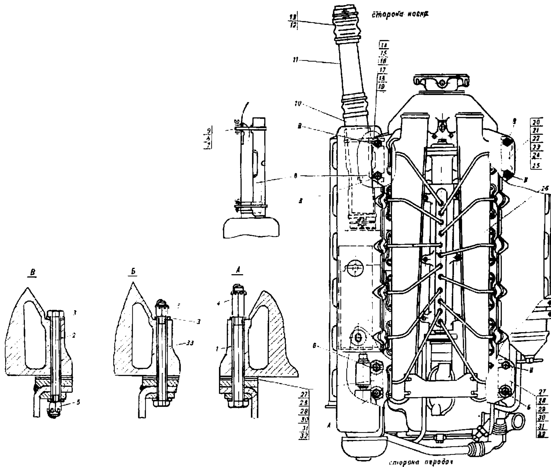
Рис. 1. Установка двигателя (166.01сб)
