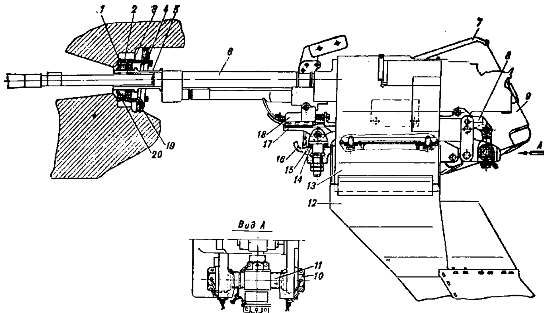
Рис. 106. Установка пулемета ПКТ (166.31.40с6)
