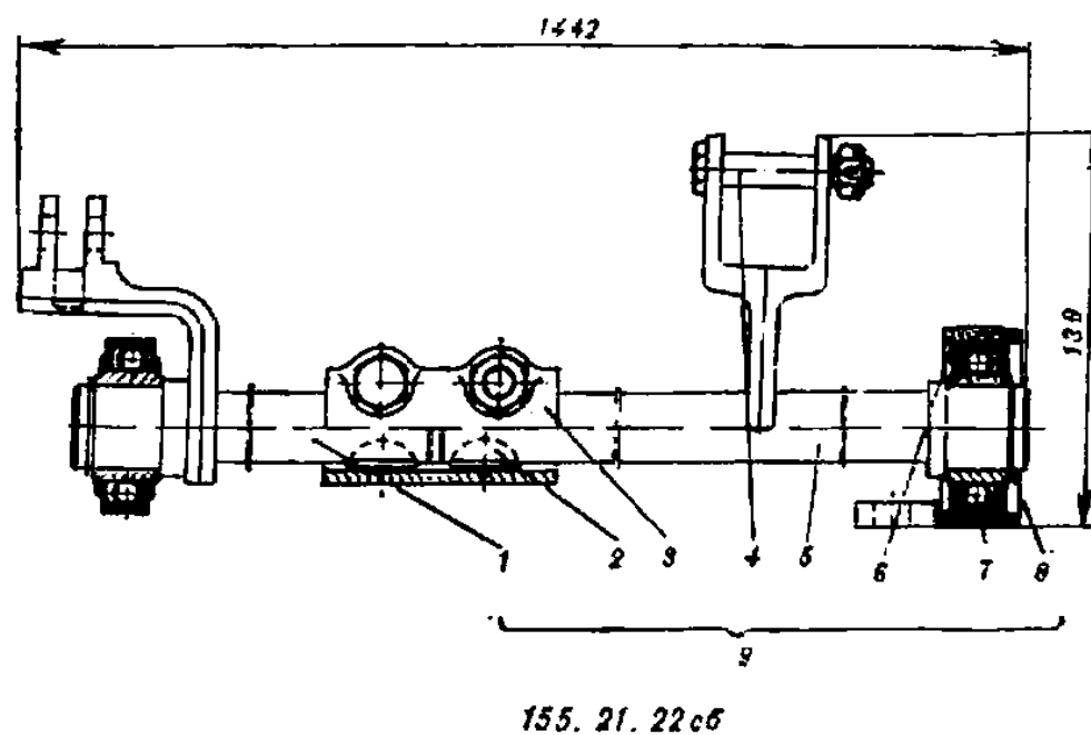
Рис. 53. Узлы привода управления главным фрикционом
