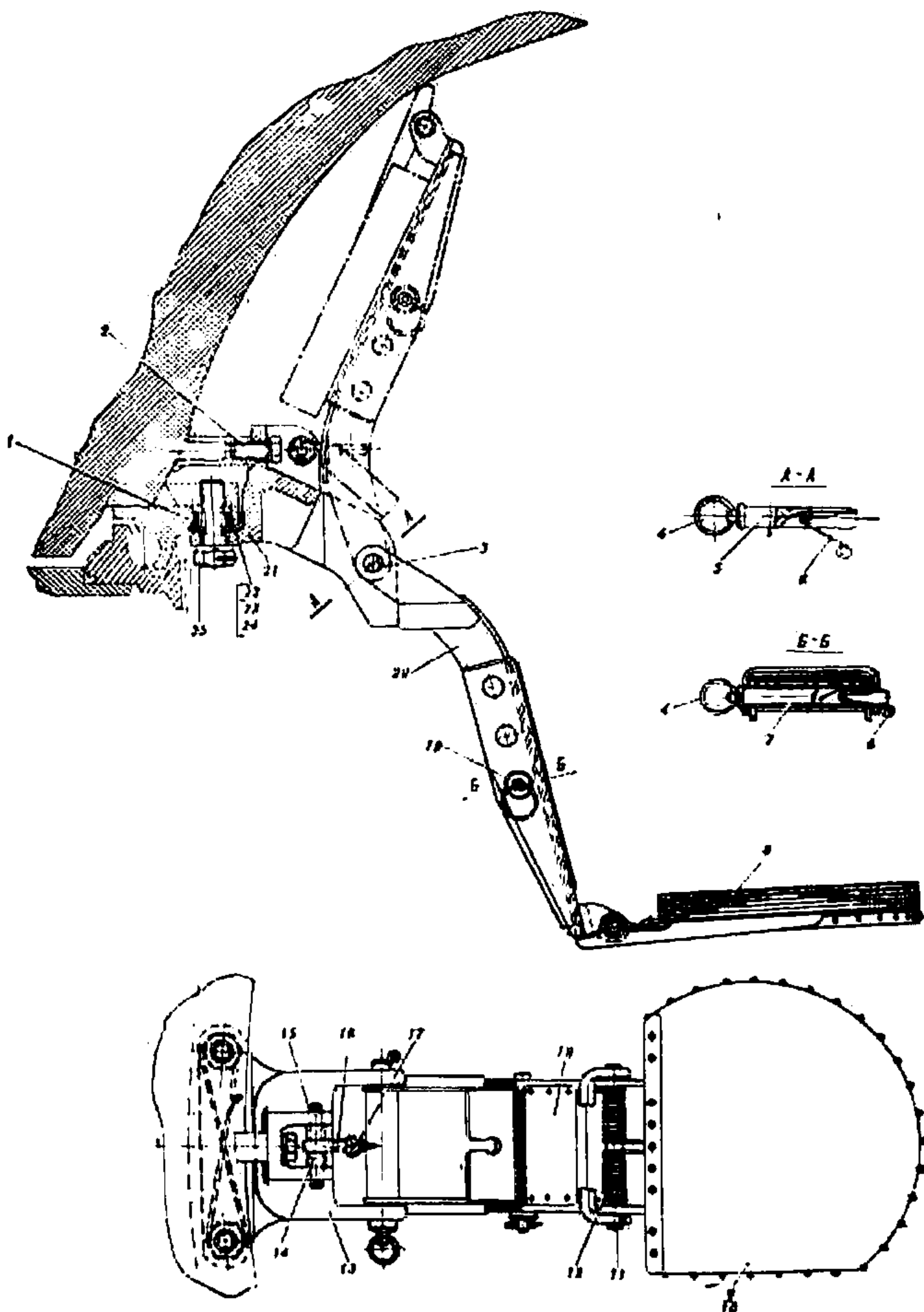
Рис. 123. Установка правого сиденья (166.35.17с6-1)
