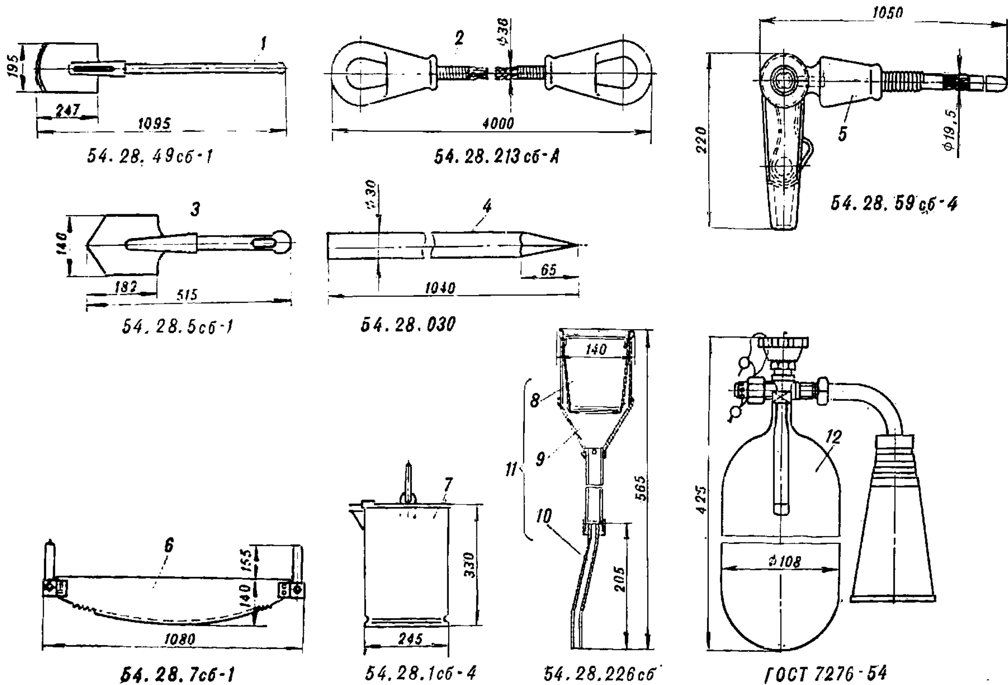
Рис. 81. Шанцевый инструмент и принадлежности
