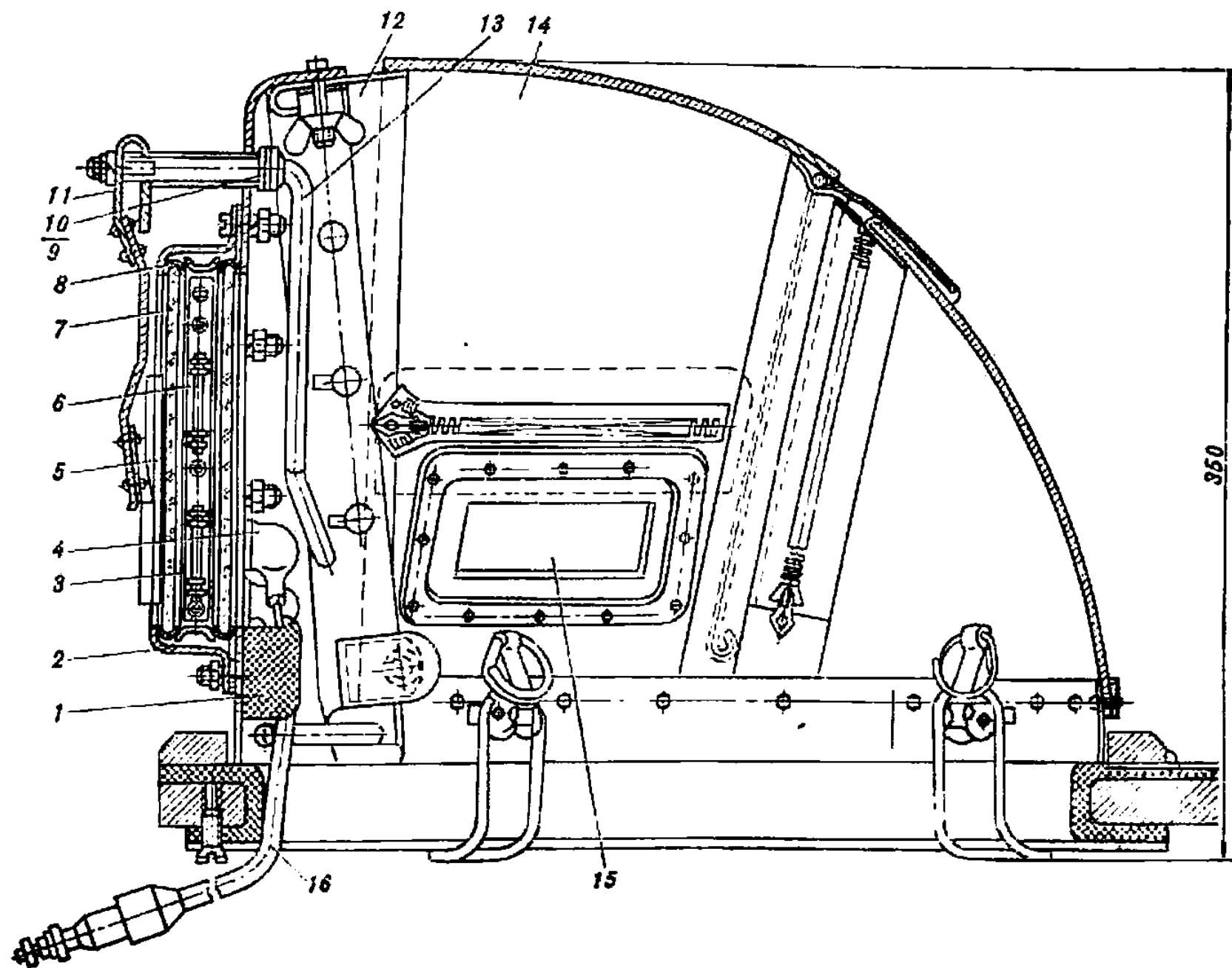
Рис. 92. Защитный колпак (155.29.112с6-А)
