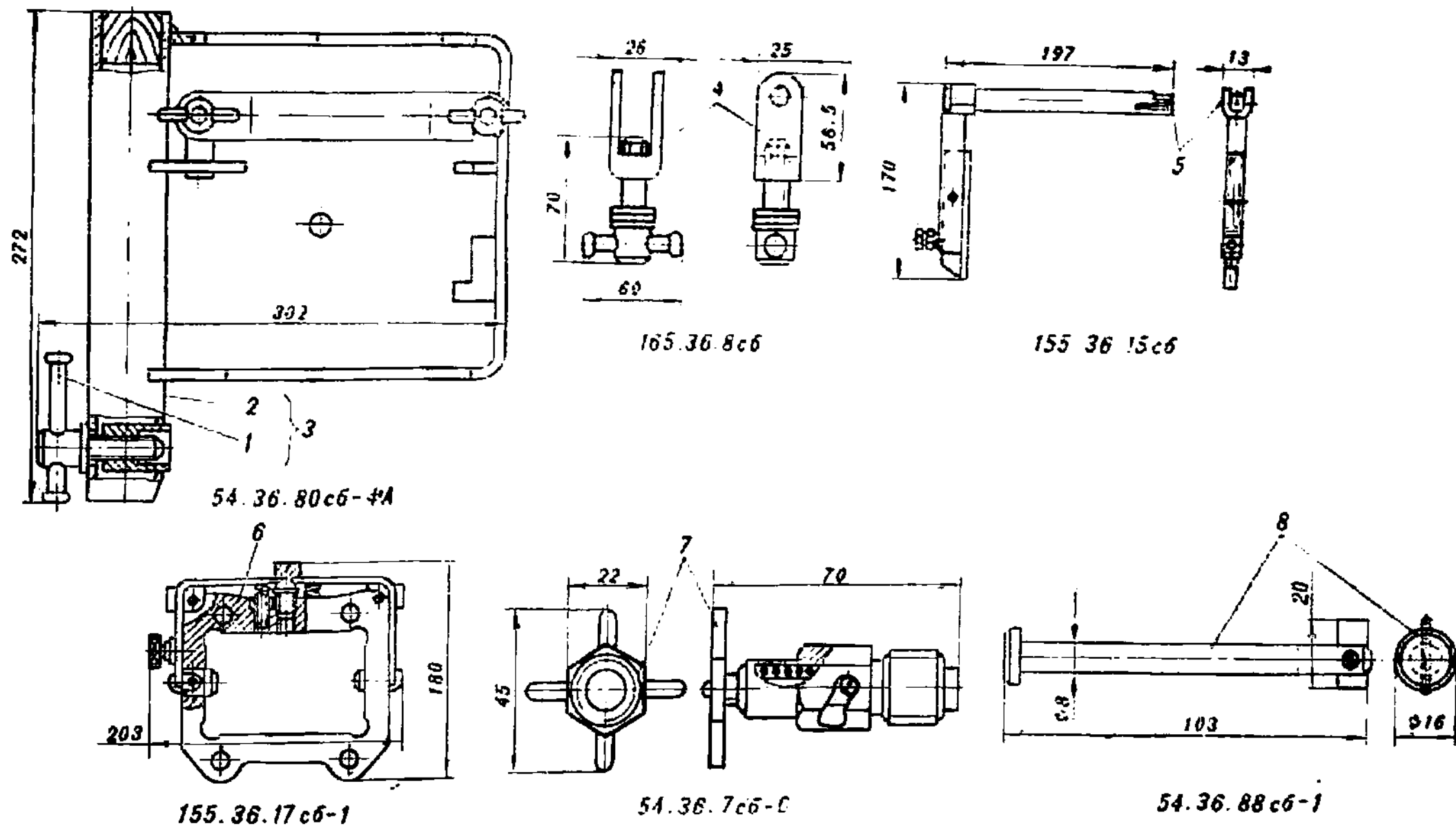
Рис. 131. Узлы крепления смотровых приборов
