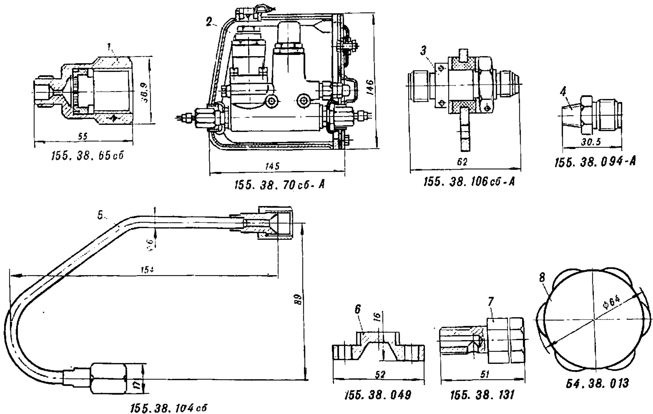
Рис. 136. Узлы и детали воздушной системы
