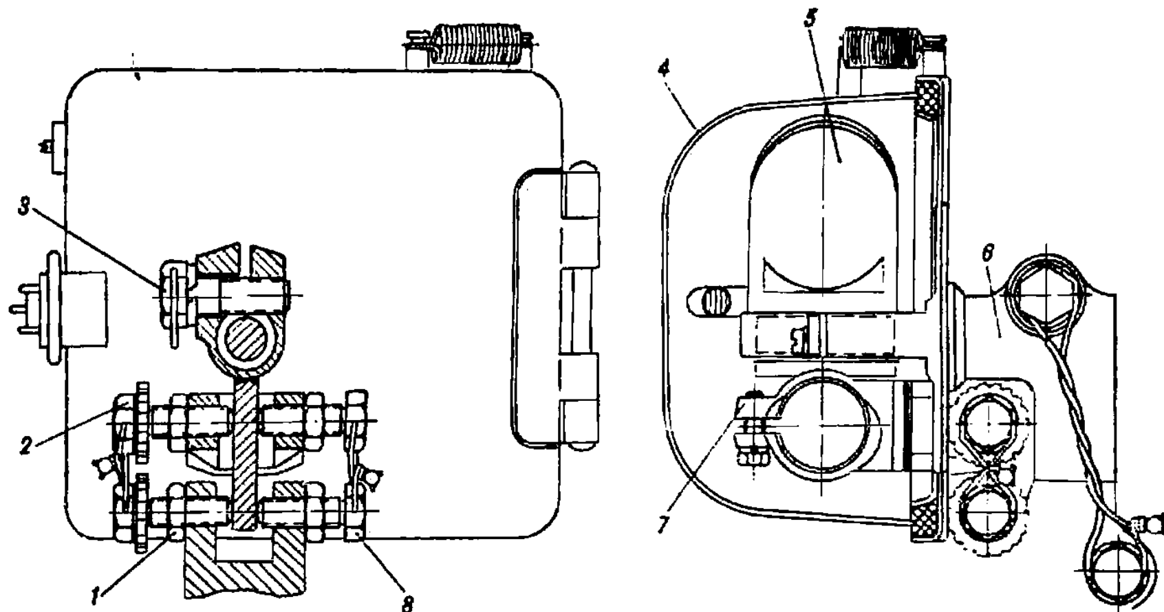
Рис. 114. Установка прибора К-10Т (155.32.3сб-1А)
