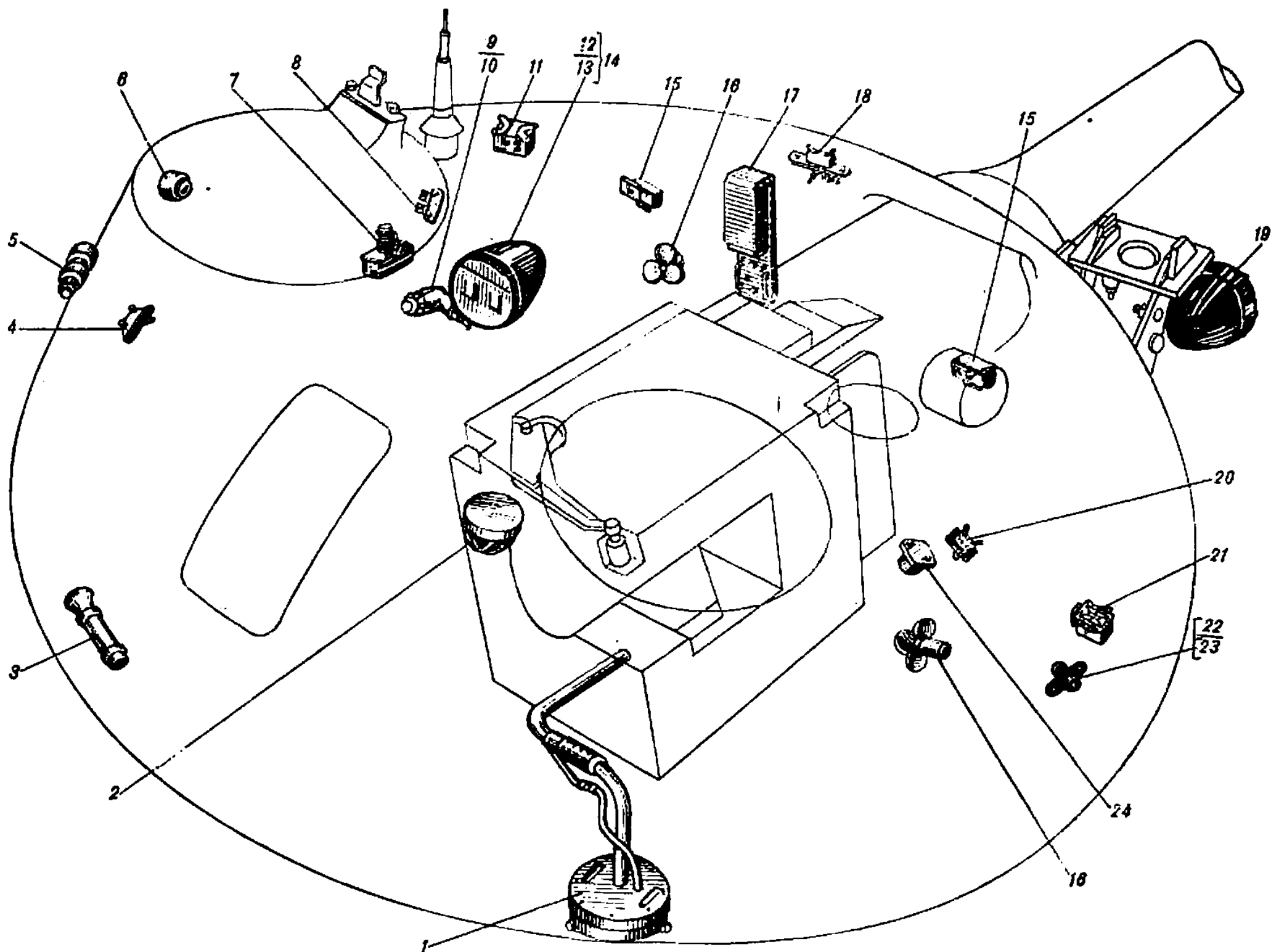
Рис. 59. Размещение электрооборудования в башне
