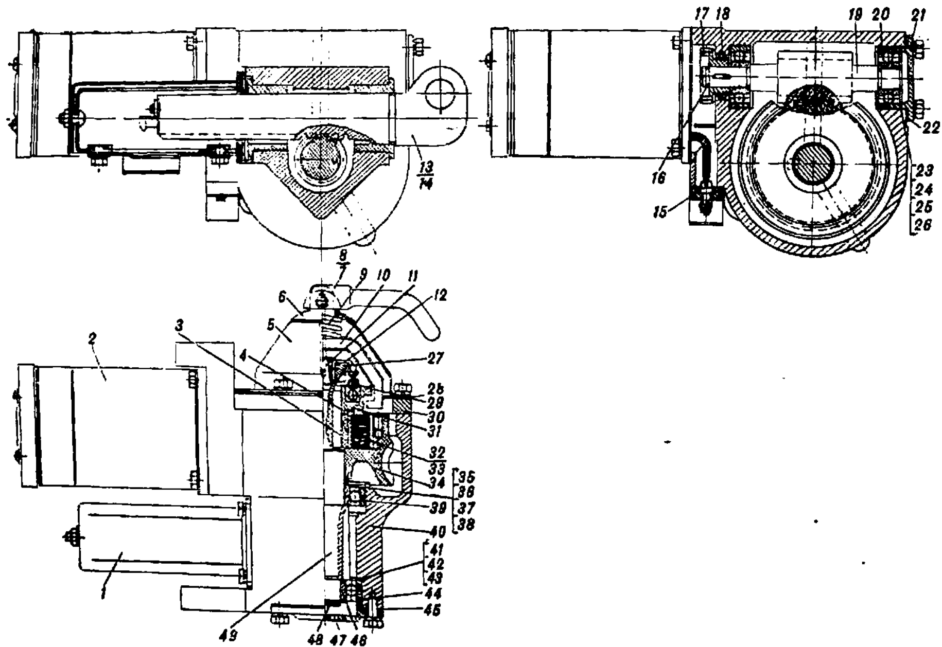
Рис. 41. Редукторы (165.17.62сб-1 и 165.17.65сб-1)
