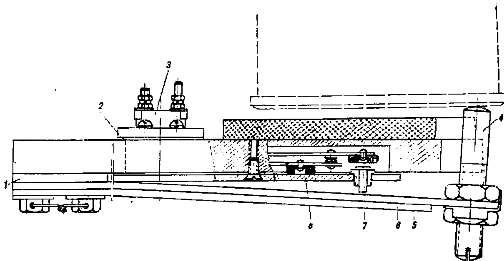
Рис. 42. Узлы включения электрической системы механизма выброса гильз
