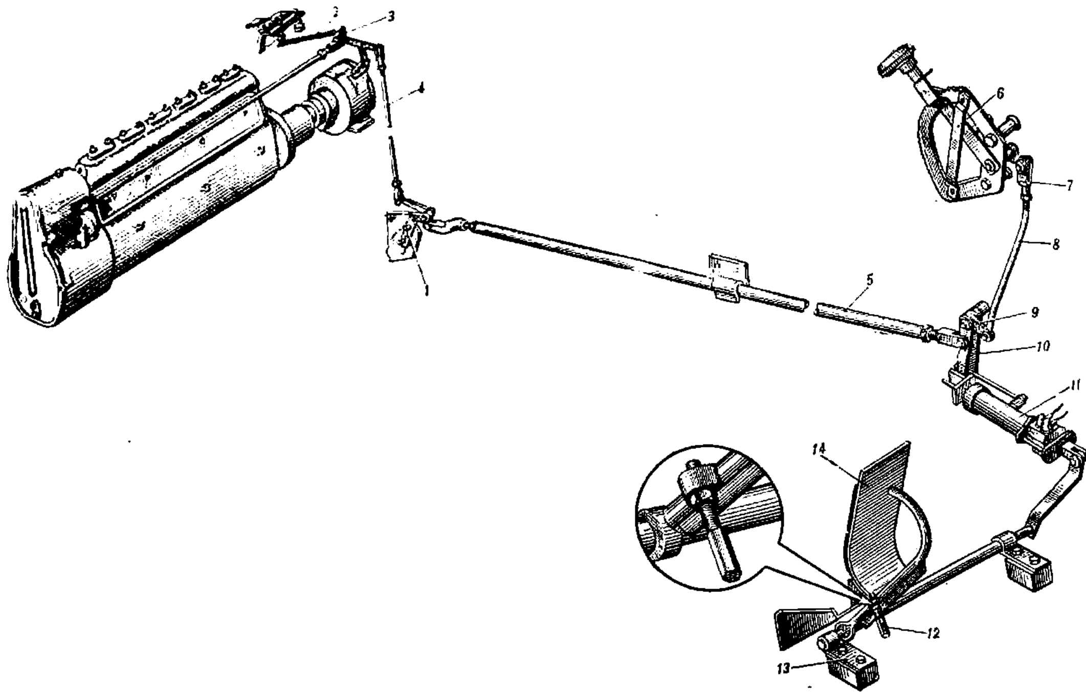
Рис. 54. Привод к топливному насосу (165.22с6-А)
