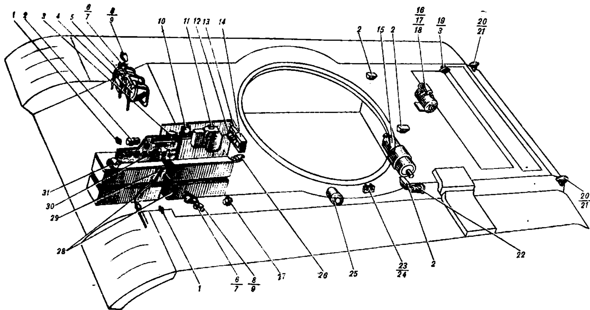
Рис. 58. Размещение электрооборудования в корпусе
