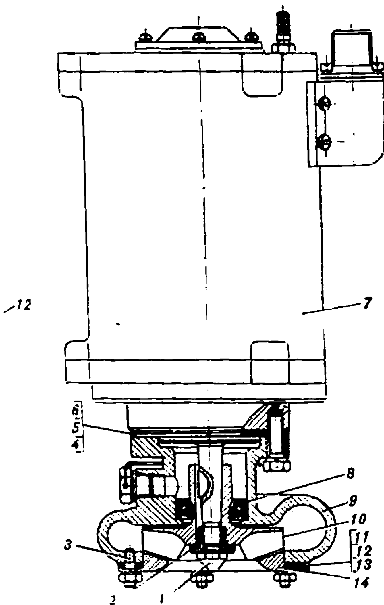
Рис. 159. Насос (54.83.78сб-А)
