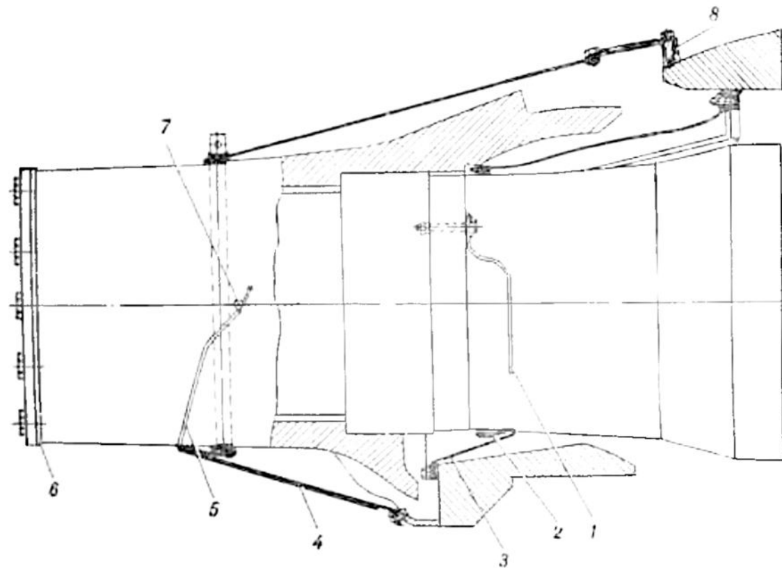
Рис. 105. Установка чехлов (166.31.2сб-1)
