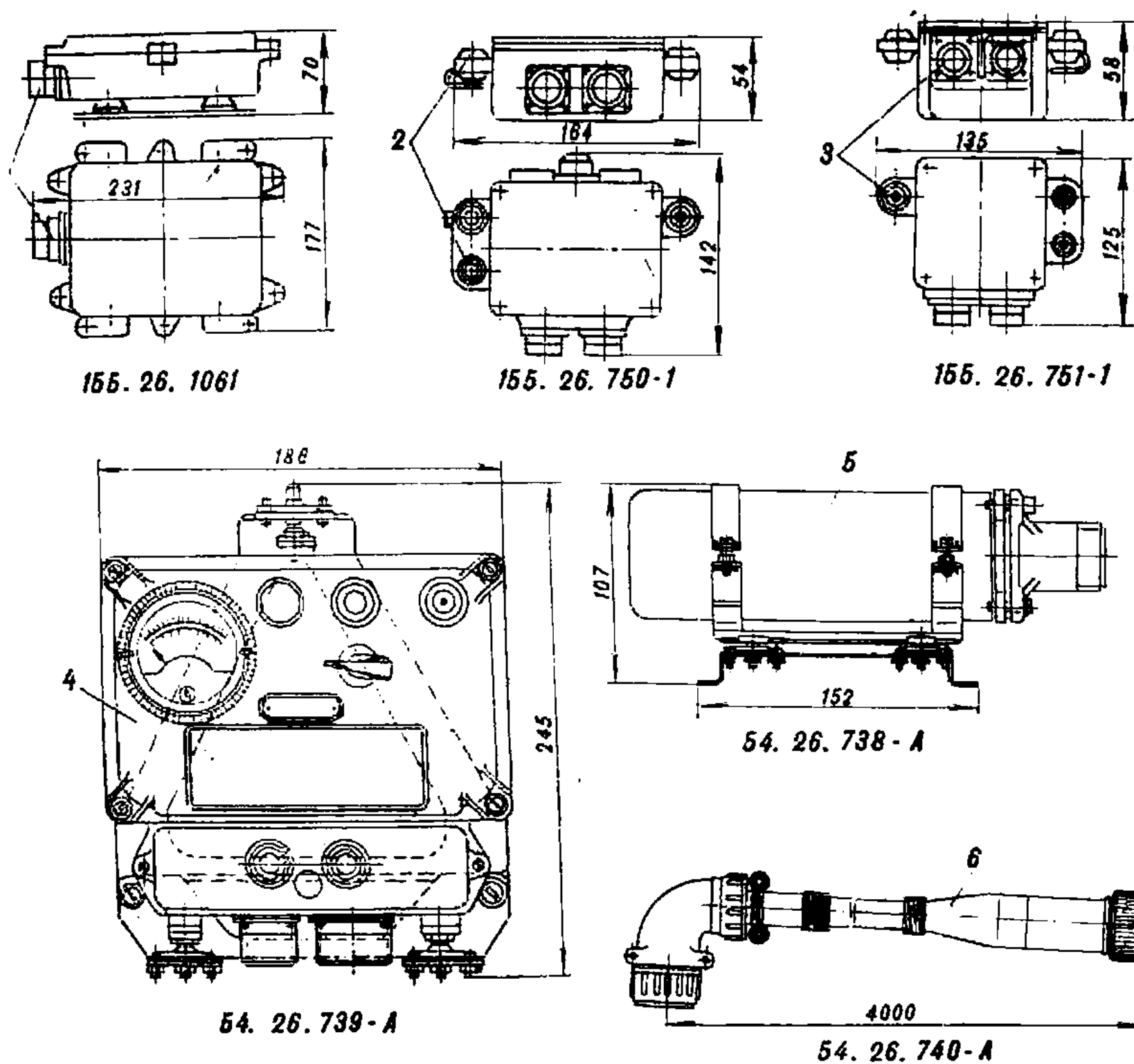
Рис. 68. Узлы системы противоатомной защиты
