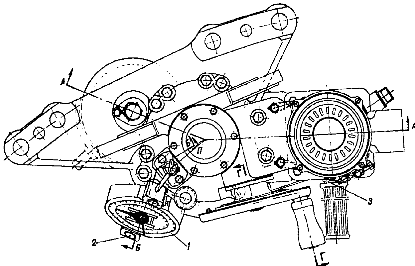
Рис. 120. Поворотный механизм (166.34сб-1)
