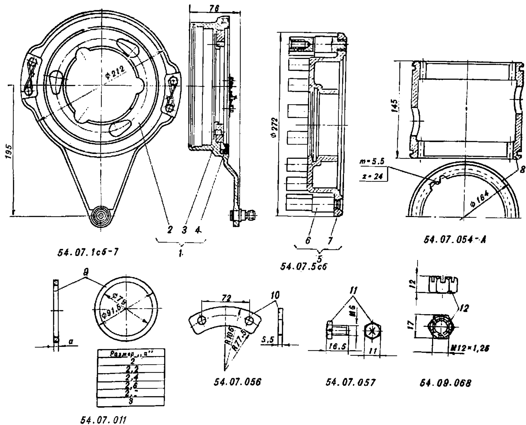
Рис. 17. Детали главного фрикциона
