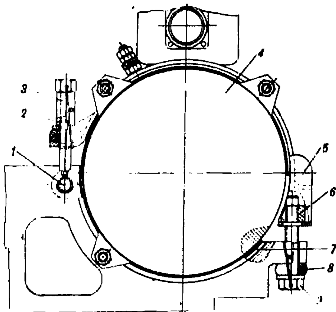
Рис. 151. Установка электромашинного усилителя (166.55.11сб-1)
