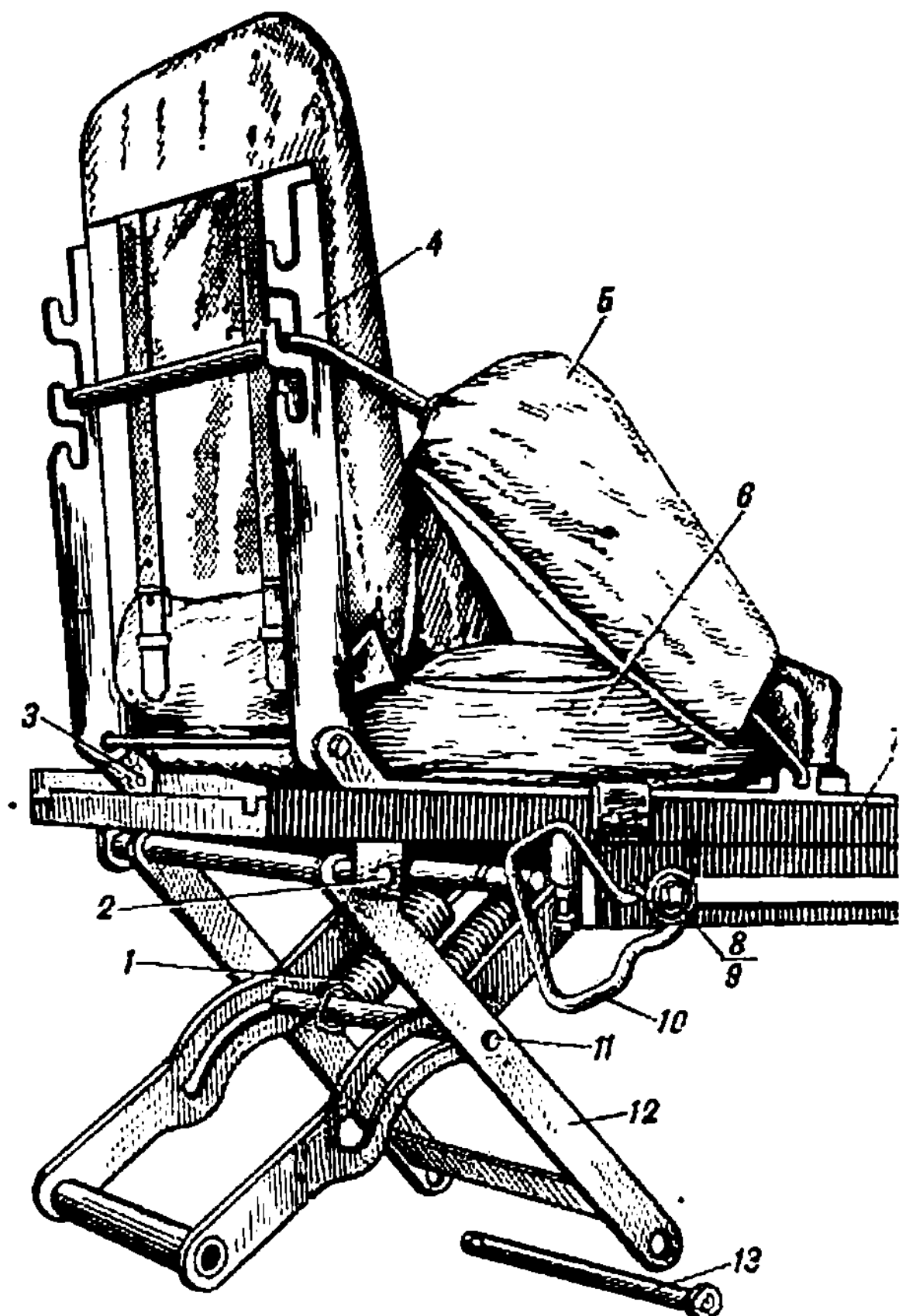
Рис. 57. Сиденье водителя (155.25сб-2)
