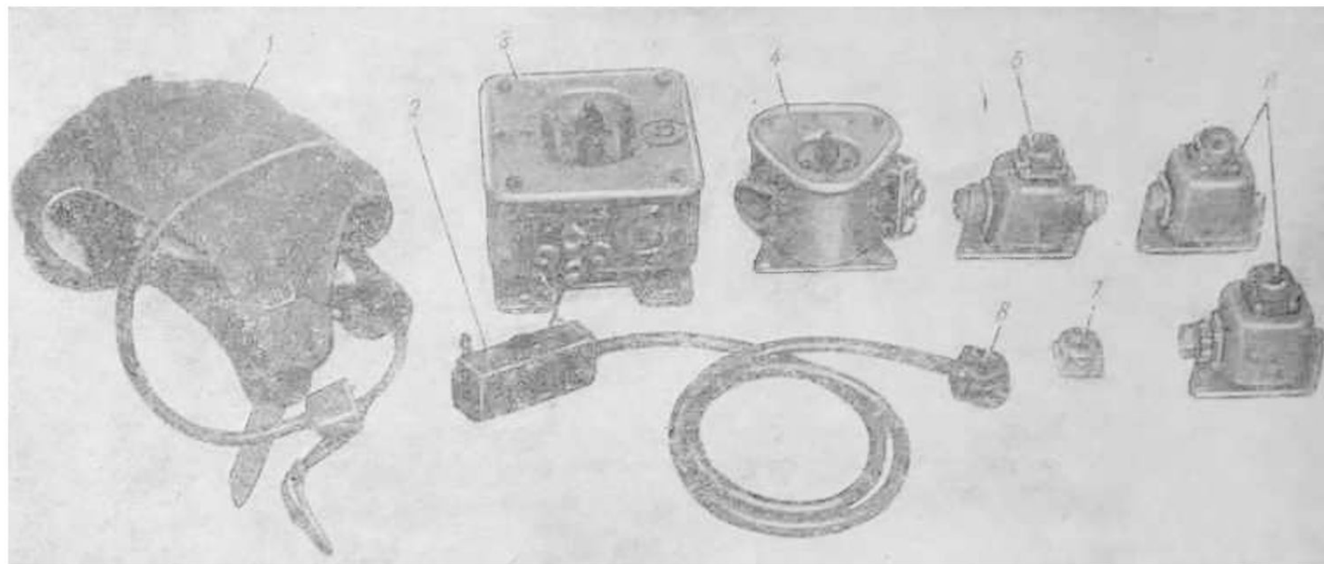
Рис. 118. Комплект ТПУ Р-124 и шлемофон
