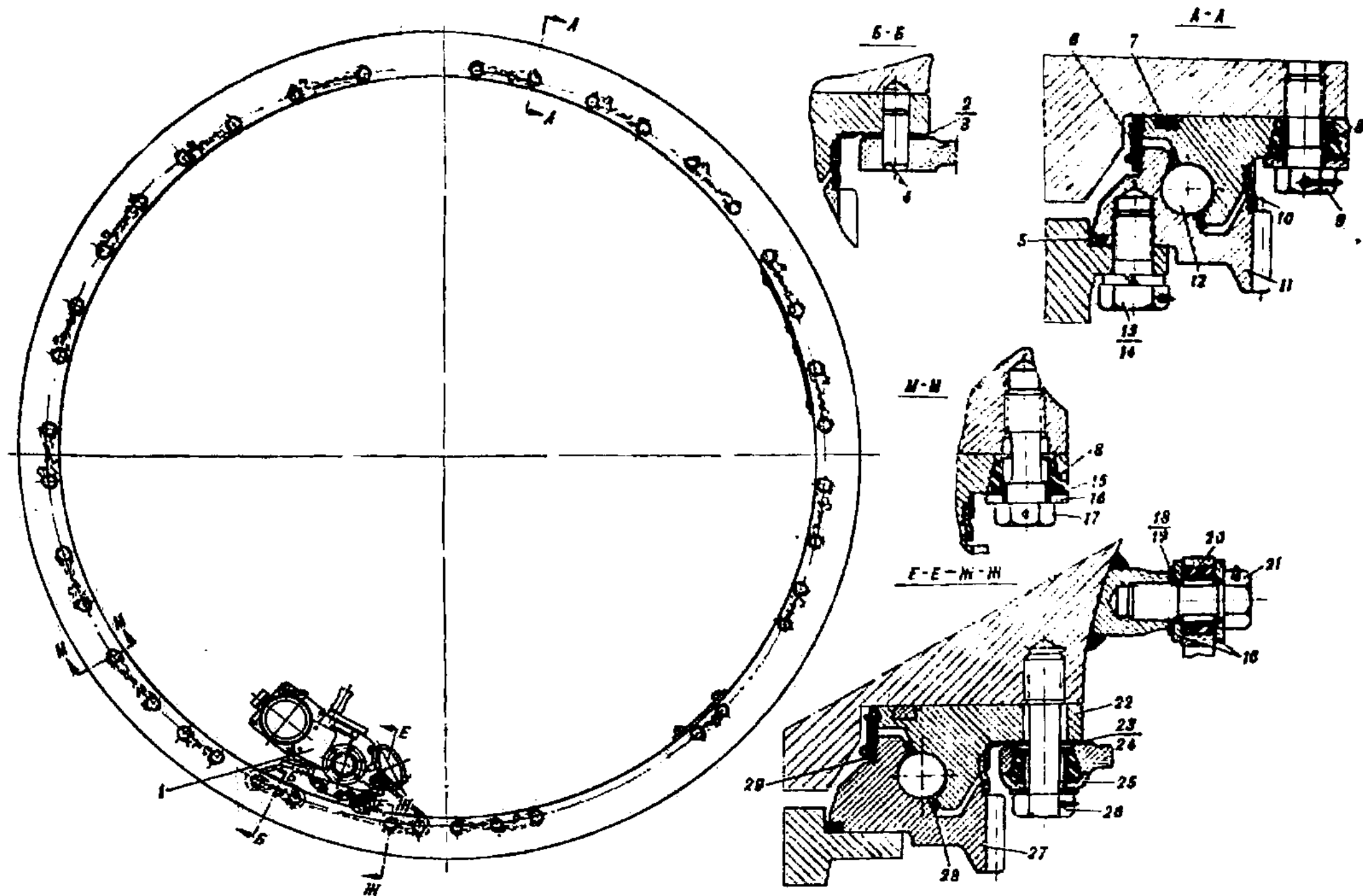
Рис. 95. Установка погона и поворотного механизма башни (165.30.20с6-1)
