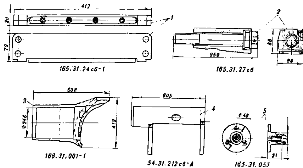
Рис. 103. Установка осветителя Л-2Г (165.31.13с6)
