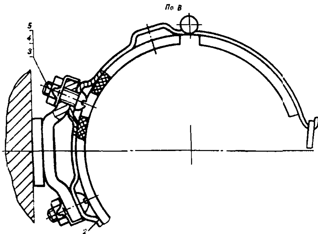
Рис. 183. Установка прибора ТДП
