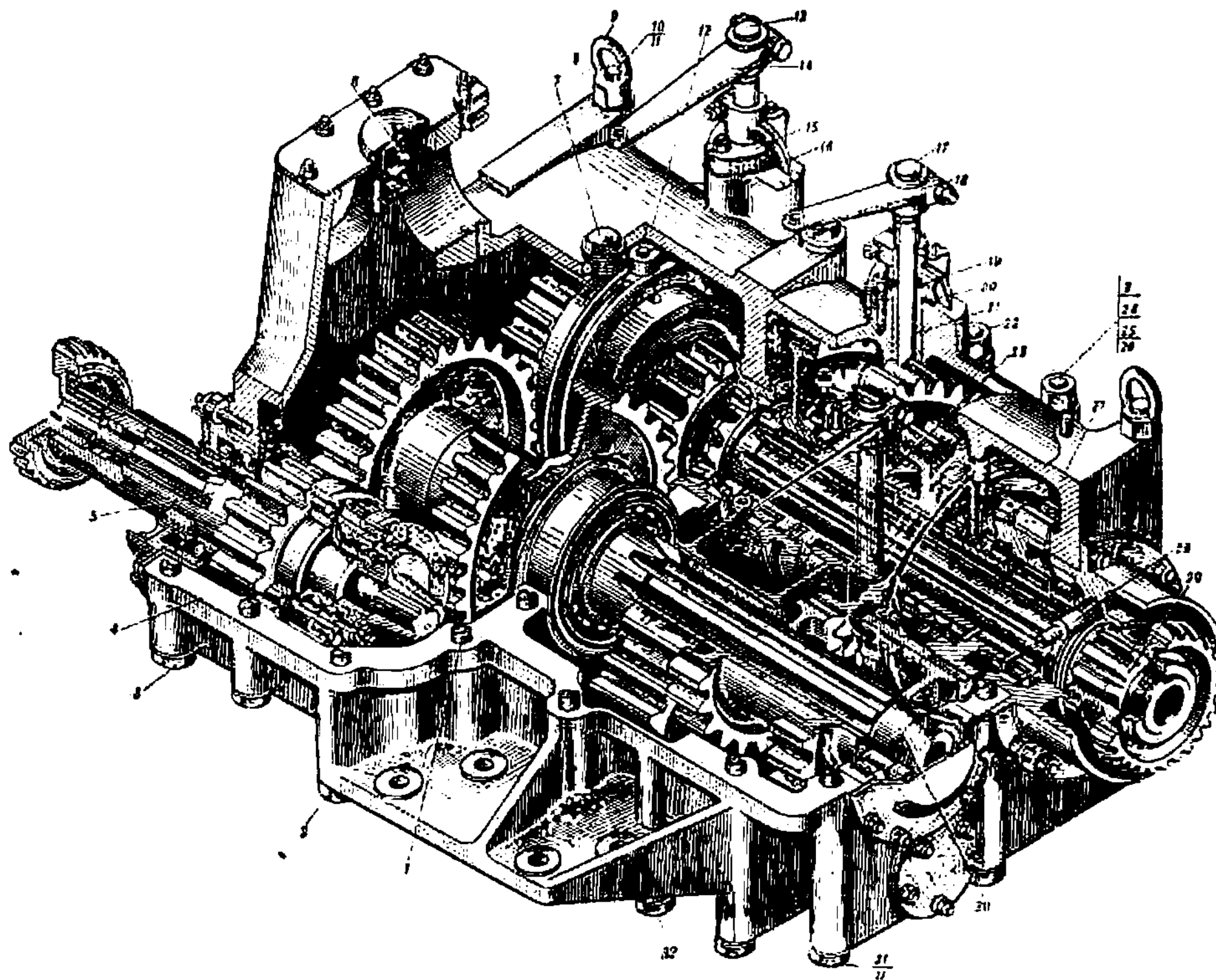
Рис. 18. Коробка передач (155.08сб-6)
