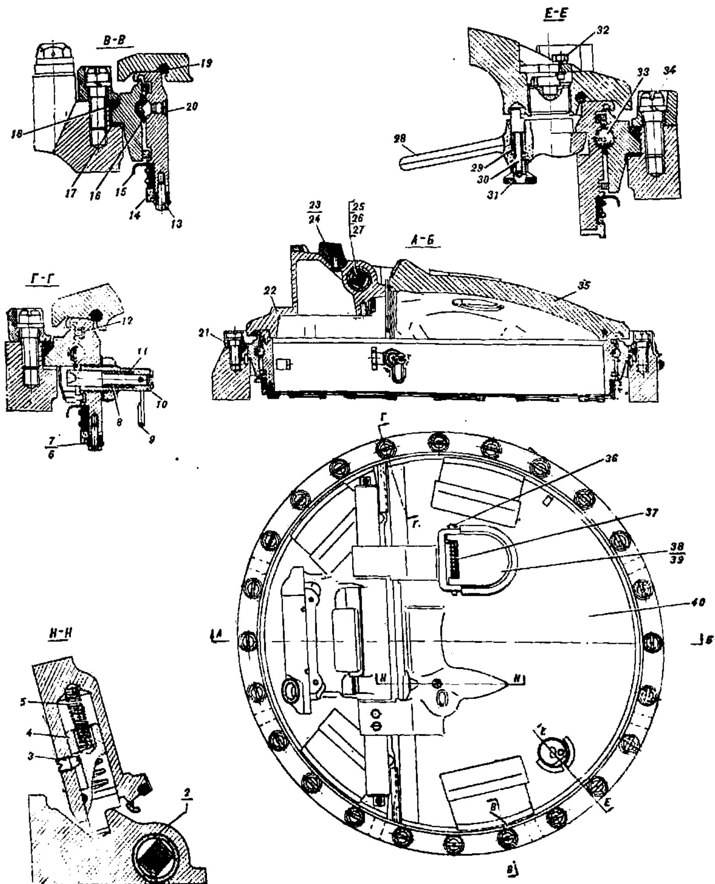
Рис. 97. Левый люк (165.30.3сб-1)
