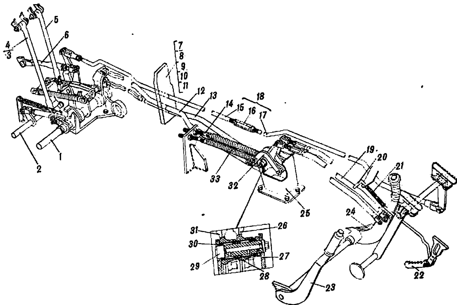
Рис. 47. Привод управления планетарным механизмом поворота (165.20с6-2)
