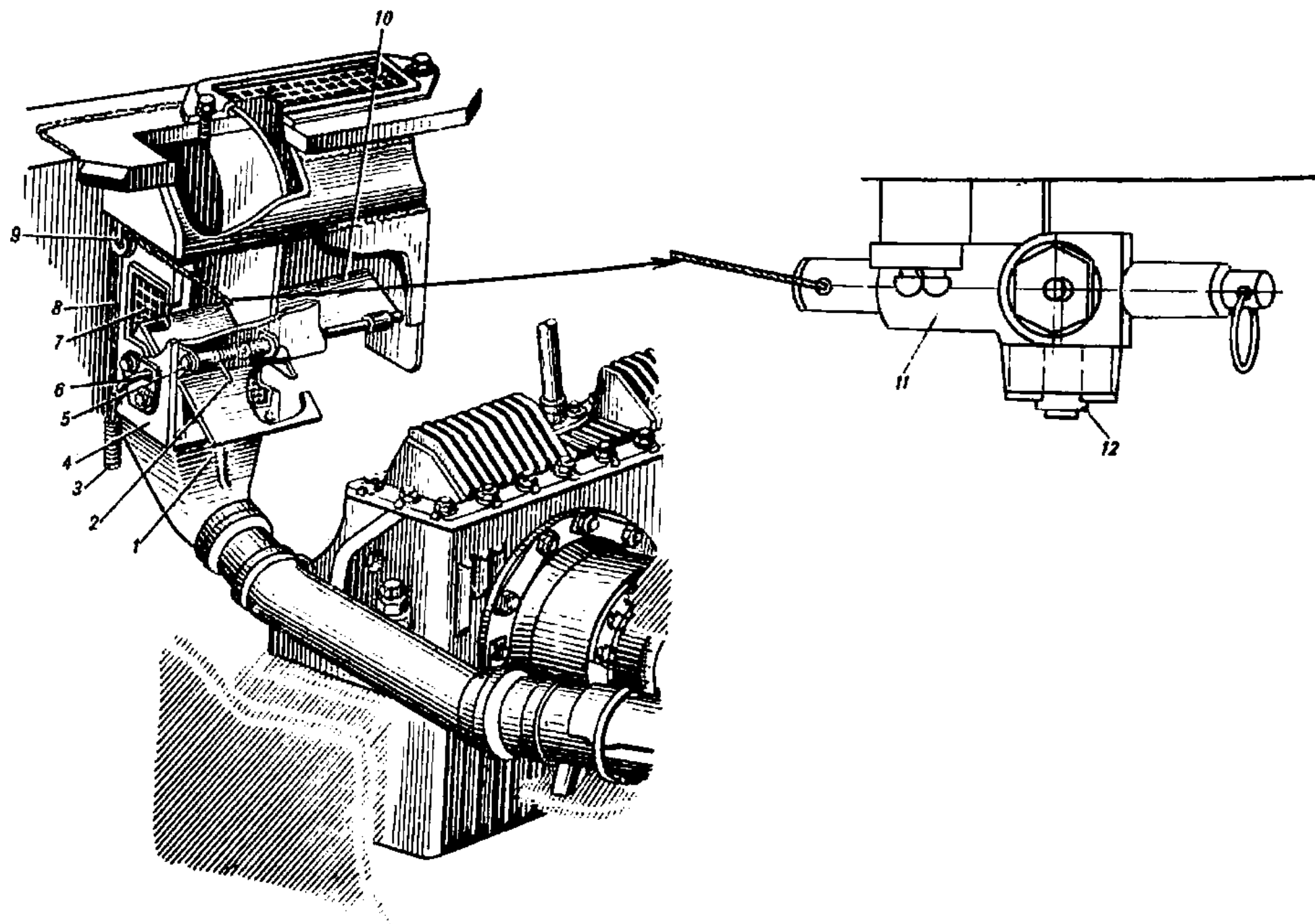
Рис. 90. Установка воздухопритока к генератору (165.29.71с6-2)
