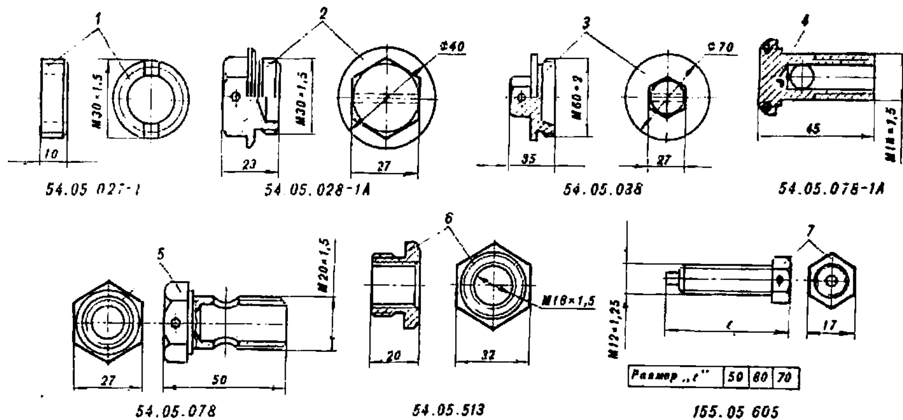
Рис. 15. Штуцера и пробки системы питания
