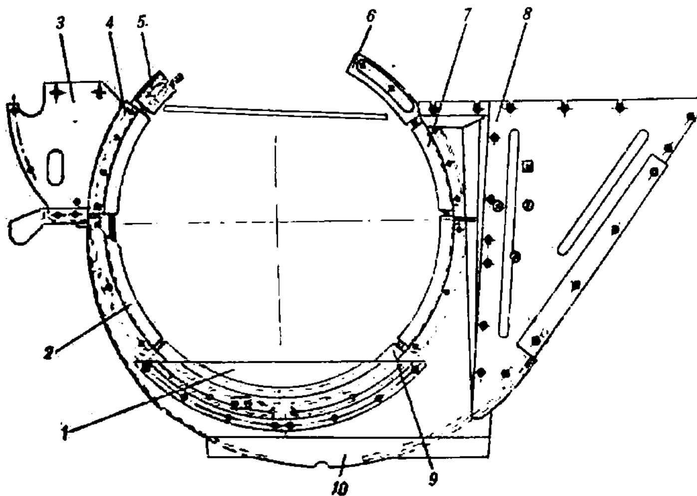
Рис. 86. Вентиляторная перегородка (166.29.72сб-2)
