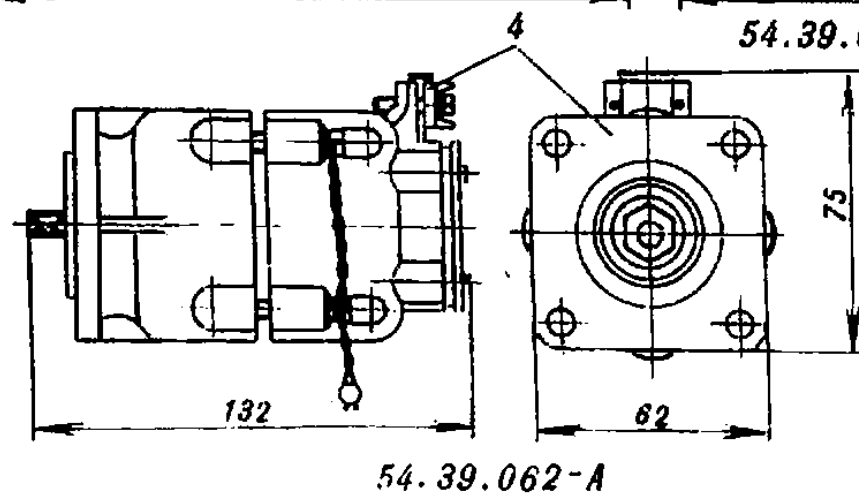
Рис. 137. Контрольно-измерительные приборы
