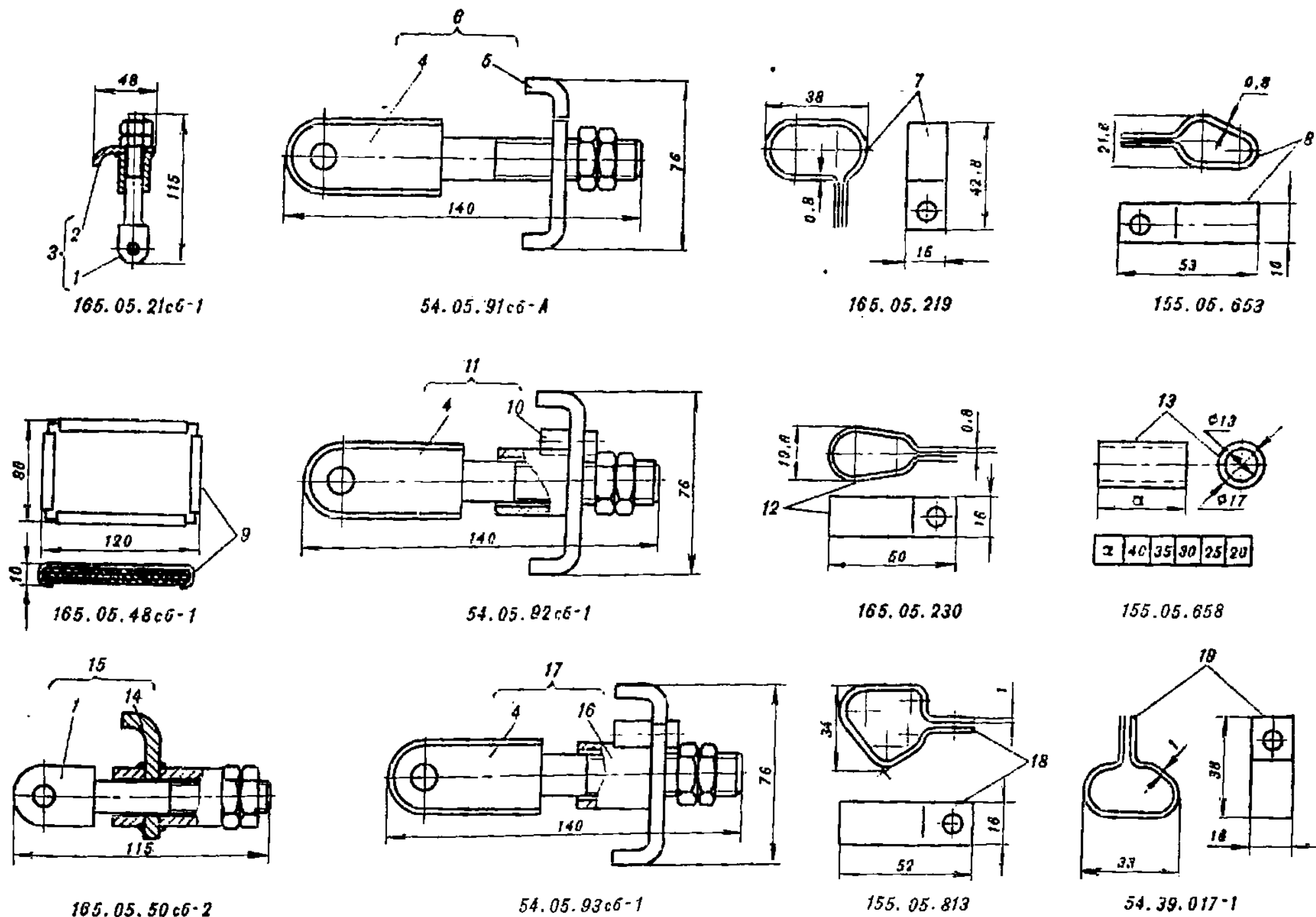
Рис. 13. Детали крепления системы питания
