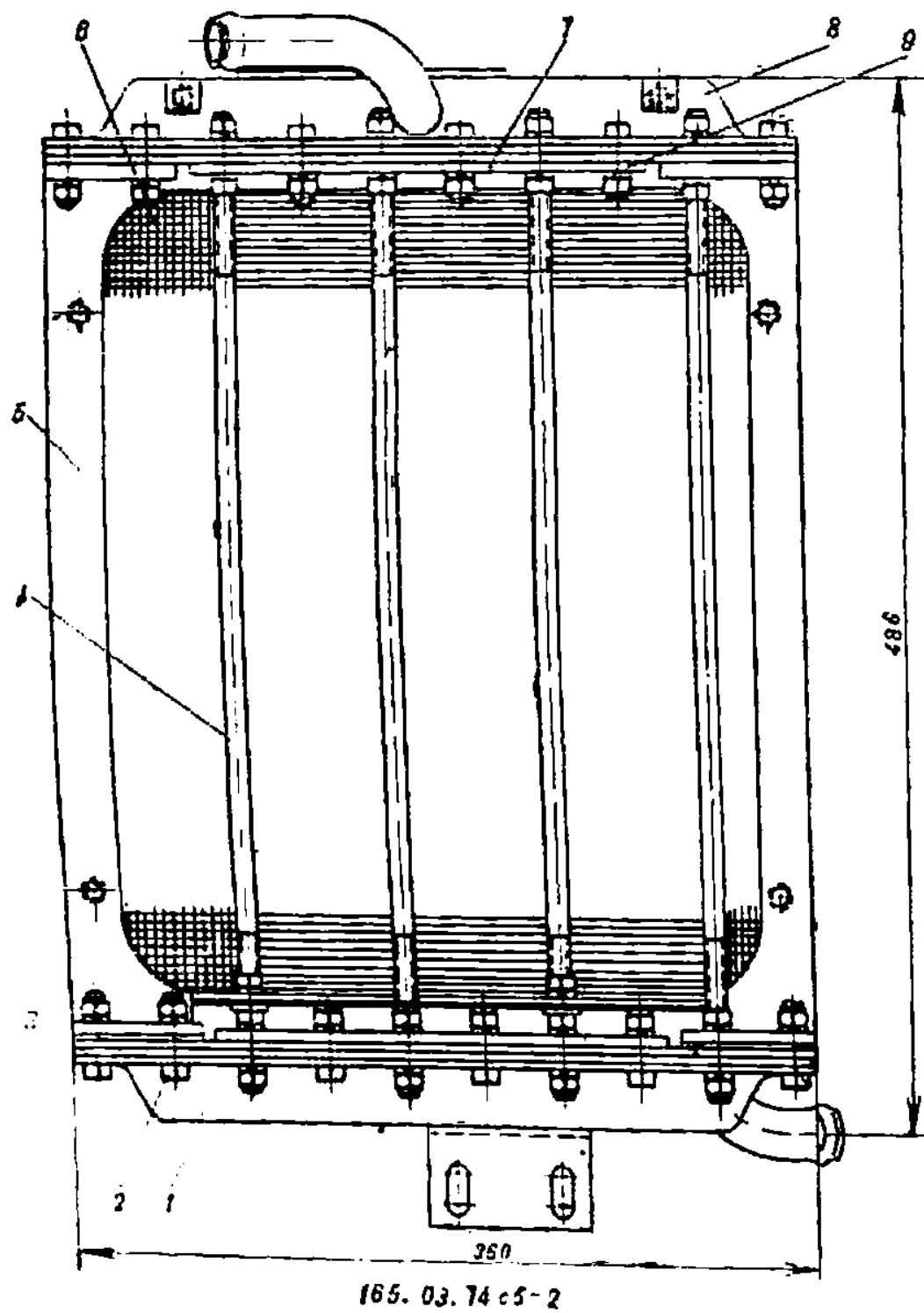
Рис. 7. Узлы системы смазки
