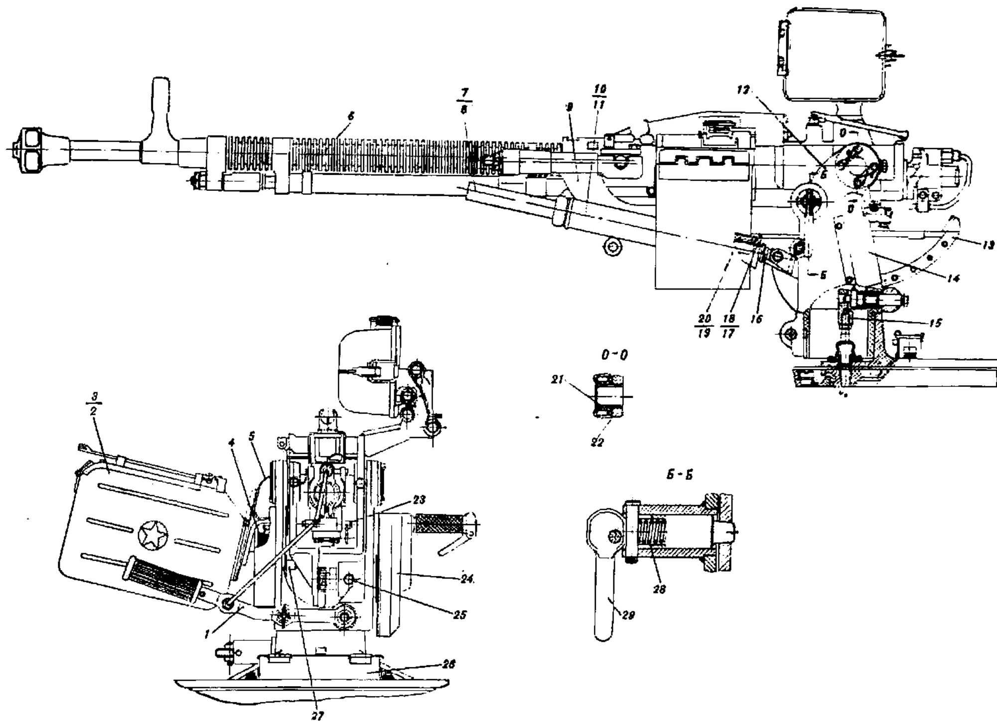
Рис. 112. Установка пулемета ДШК-М (155.32сб)
