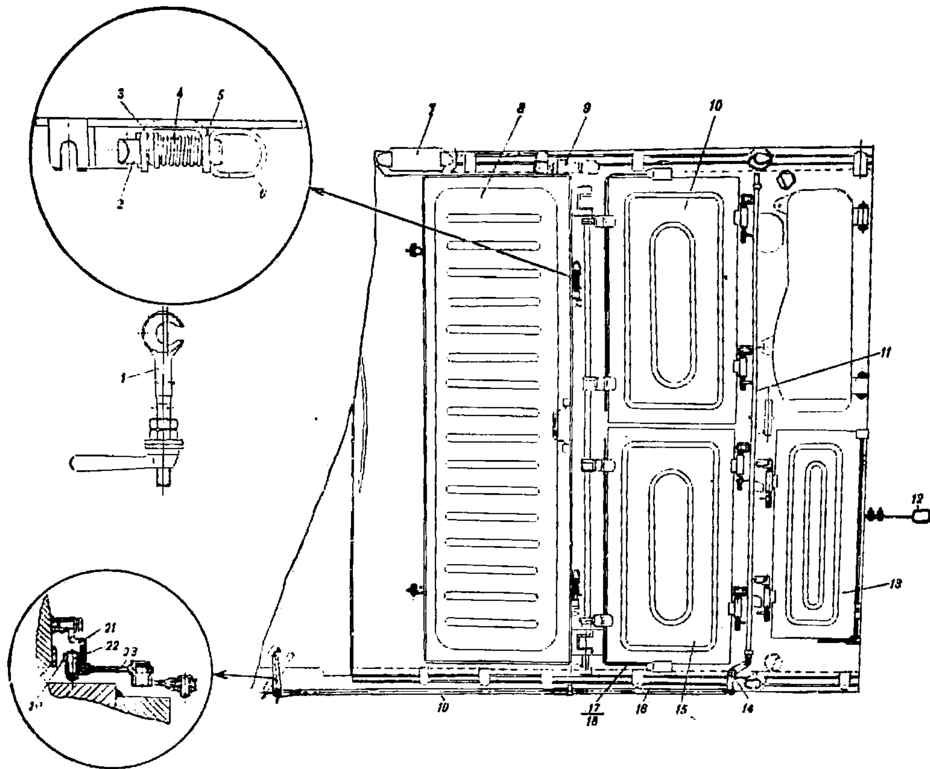
Рис. 89. Установка крышек ОПВТ (166.29.292сб-2)
