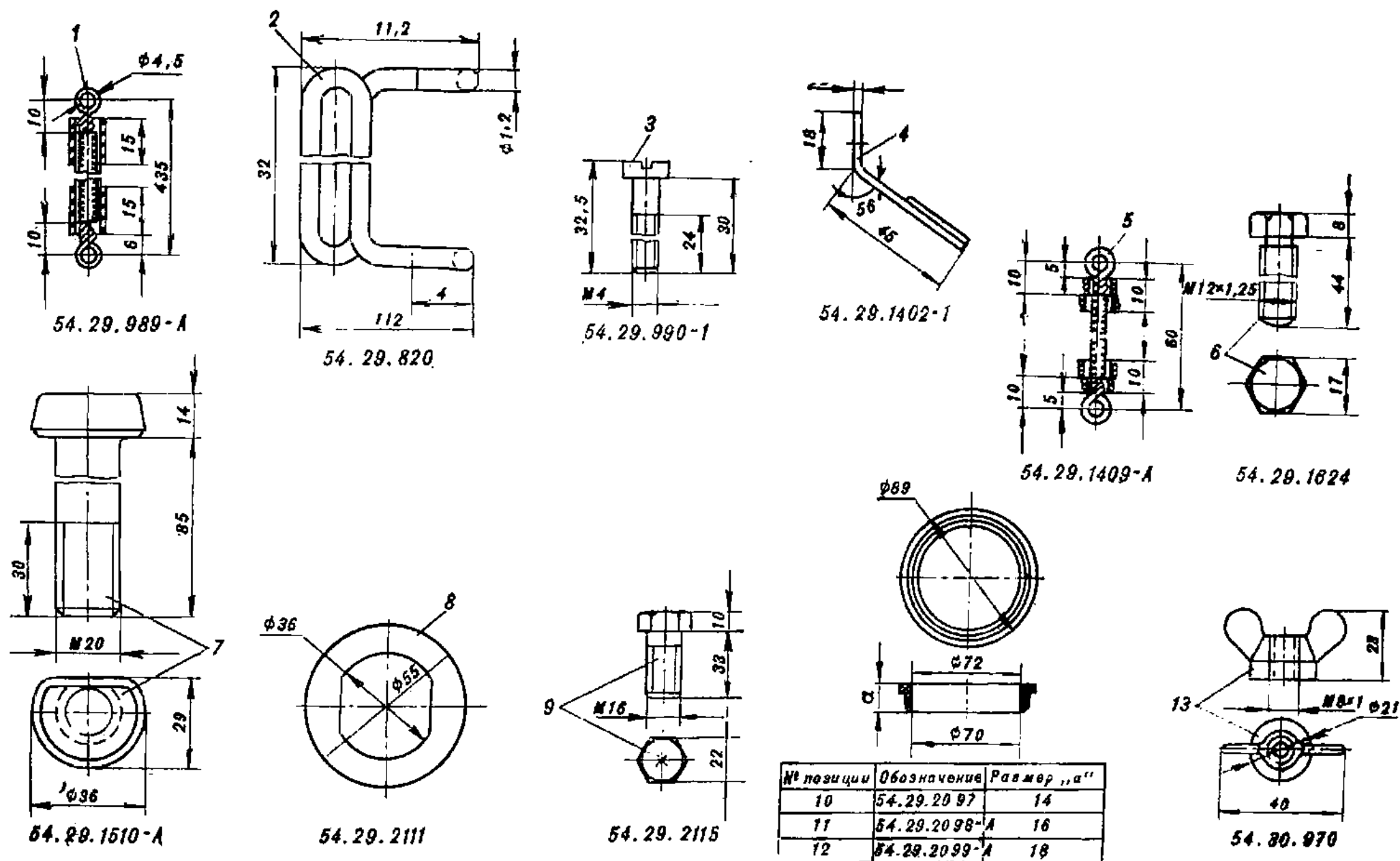
Рис. 94. Детали корпуса
