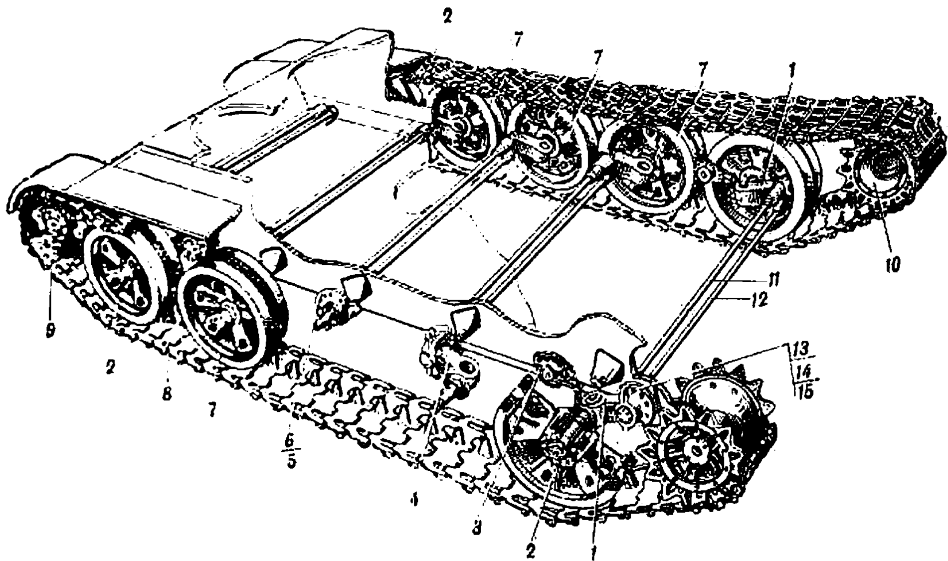
Рис. 31. Узлы ходовой части
