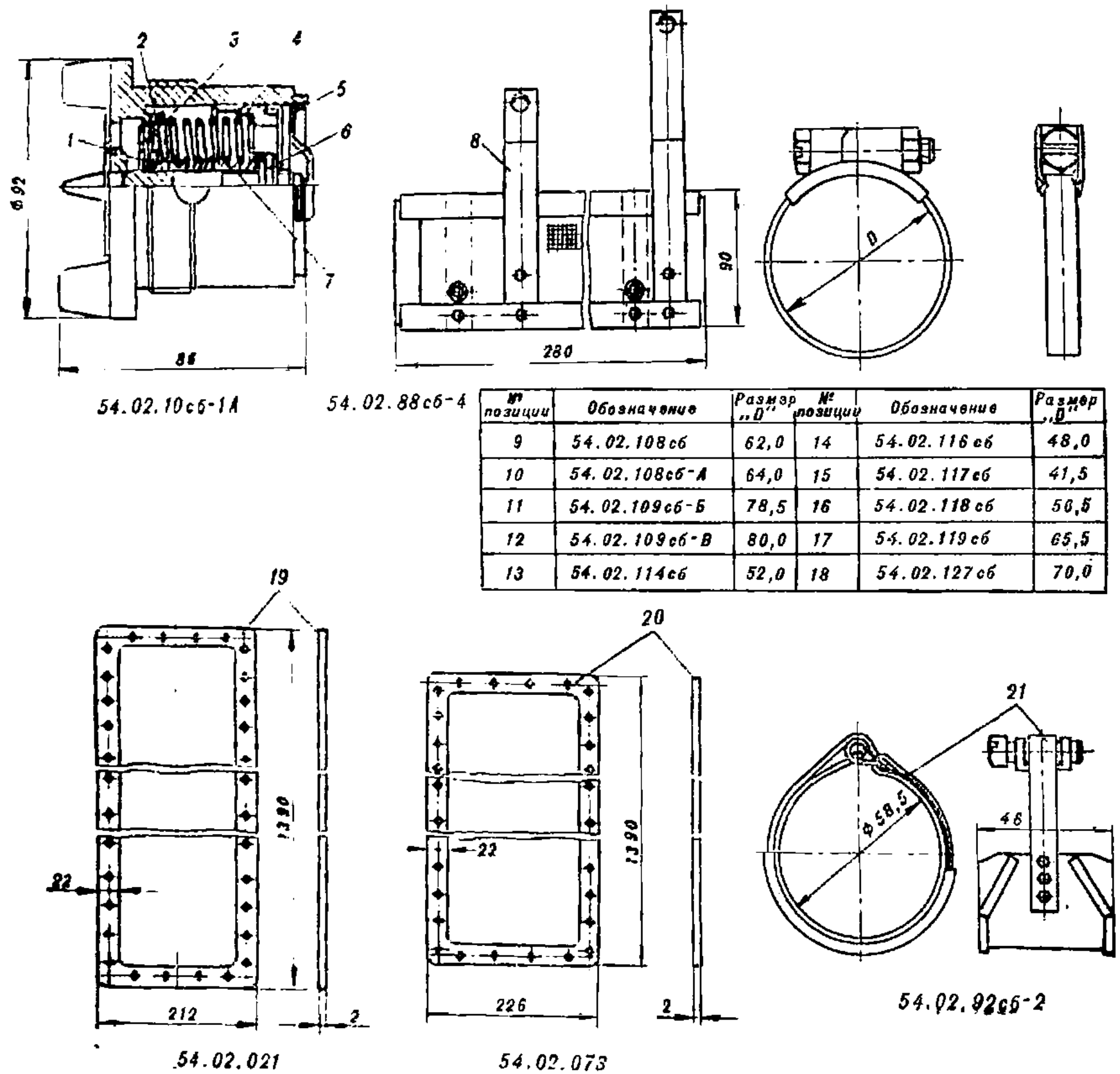
Рис. 4. Детали системы охлаждения
