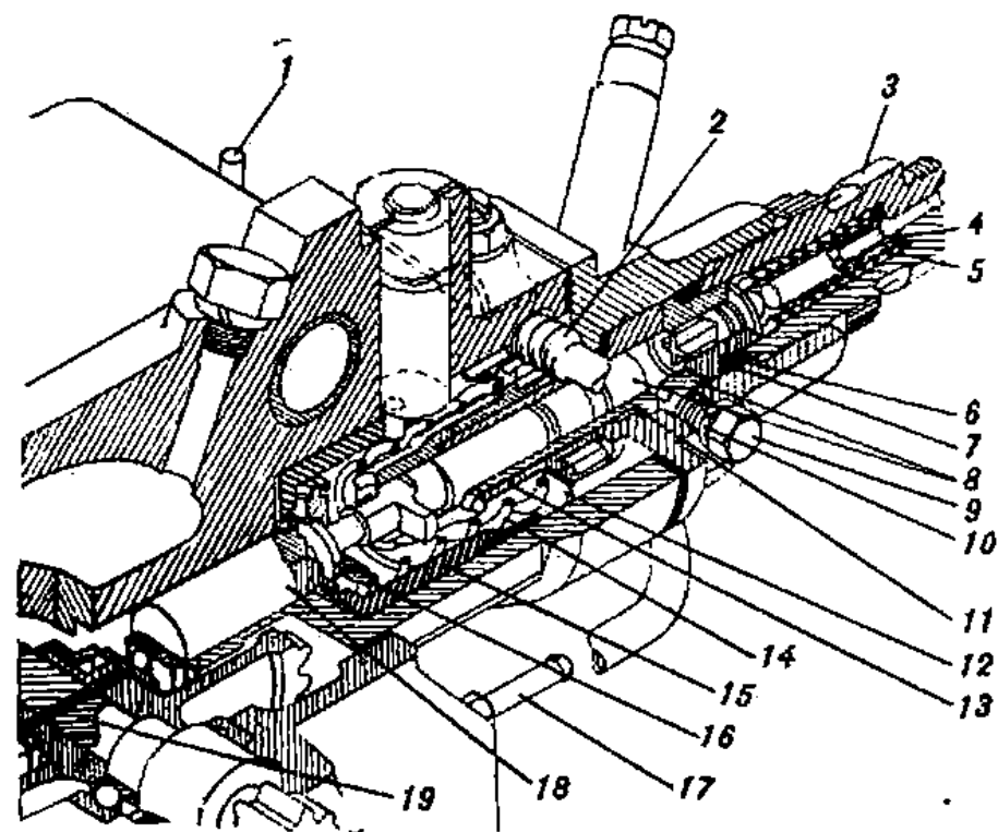
Рис. 145. Узел топливного насоса подогревателя
