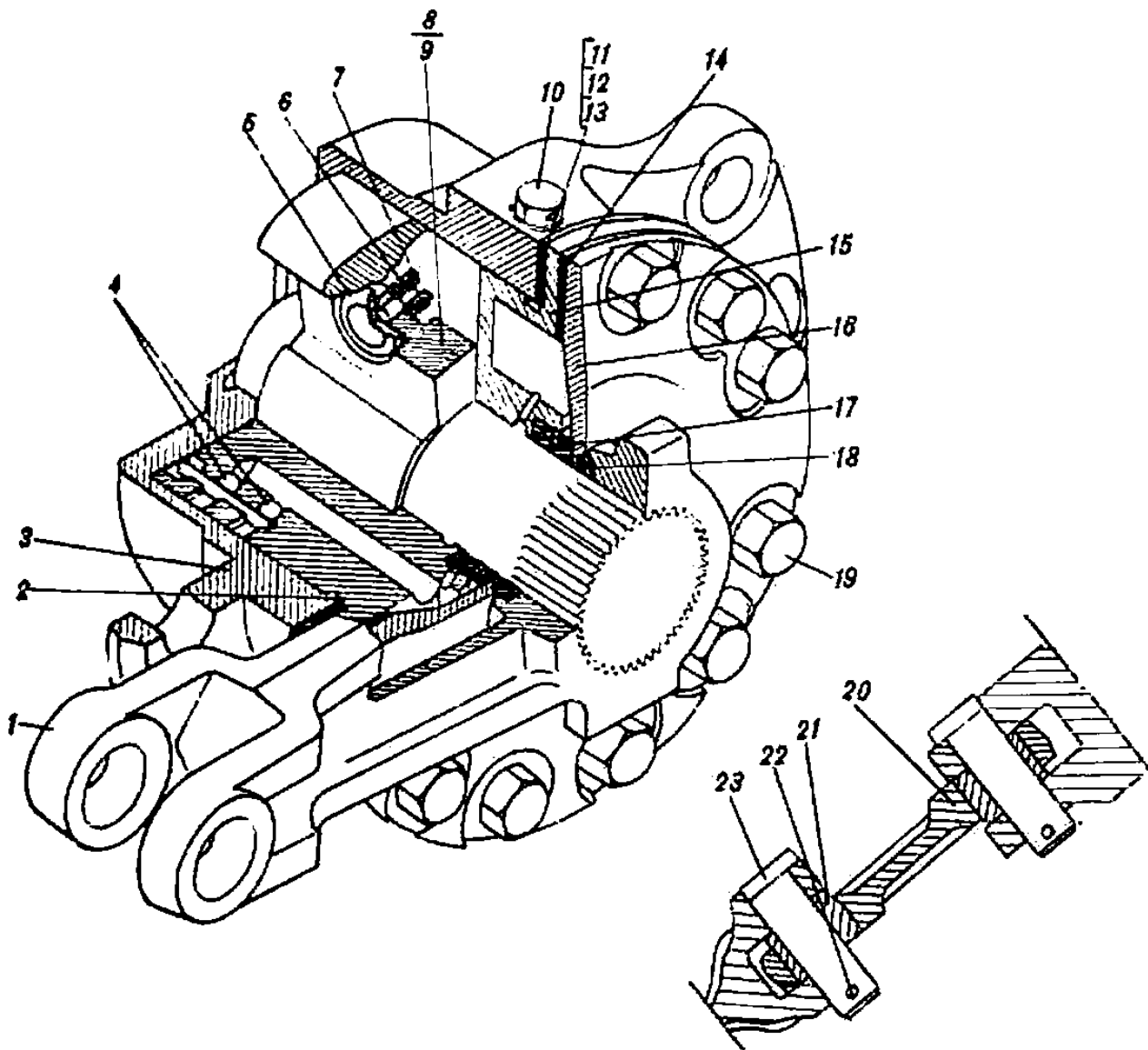
Рис. 34. Гидравлический амортизатор (54.14.4сб-4Б для 1-го правого и 5-го левого катков и 54.14.5сб-4Б для 1-го левого и 5-го правого катков)
