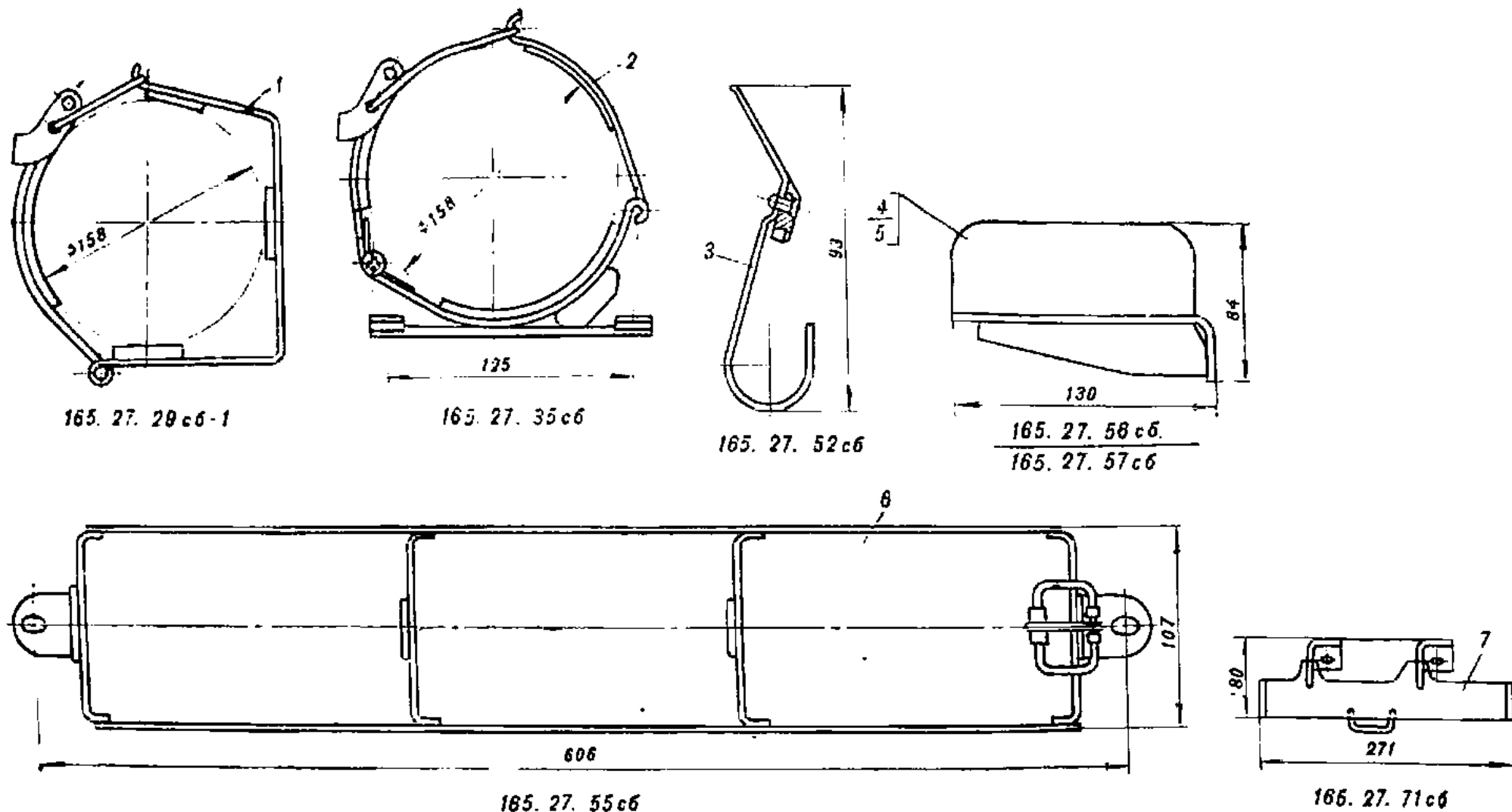
Рис. 72. Узлы укладки боекомплекта
