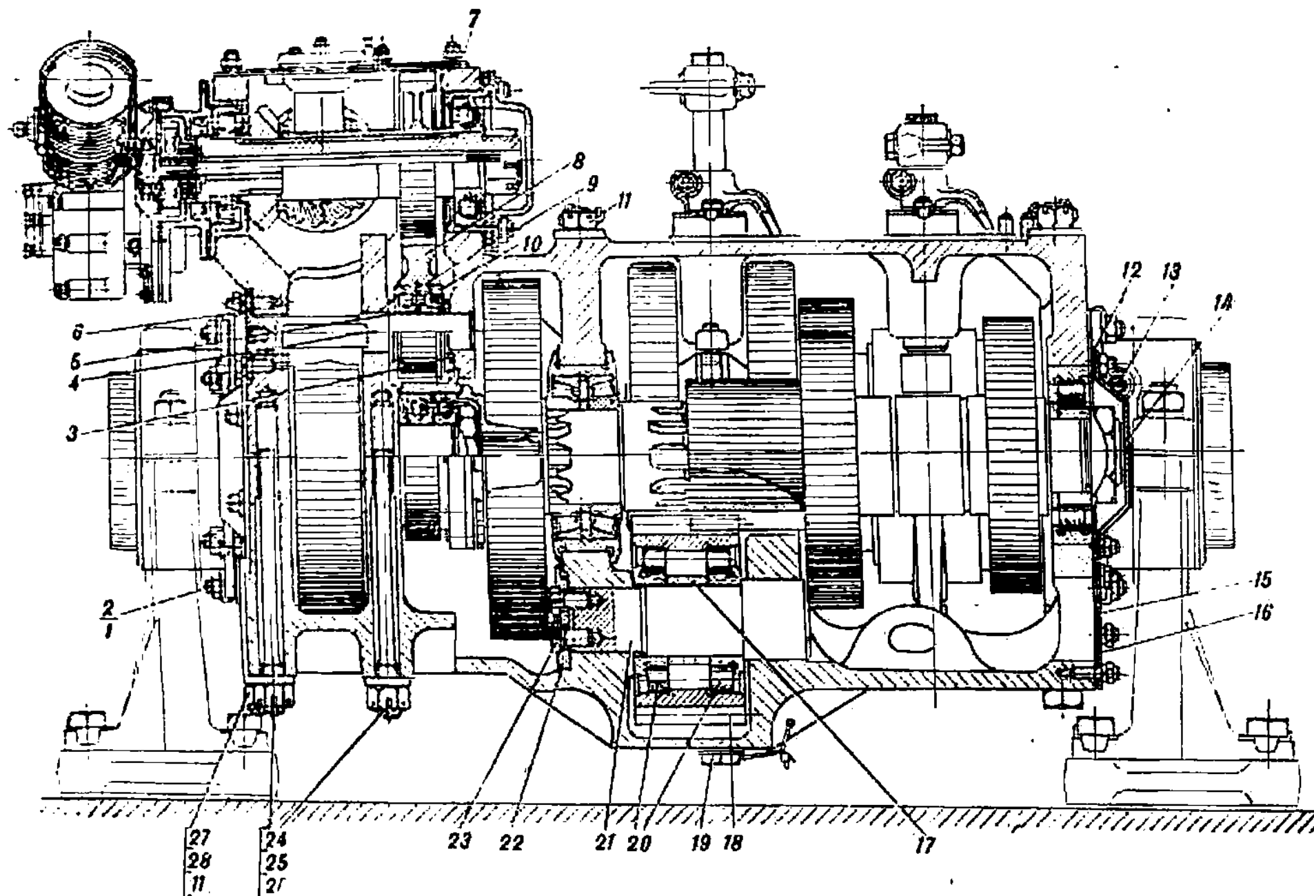
Рис. 19. Коробка передач (разрез по передаточному валу)
