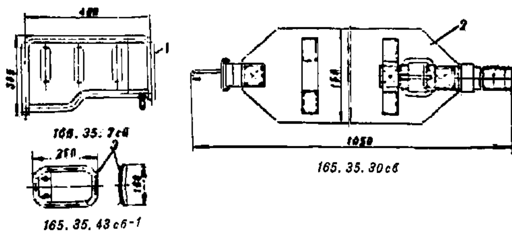
Рис. 126. Узлы установки сидений
