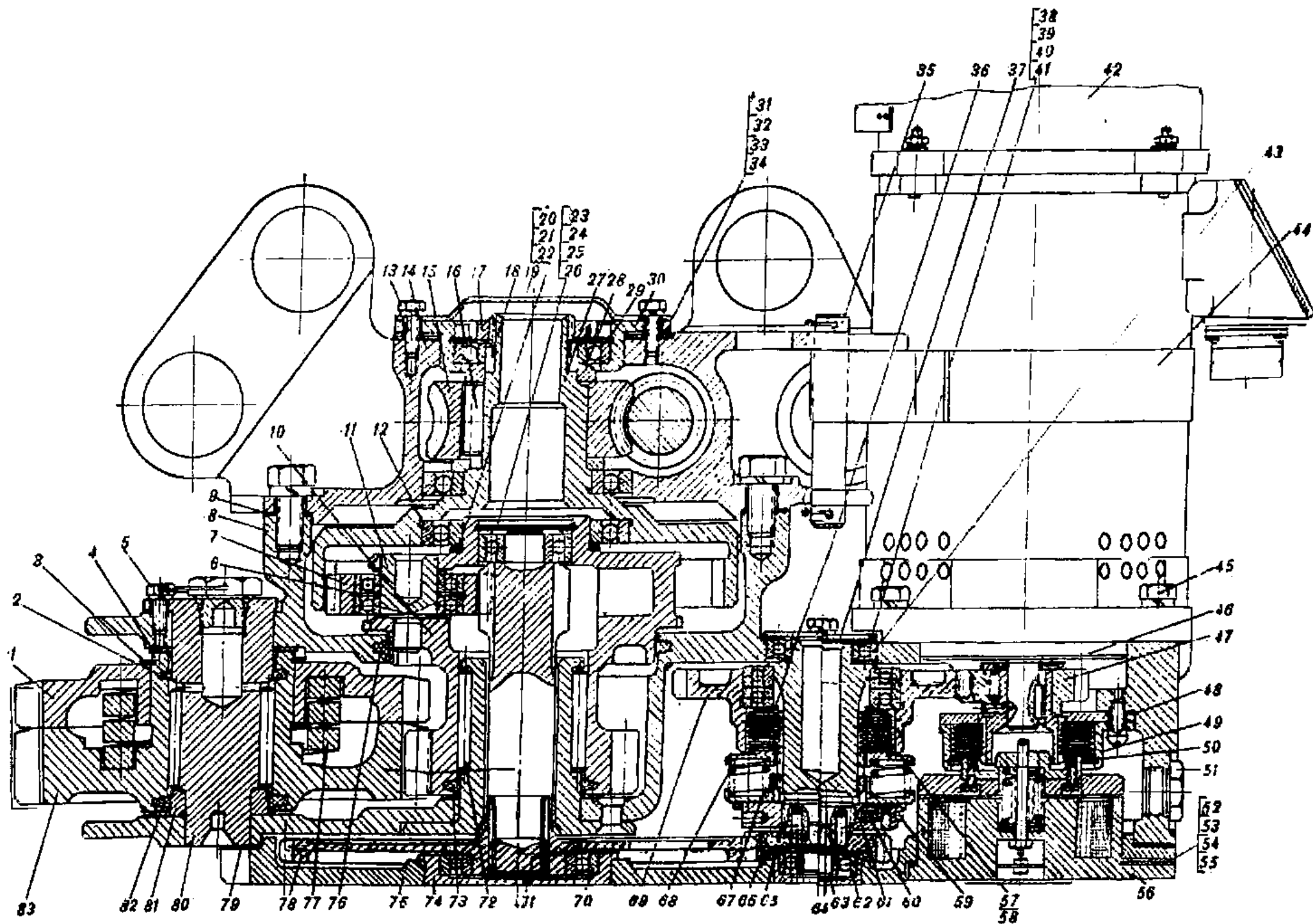
Рис. 121. Поворотный механизм А-А (см. рис. 120)
