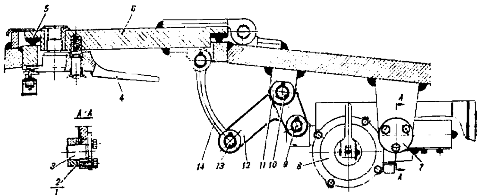
Рис. 43. Установка привода люка выброса гильз (165.17.57сб-1)
