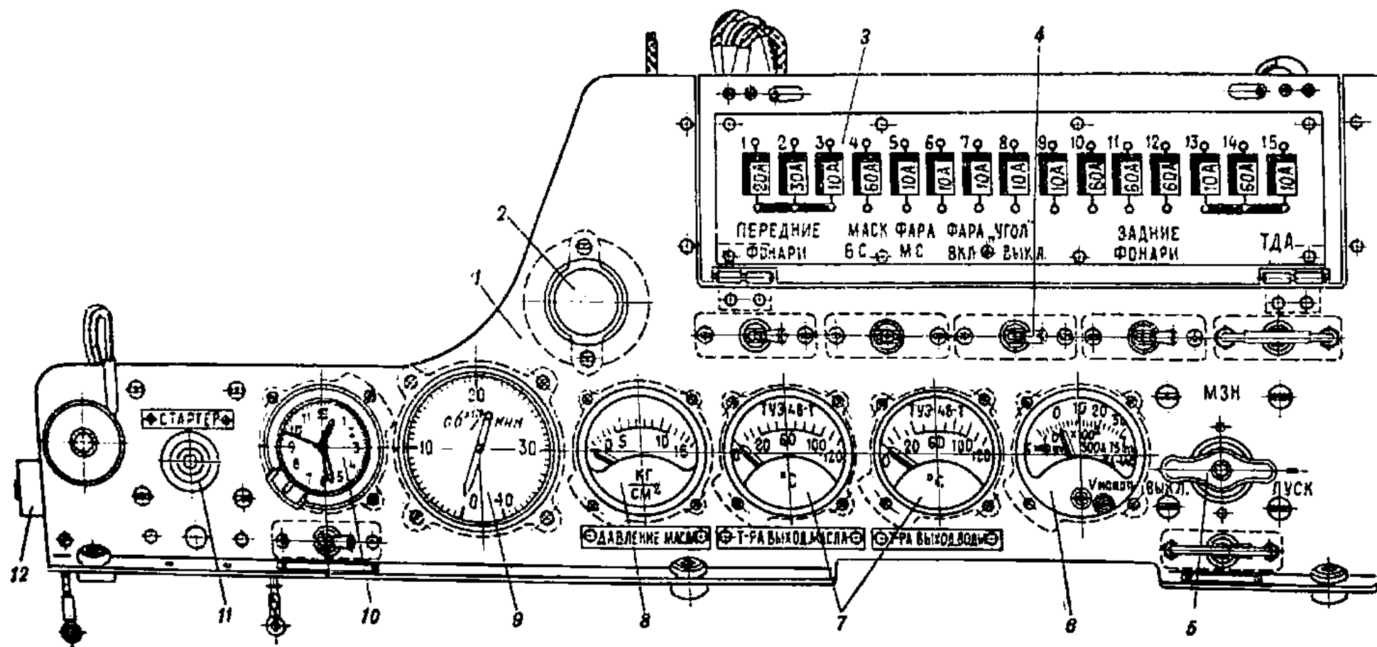
Рис. 60. Щиток приборов водителя (166.26.1сб-2)
