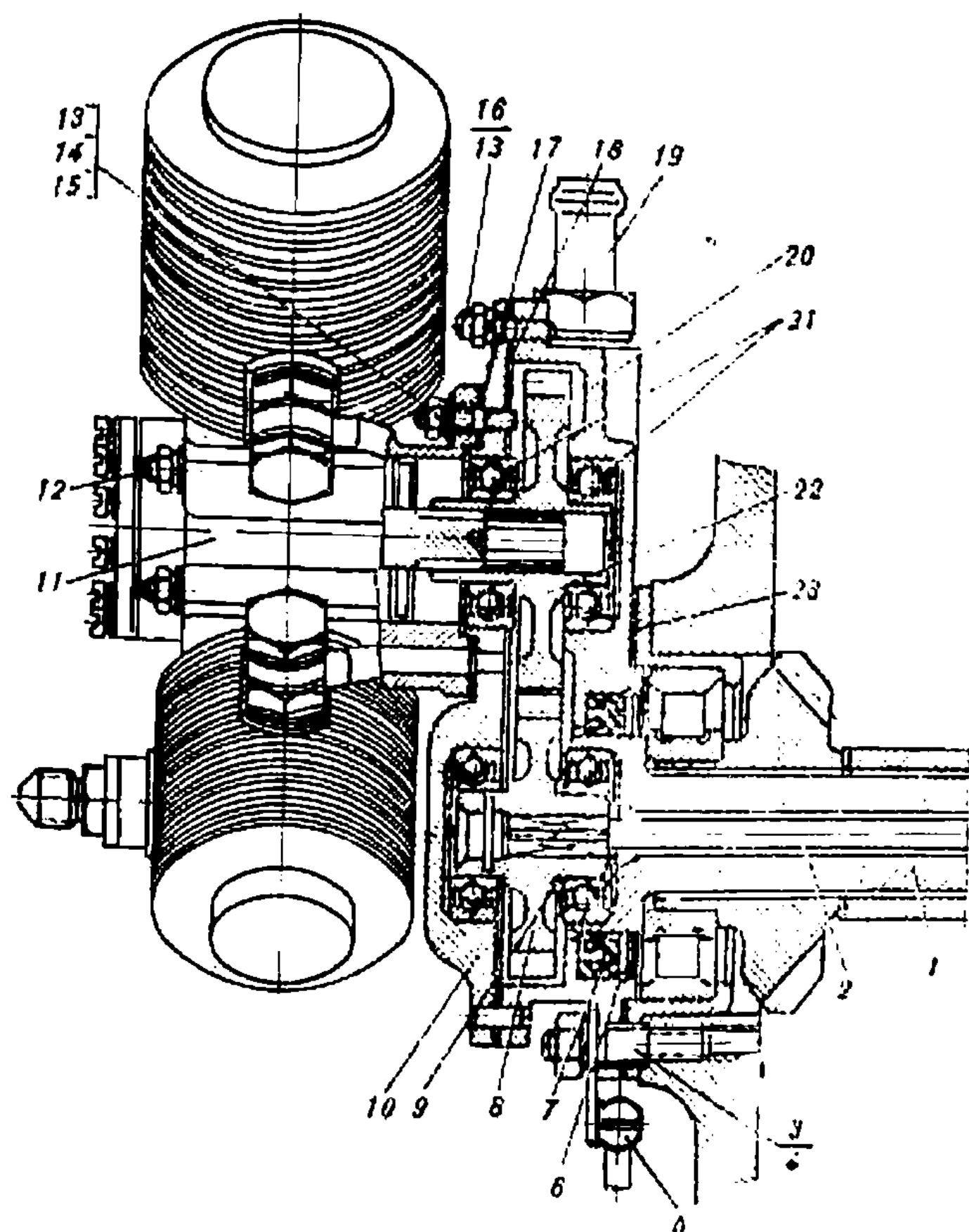
Рис. 20. Привод к компрессору
