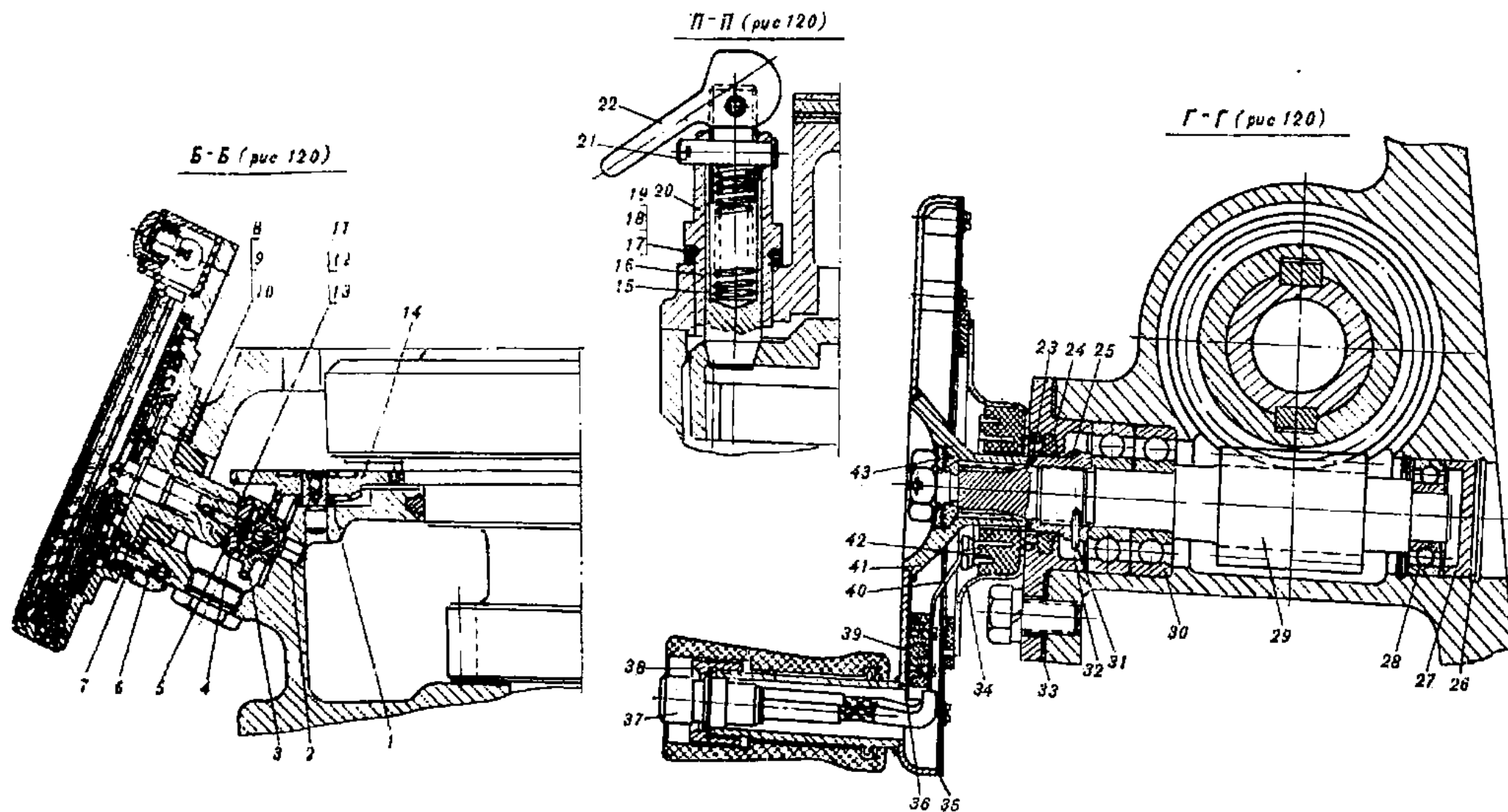
Рис. 122. Узлы поворотного механизма (166.34сб-1)
