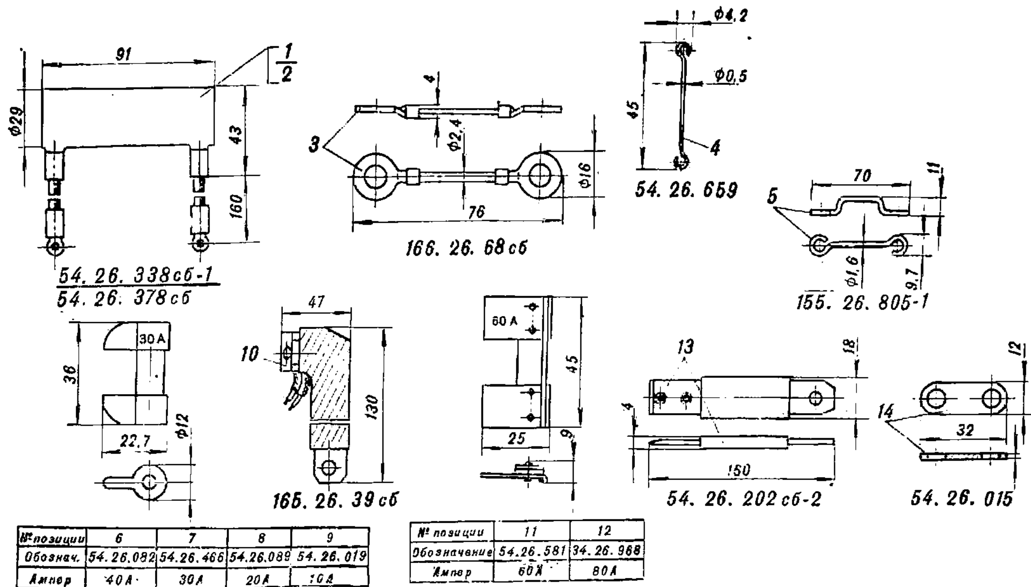
Рис. 65. Резисторы, предохранители, переключки
