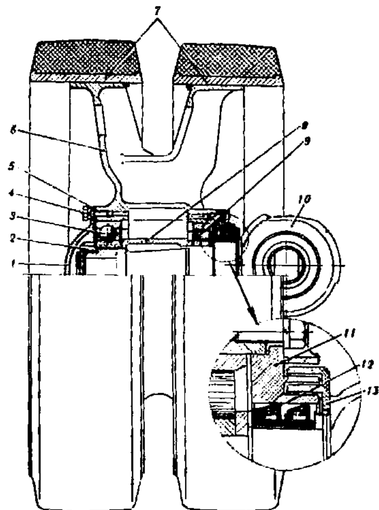
Рис. 33. Подвеска со средним опорным катком (165.12.3сб-А)
