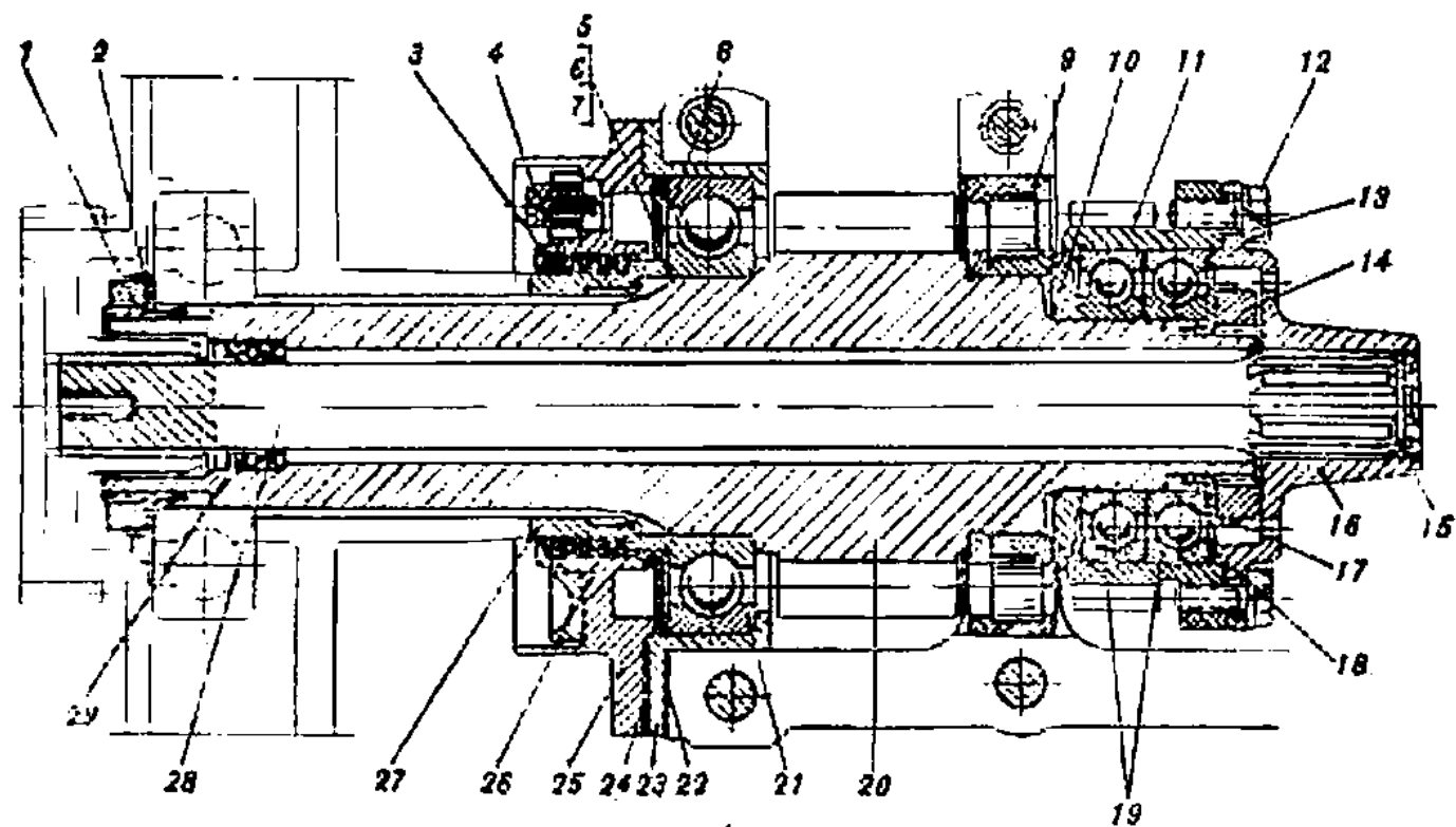
Рис. 22. Вал ведущий
