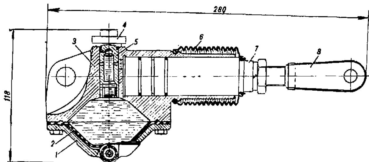
Рис. 51. Бустер (155.21.15сб)
