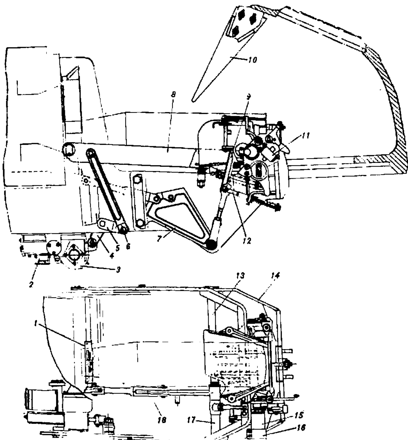
Рис. 39. Механизм выброса гильз (165.17.1сб-2)
