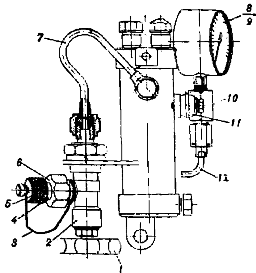
Рис. 134. Отстойник с манометром (155.38.133сб)
