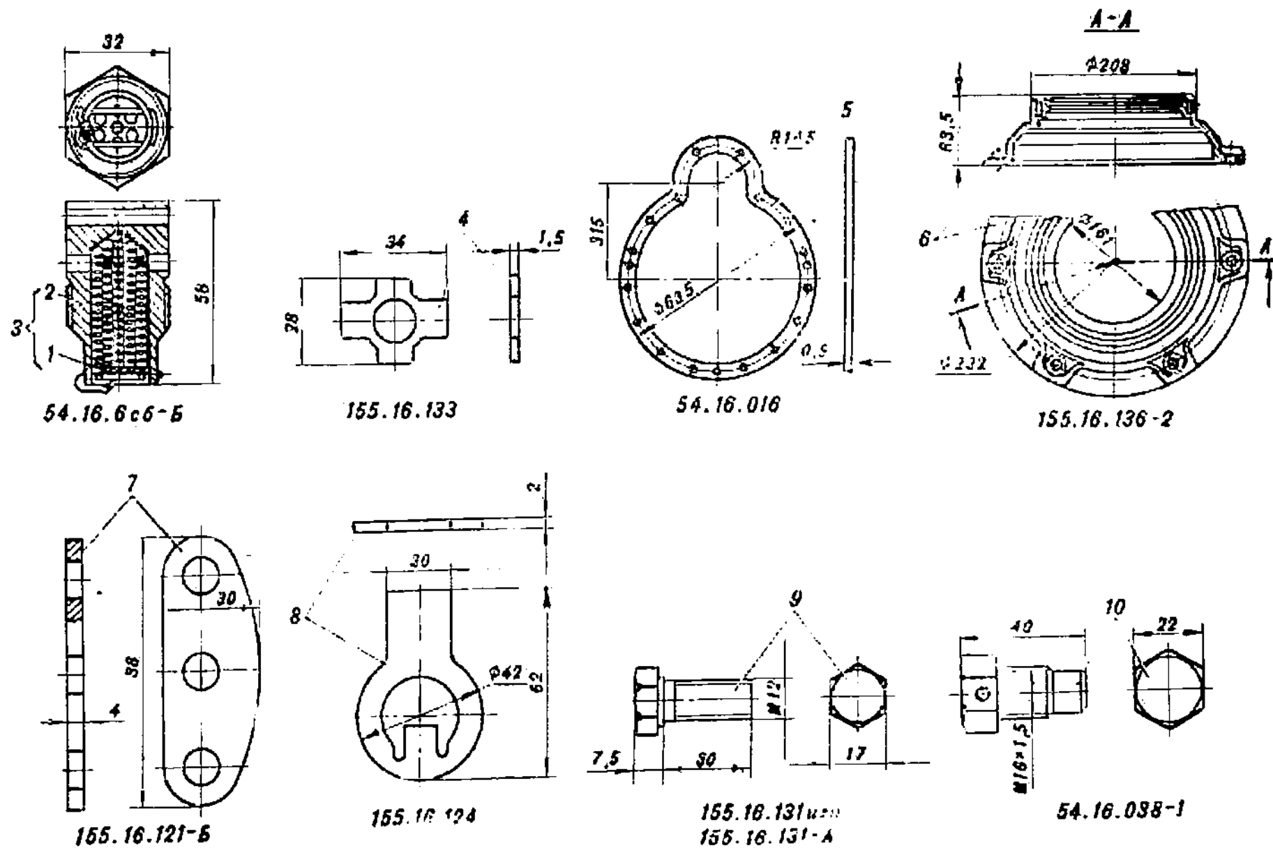
Рис. 38. Детали бортовой передачи
