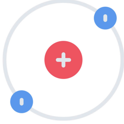
Protons
