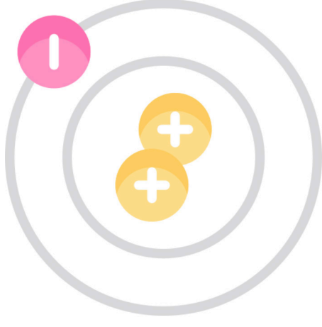
Ion
