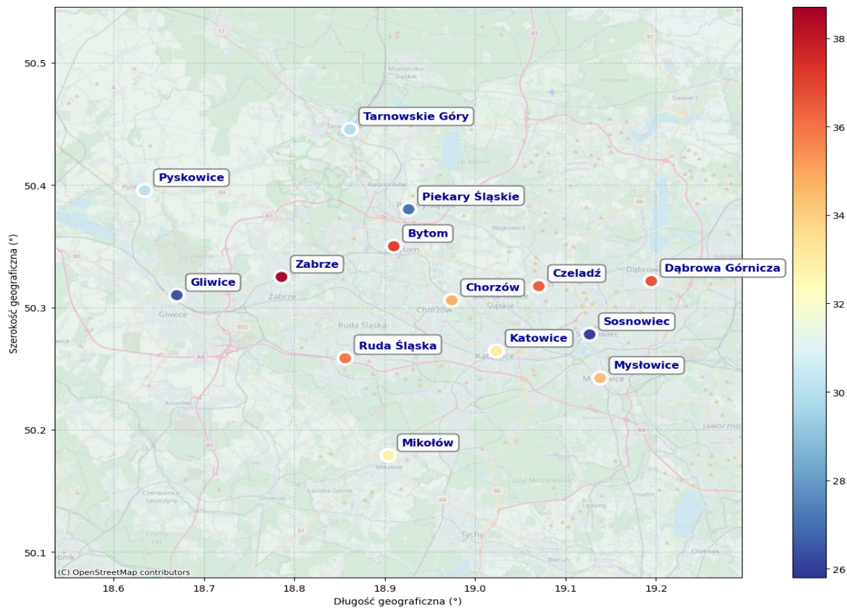
Mapa punktów pomiarowych - PM25 (2025-01-03)
