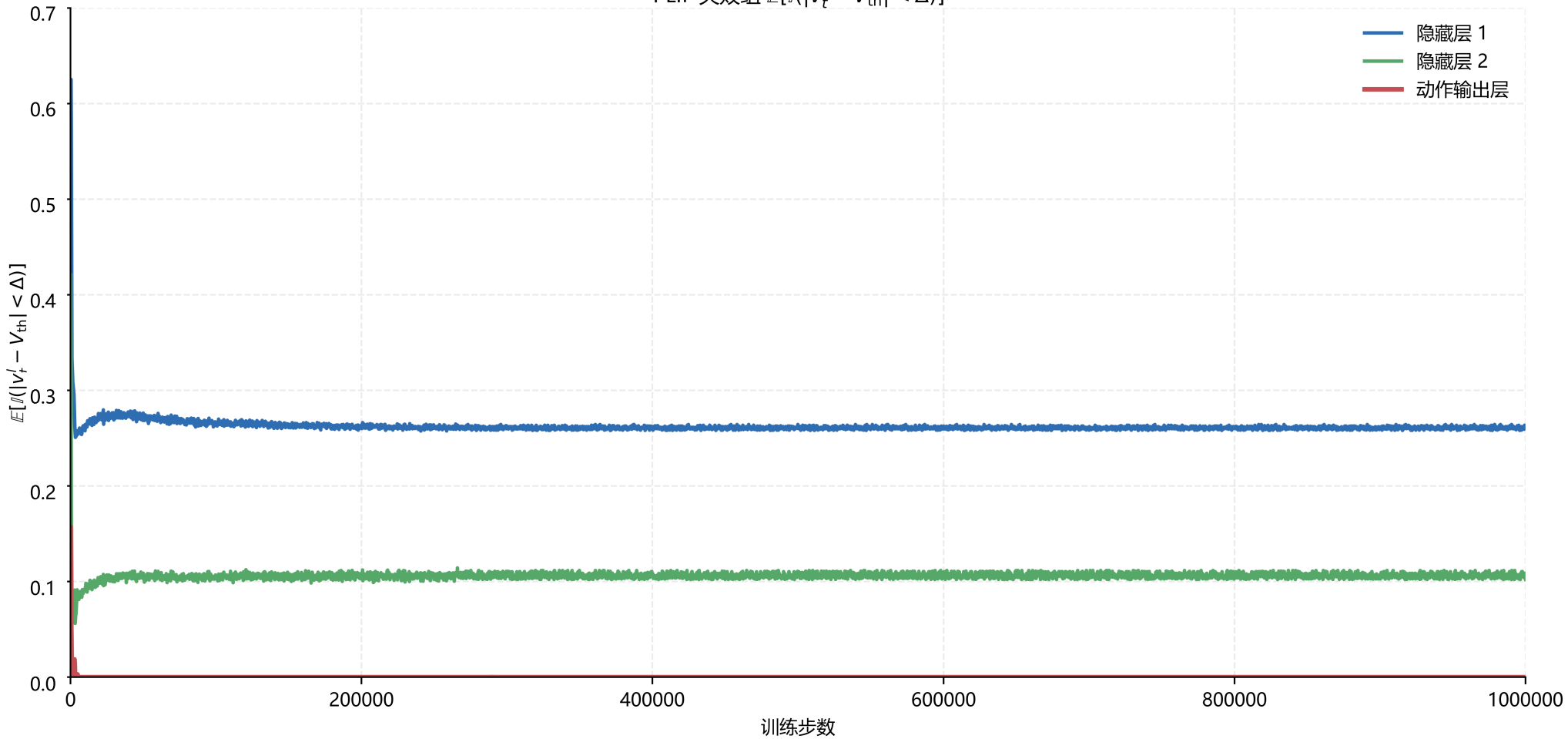
PLIF 失败组 E[\mathbb{I}(|v_t^l - V_{th}| < \Delta)]
