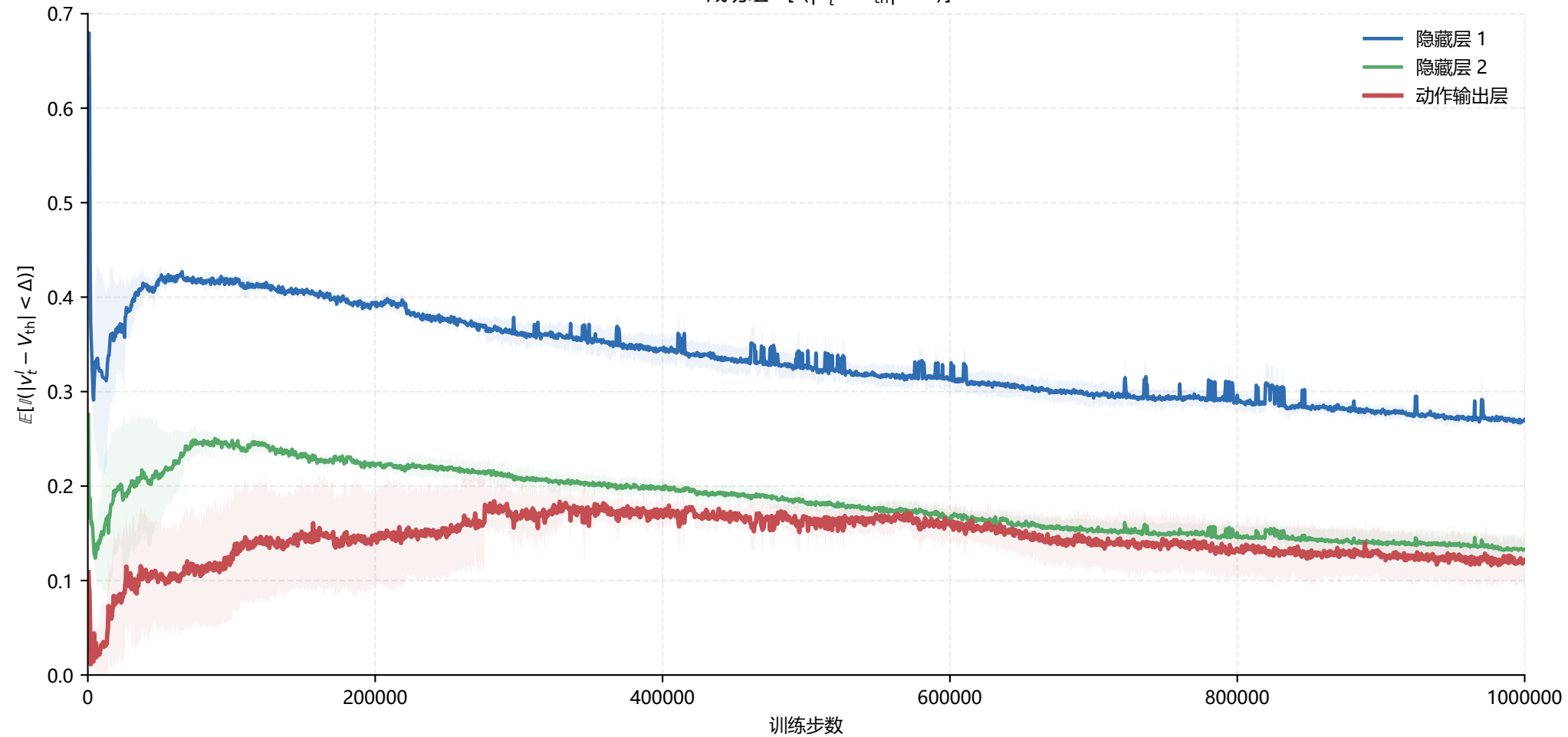
PLIF 成功组 \mathbb{E}[\mathbb{I}(|v_t^l - V_{th}| < \Delta)]
