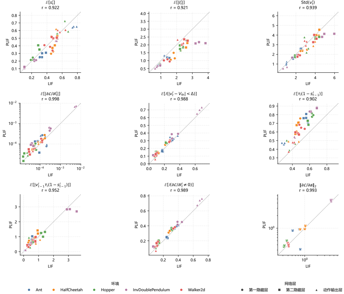
图 5-9 成功训练组中 LIF 与 PLIF 的配对机制诊断指标对比。每个点对应一个环境、随机种子和网络层在训练后期的平均值，虚线表示 y = x 。较高的配对相关性说明二者在放电状态、膜电位尺度、代理梯度窗口占比和反向梯度通道上具有相近的训练机制。
