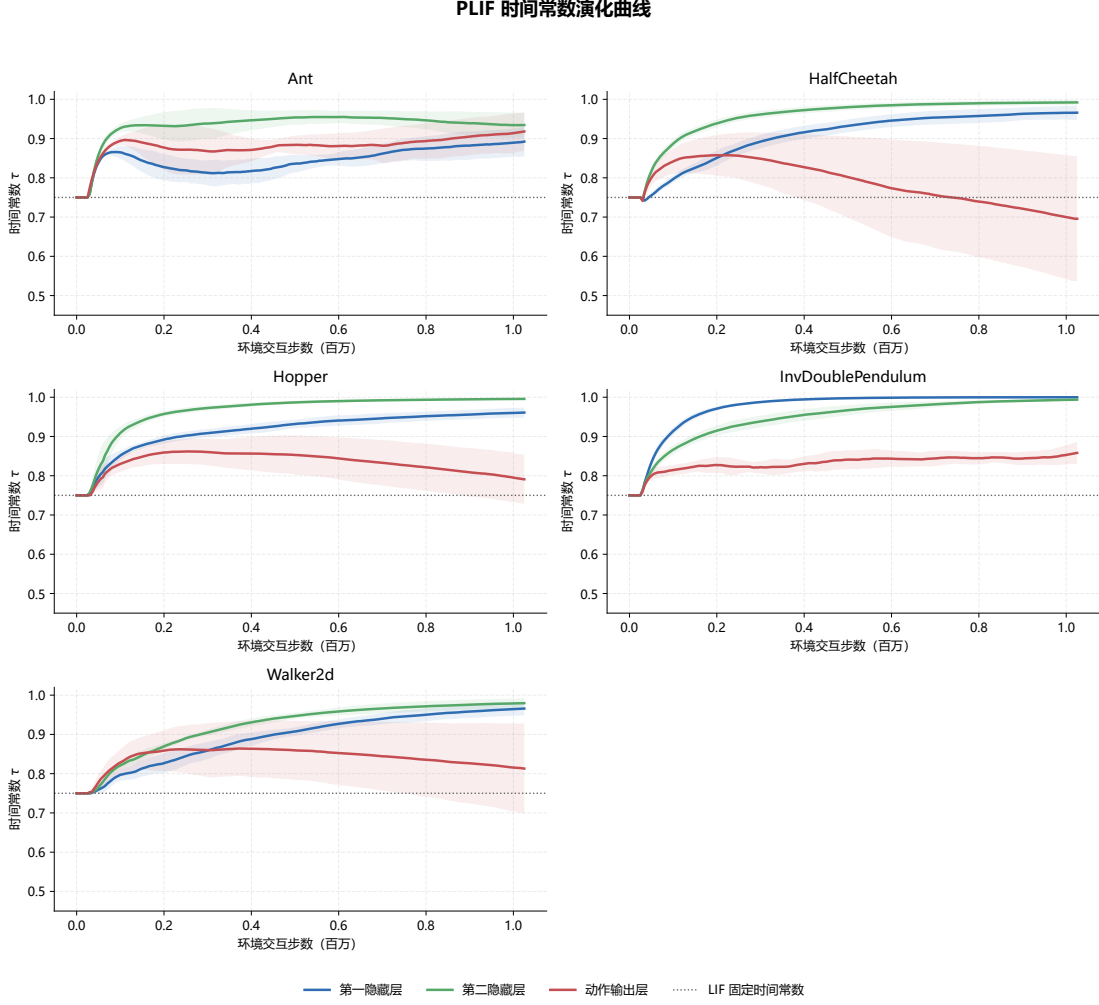
图 5-8 常规 PT-PLIF 实验中不同环境的 PLIF 时间常数演化曲线。蓝色和绿色分别表示两层隐藏层 PLIF 神经元模块，红色表示动作输出层，灰色虚线表示与 LIF 对齐的固定初始值 0.75。
