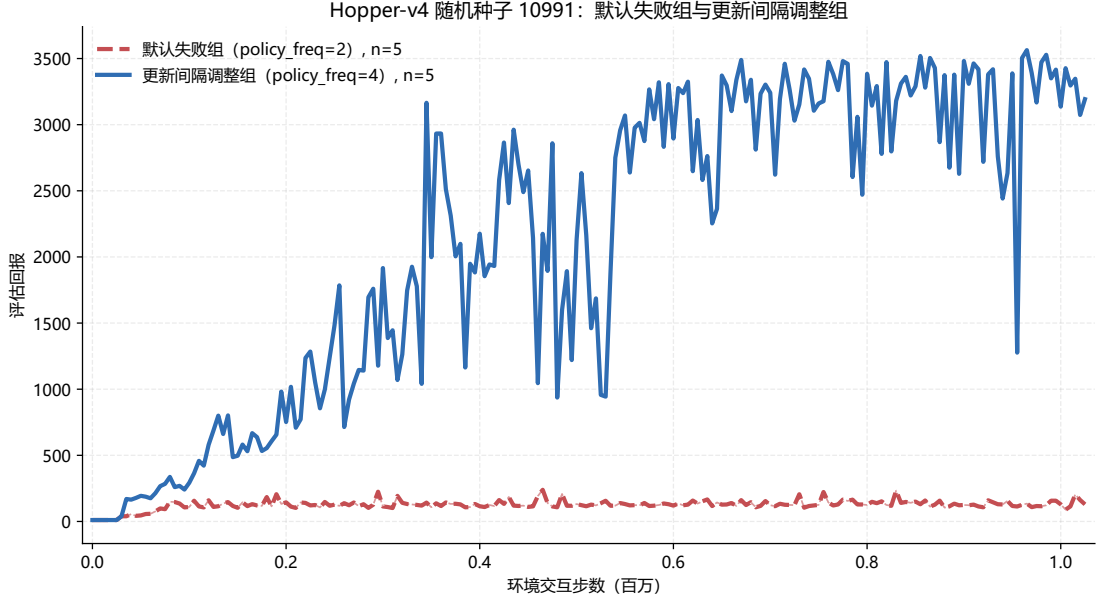
图 4-3 Hopper-v4 随机种子 10991 下默认失败组与 policy_freq 调整组的重复运行学习曲线
