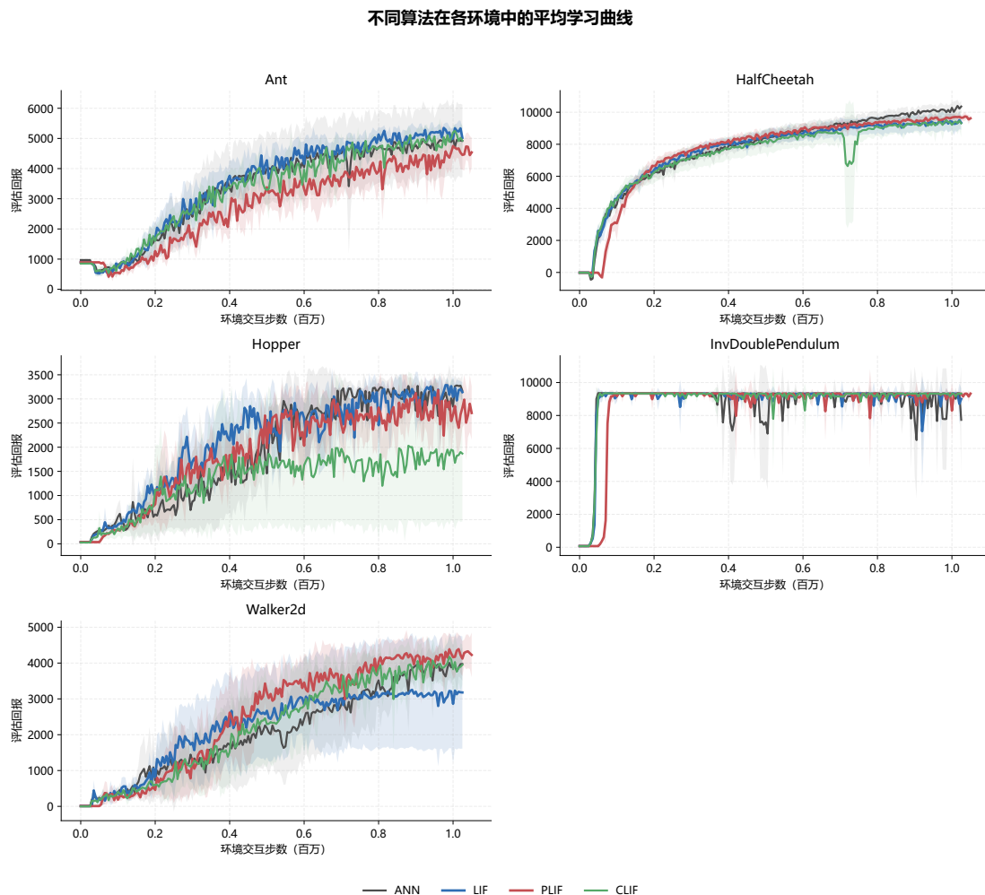
图 4-2 不同算法在五个 MuJoCo 环境中的学习曲线对比
