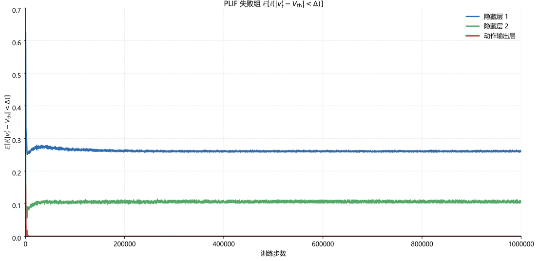
图 4-6 Hopper-v4 默认失败组的代理梯度窗口占比。纵轴为 \mathbb{E}[\mathbb{I}(|v_t^l - V_{th}| < \Delta)] ，表示各层膜电位落入代理梯度有效窗口的比例。
