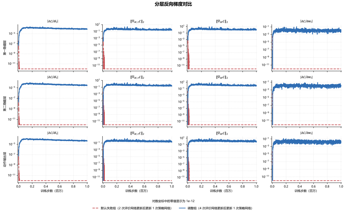
图 4-4 Hopper-v4 随机种子 10991 下默认失败组与 actor 更新间隔调整组的分层 STBP 梯度对比。每条曲线先对 5 个脉冲时间步聚合，再对 5 次重复运行取平均；对数坐标中精确零值以 10^{-12} 显示。
