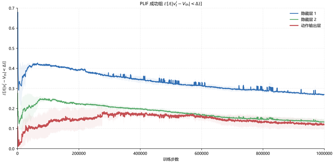
图 4-7 Hopper-v4 actor 更新间隔调整成功组的代理梯度窗口占比。与默认失败组相比，成功组在隐藏层和动作输出层均能长期保留非零代理梯度窗口占比。
