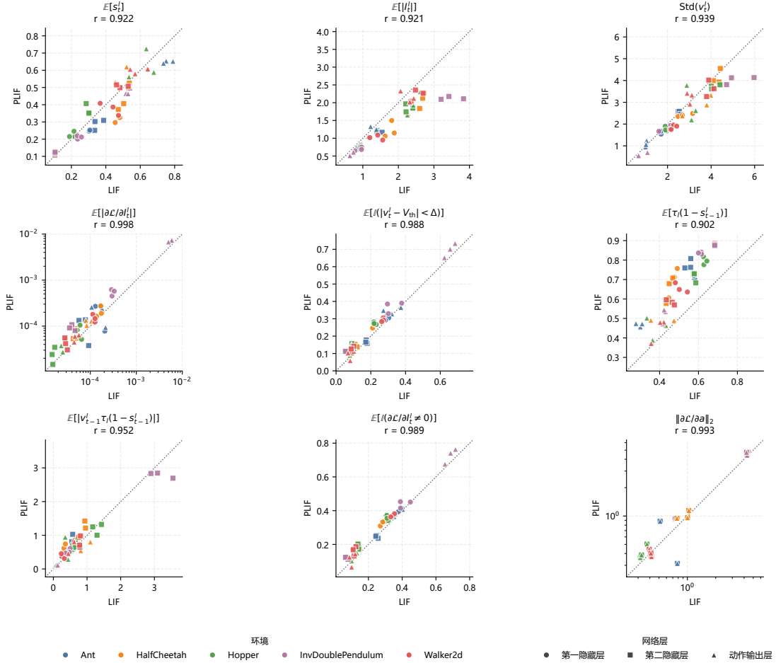
图 4-9 成功训练组中 LIF 与 PLIF 的配对机制诊断指标对比。每个点对应一个环境、随机种子和网络层在训练后期的平均值，虚线表示 y = x 。较高的配对相关性说明二者在放电状态、膜电位尺度、代理梯度窗口占比和反向梯度通道上具有相近的训练机制。
