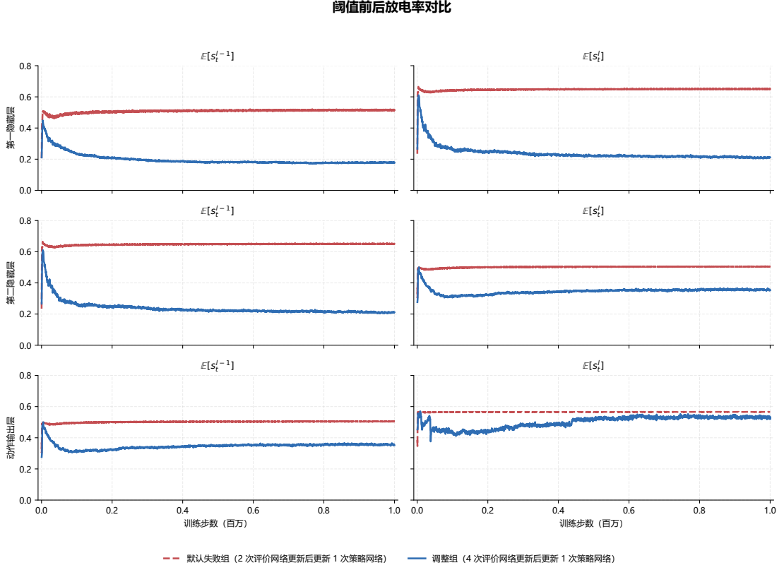
图 4-5 Hopper-v4 随机种子 10991 下默认失败组与 actor 更新间隔调整组的阈值前放电率与阈值后放电率对比。失败组后期仍保持较高阈值后放电率，说明低回报停滞不是由脉冲沉默直接造成。
