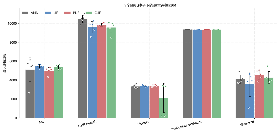
图 4-1 不同算法在五个 MuJoCo 环境中的最大评估回报对比
