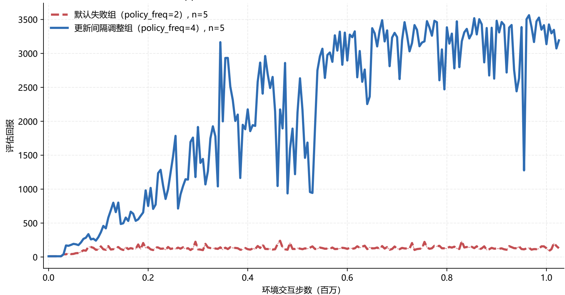
Hopper-v4 随机种子 10991：默认失败组与更新间隔调整组
