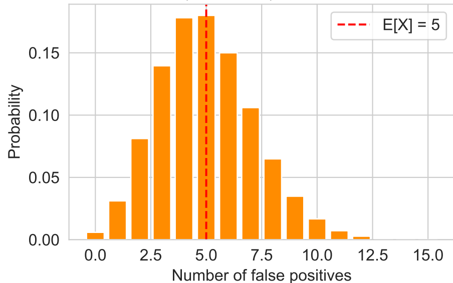
Binomial(100, 0.05): False Positives
