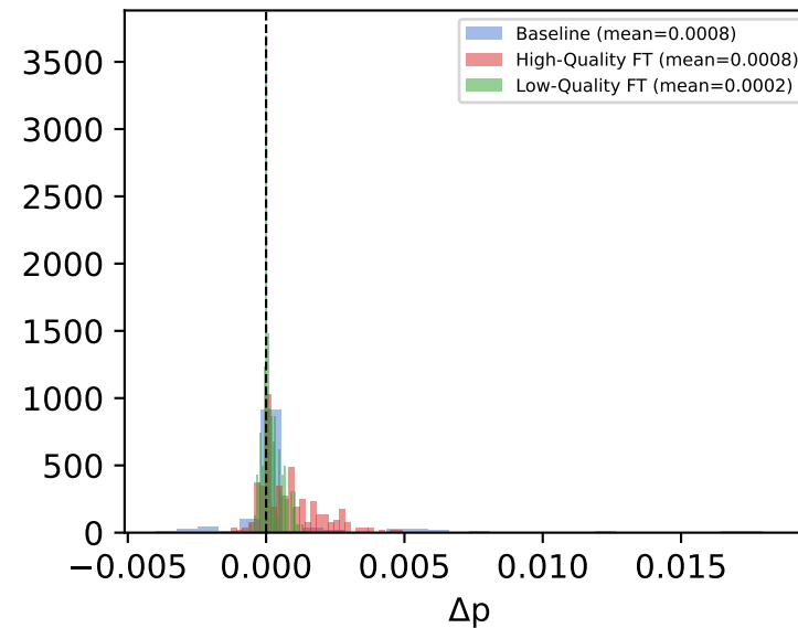
Mistral-7B
