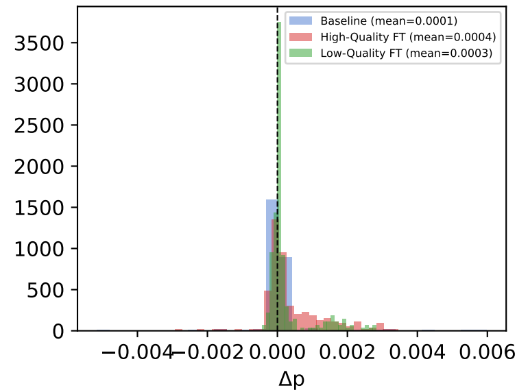
LLaMA-3-8B
