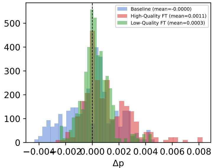
Phi-3
