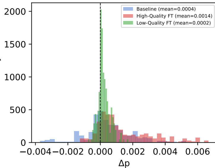
LLaMA-3-3B
