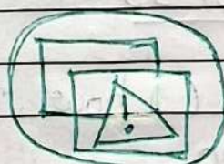
Adware
