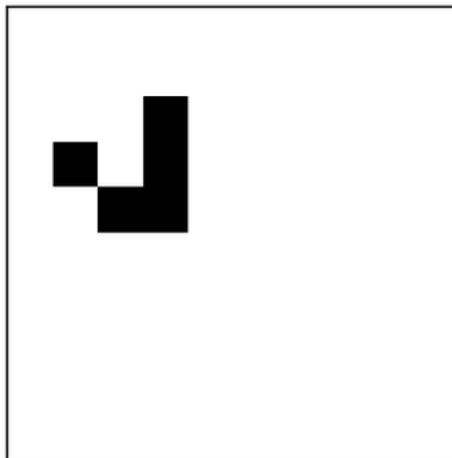
Игра «Жизнь» Конвея: движение планера (glider)
