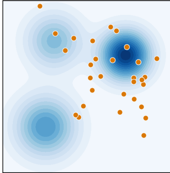
промежуточная стадия
