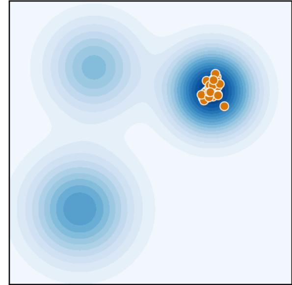
сходимость роя
