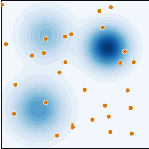
начальное распределение
