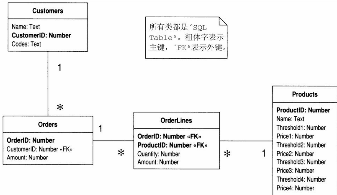
图12-8 订单程序所用的数据库
