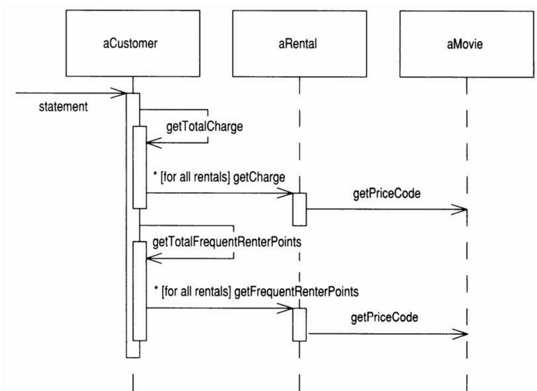
图1-11 “总量计算”函数被提炼后的序列图
