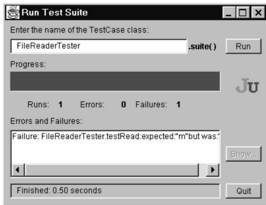
图4-2 JUnit的图形用户界面
