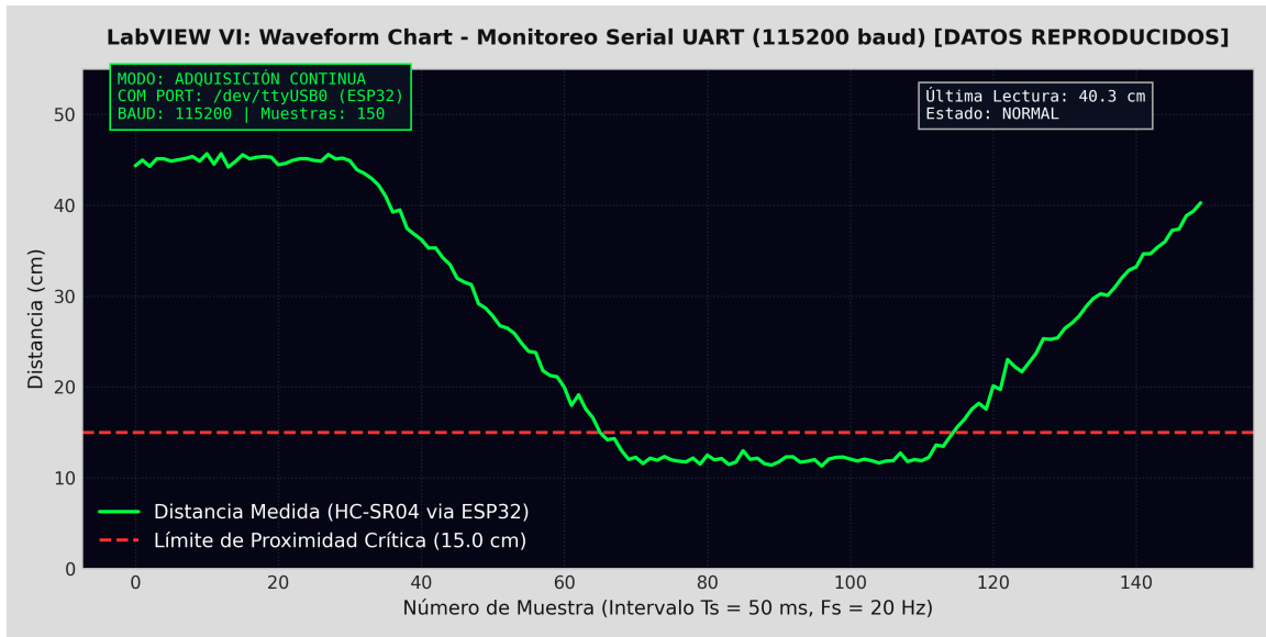
Figura 5: Emulación del Panel Frontal del Instrumento Virtual en LabVIEW: monitoreo continuo de distancia a 115200 baudios con límite de proximidad fijado en 15.0 cm.
