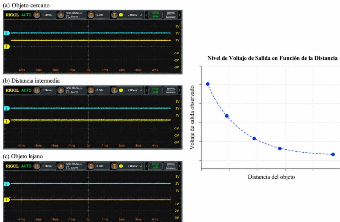
Figura 4: Señal observada en el osciloscopio durante la caracterización del sensor ultrasónico. La respuesta presenta un nivel de voltaje aproximadamente constante, acompañado de pequeñas variaciones de ruido. Al modificar la distancia del objeto frente al sensor, se observó un cambio en el nivel de voltaje de la señal.
