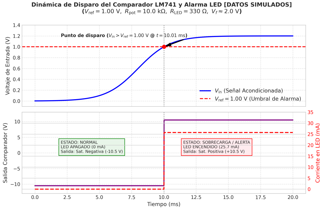
Figura 3: Dinámica de conmutación del comparador LM741 y polarización del LED indicador ante cruce de umbral ( V_{ref} = 1.00 \text{ V} , V_{in} = 1.20 \text{ V} , R_{pot} = 10.0 \text{ k}\Omega , R_{LED} = 330 \Omega , V_f \approx 2.0 \text{ V} , I_{LED} \approx 25.7 \text{ mA} ).
