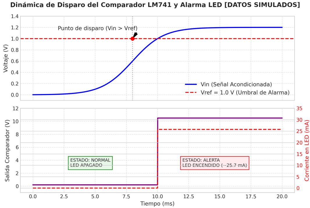
Figura 3: Dinámica de conmutación del comparador LM741 y polarización del LED indicador ante cruce de umbral ( V_{ref} = 1.00\text{ V} , V_{in} = 1.20\text{ V} , R_{LED} = 330\ \Omega , I_{LED} \approx 25.7\text{ mA} ).
