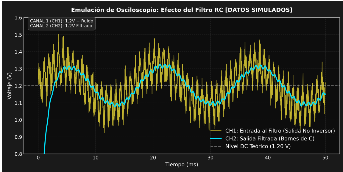
Figura 2: Emulación de osciloscopio de dos canales: señal de entrada con rizado y ruido antes del filtro (CH1, amarillo) vs. señal atenuada y suavizada en borres del capacitor (CH2, cian)
