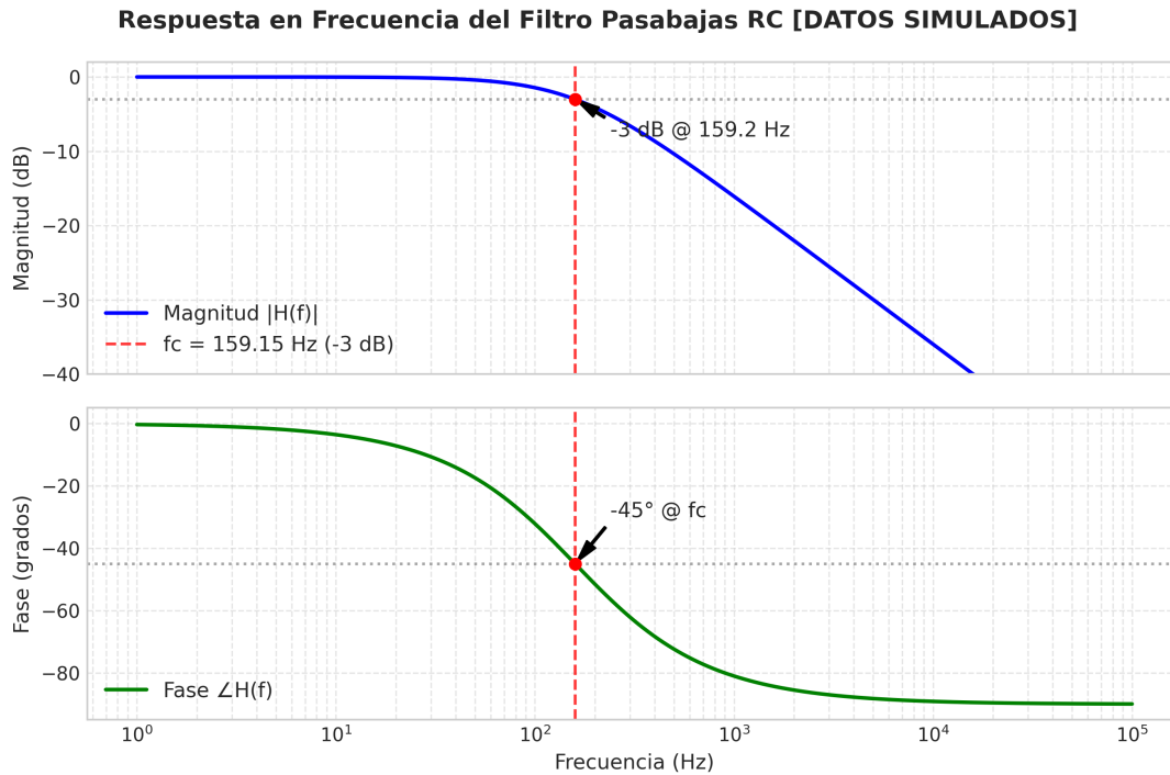
Figura 1: Respuesta en frecuencia del filtro pasabajas pasivo RC obtenida mediante simulación numérica ( R = 10.0 k \Omega , C = 100 nF, f_c = 159.15 Hz, \tau = 1.0 ms).
