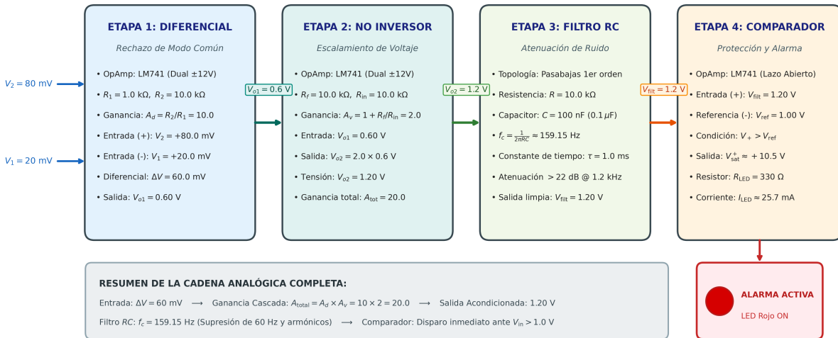
Figura 1: Diagrama esquemático en bloques de la cadena analógica de acondicionamiento, filtrado pasivo y protección por comparador ( R_1 = 1.0 \text{ k}\Omega , R_2 = 10.0 \text{ k}\Omega , R_f = 10.0 \text{ k}\Omega , R_{in} = 10.0 \text{ k}\Omega , R = 10.0 \text{ k}\Omega , C = 100 \text{ nF} , R_{LED} = 330 \Omega , V_{ref} = 1.00 \text{ V} ).
