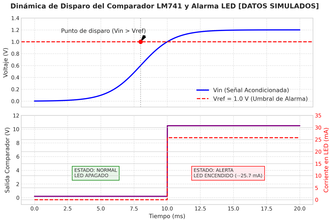
Figura 4: Dinámica de conmutación del comparador LM741 y polarización del LED indicador ante cruce de umbral ( V_{ref} = 1.00 \text{ V} , V_{in} = 1.20 \text{ V} , R_{pot} = 10.0 \text{ k}\Omega , R_{LED} = 330 \Omega , V_f \approx 2.0 \text{ V} , I_{LED} \approx 25.7 \text{ mA} ).
