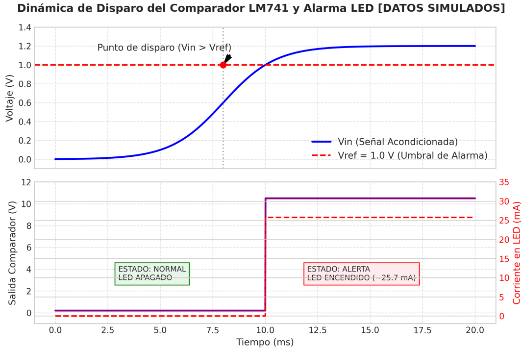
Figura 4: Dinámica de conmutación del comparador LM741 y polarización del LED indicador ante cruce de umbral ( V_{ref} = 1.00\text{ V} , V_{in} = 1.20\text{ V} , R_{LED} = 330\ \Omega , I_{LED} \approx 25.7\text{ mA} ).
