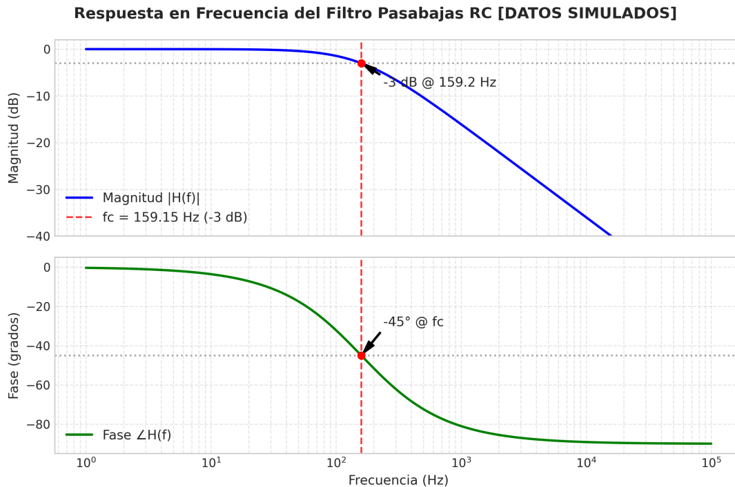
Figura 2: Respuesta en frecuencia del filtro pasabajas pasivo RC obtenida mediante simulación numérica ( R = 10.0 k \Omega , C = 100 nF, f_c = 159.15 Hz, \tau = 1.0 ms).
