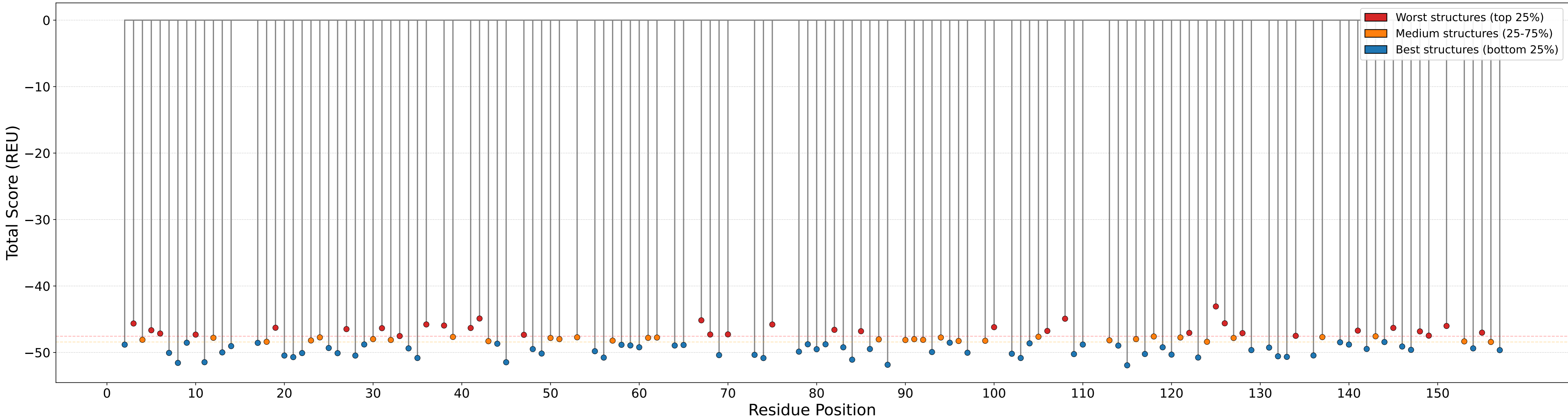
eIF4E - Alanine Scan Total Score
