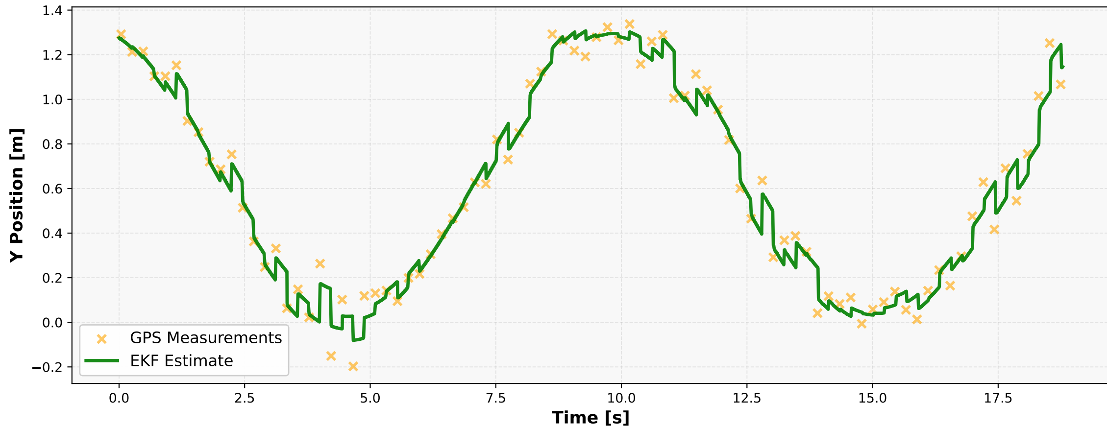
GPS vs EKF: Y Position
