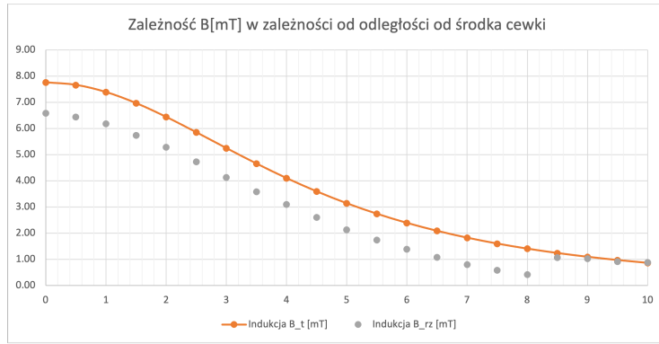
Rysunek 4: Wykres 2. Rozkład B(x) wyznaczony z pomiarów (punkty) oraz krzywa teoretyczna B_{teo}(x) (linia).
