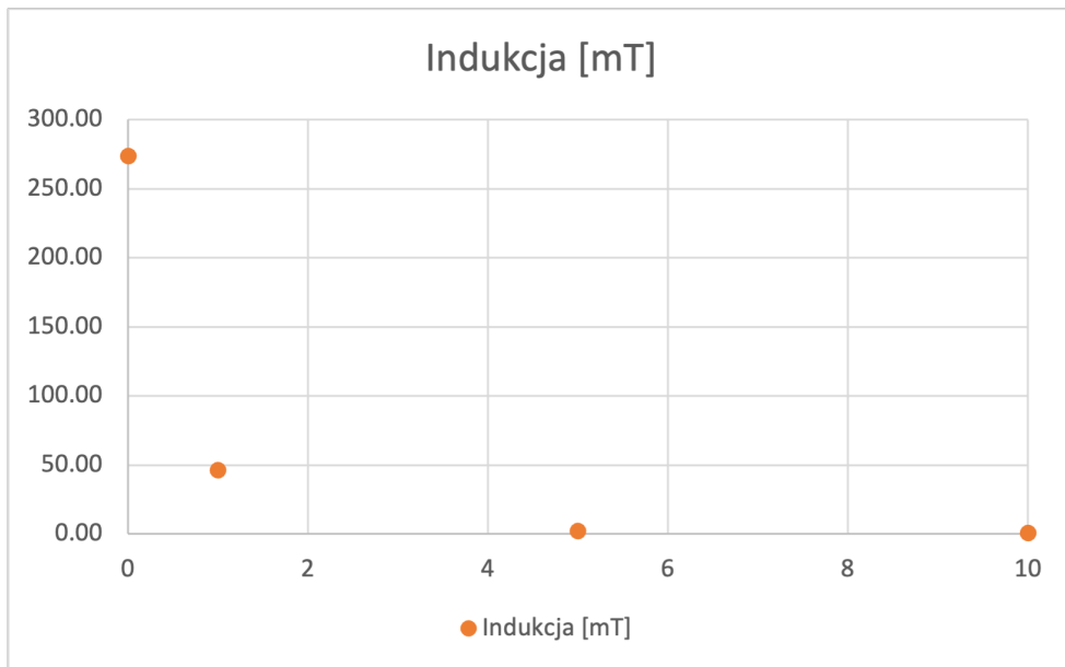
Rysunek 5: Wykres 3. Rozkład indukcji magnetycznej B(x) magnesu ferrytowego.
