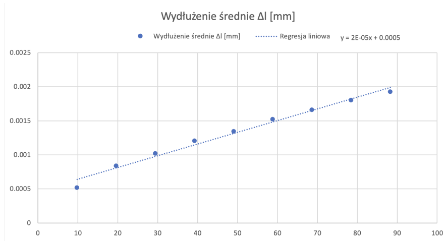
Rysunek 2: Wykres zależności wydłużenia mosiężnego pręta od siły doń przyłożonej.
