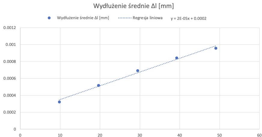
Rysunek 3: Wykres zależności wydłużenia mosiężnego pręta od siły doń przyłożonej.
