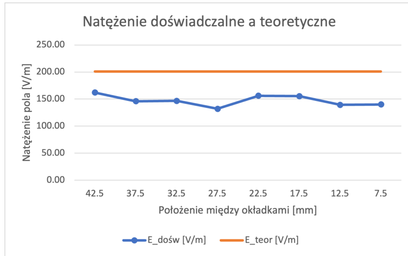
Rysunek 7: Wykres przedstawiający wartości doświadczalne i teoretyczne natężenia E w zależności od odległości od okładki kondensatora
