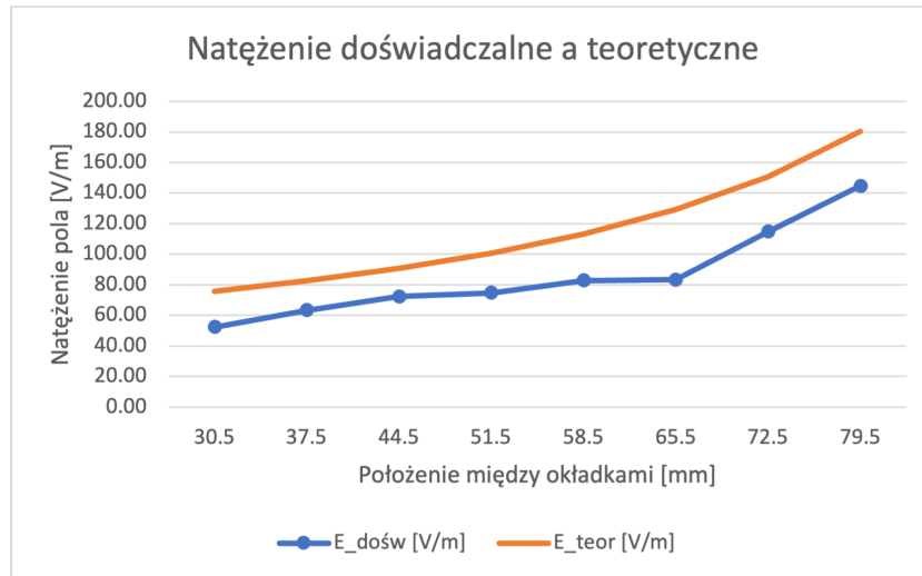
Rysunek 9: Wykres przedstawiający wartości doświadczalne i teoretyczne natężenia E w zależności od odległości od okładki kondensatora
