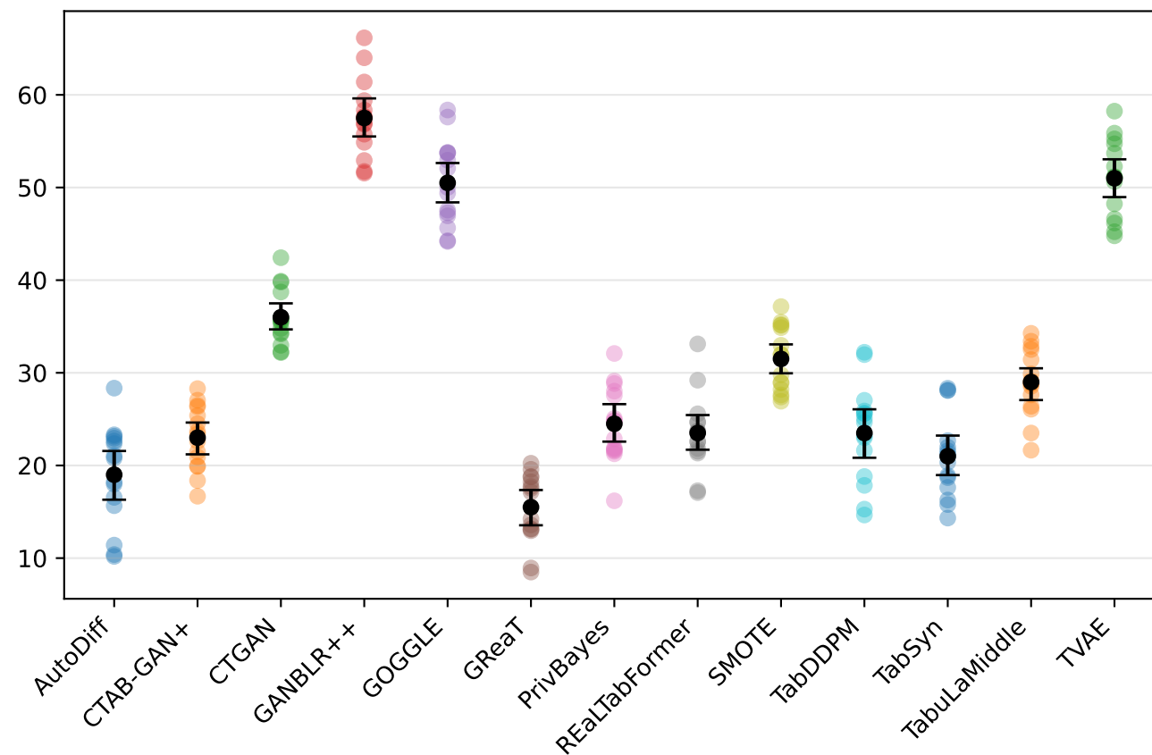
GPU
