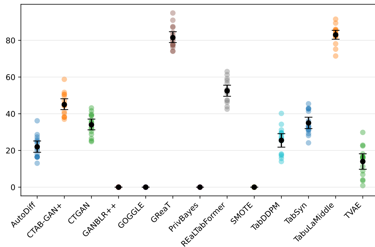
GPU
