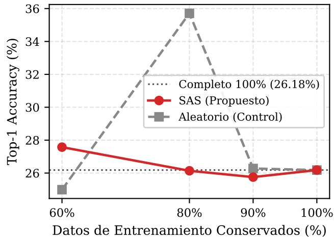
(d) SimSiam
