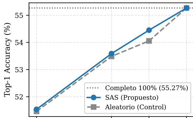
(d) SimSiam
