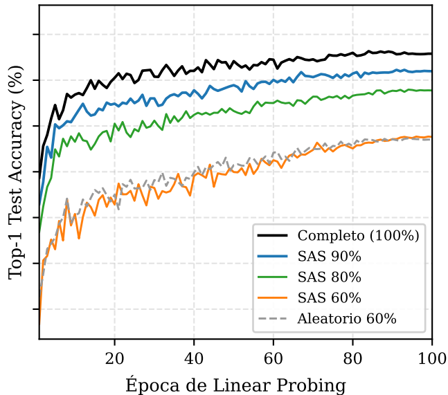
Convergencia Lineal: BYOL
