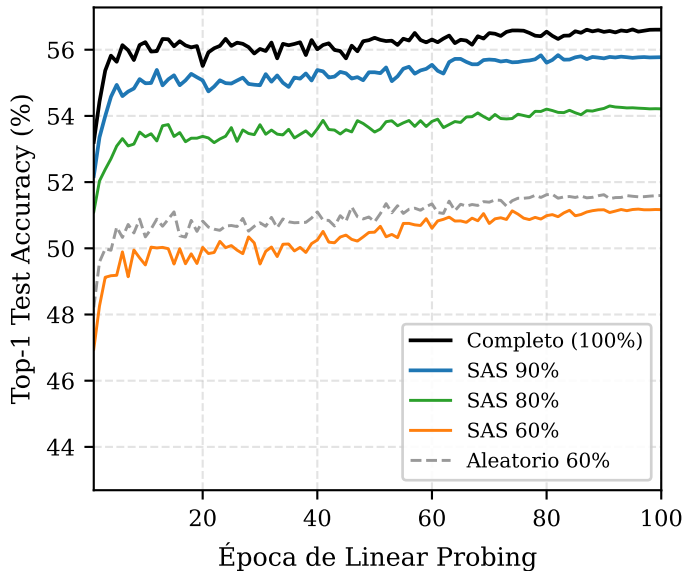
Convergencia Lineal: Align-Uniform
