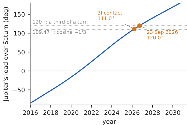
(d) the Jupiter-Sun-Saturn angle
