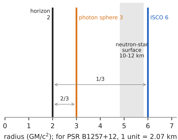
(d) the thirds of a non-rotating horizon
