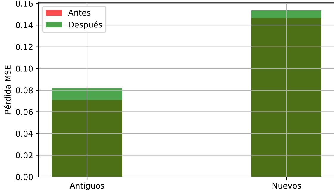
Efecto - Cambio Numérico Gradual
