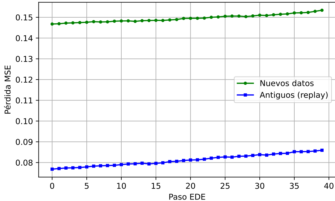
Evolución con EWC - Cambio Numérico
