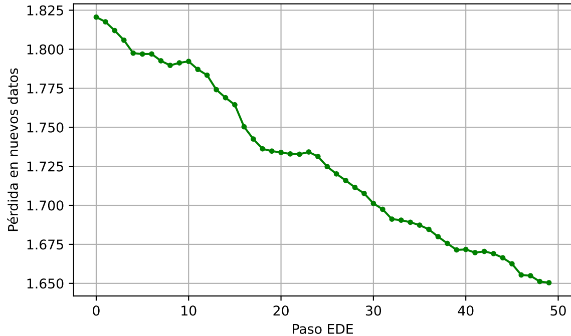
Adaptación con buffer de replay
