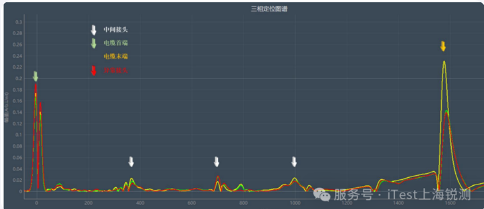
(中间接头定位图)
