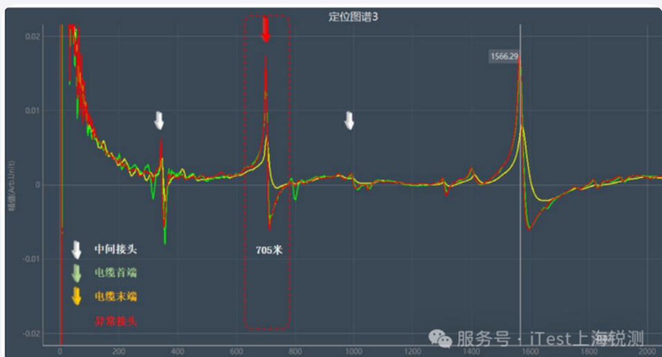
(中间接头缺陷定位图)
