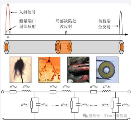
(宽频阻抗谱法测试原理示意图)
