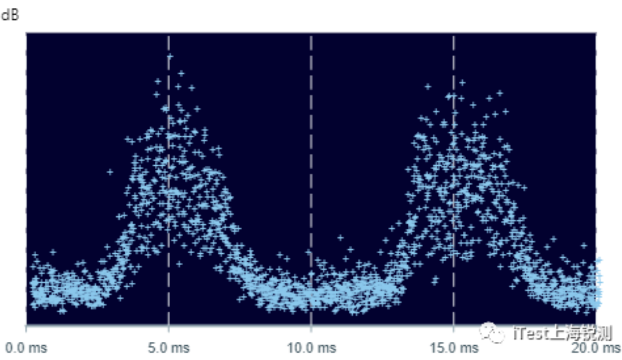
图2、局放检测图谱
