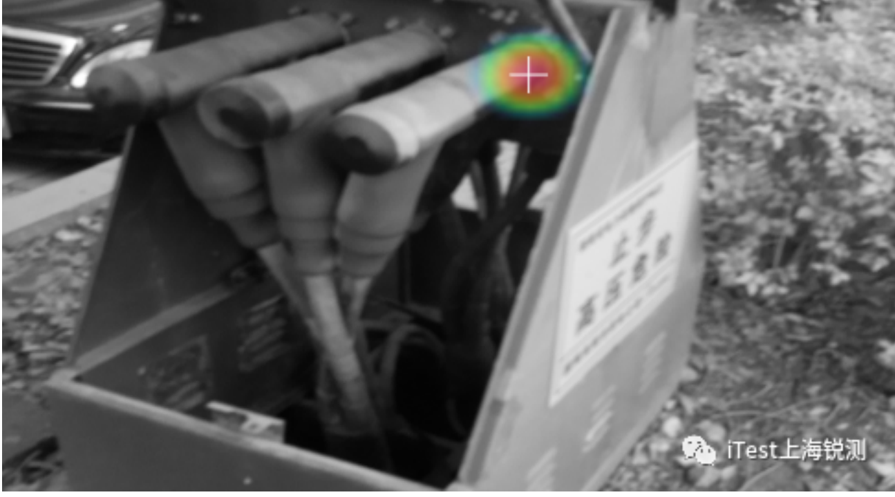
图1、分接箱局放定位图
