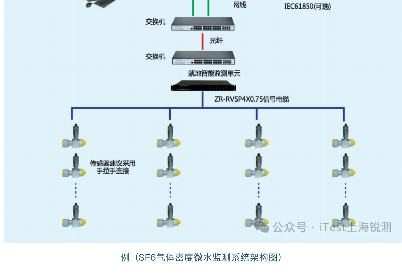
例（SF6气体密度微水监测系统架构图）
