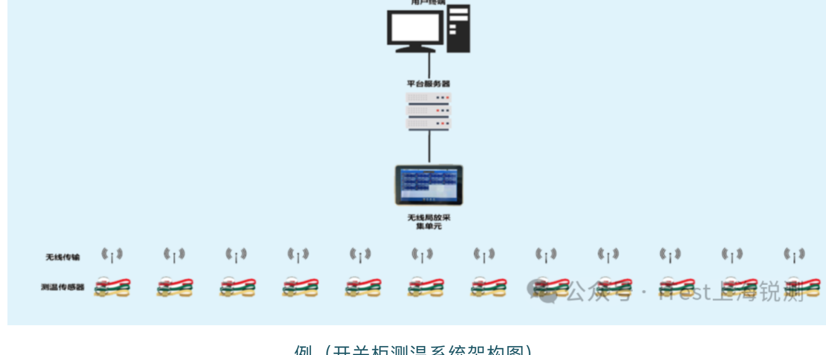
例（开关柜测温系统架构图）
