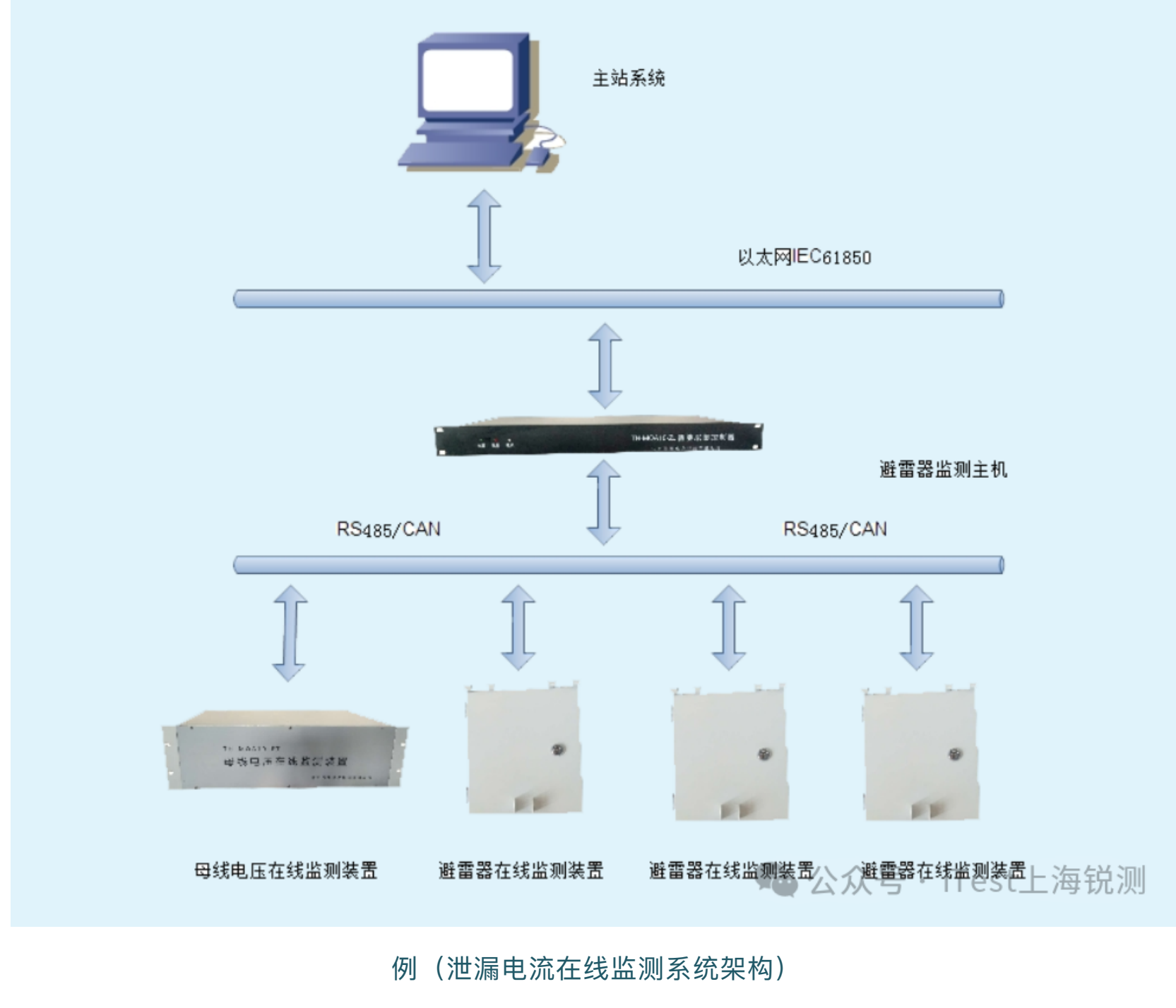
例（泄漏电流在线监测系统架构图）
