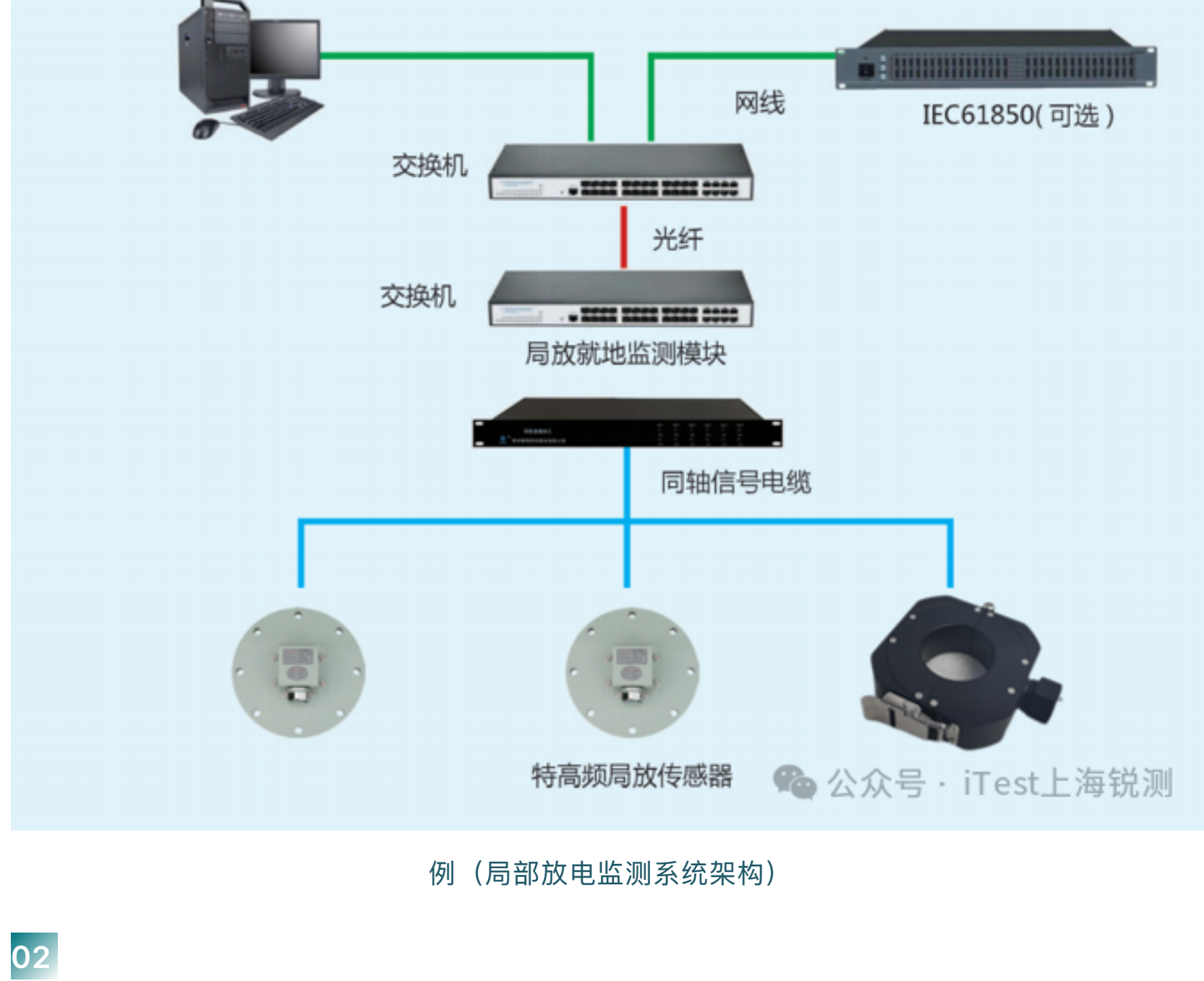
例（局部放电监测系统架构图）
