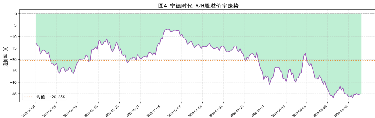
图4 宁德时代A/H股溢价率走势
