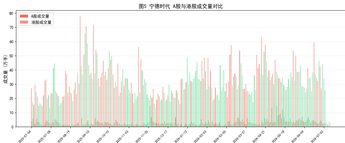
图5 宁德时代A股与港股成交量对比
