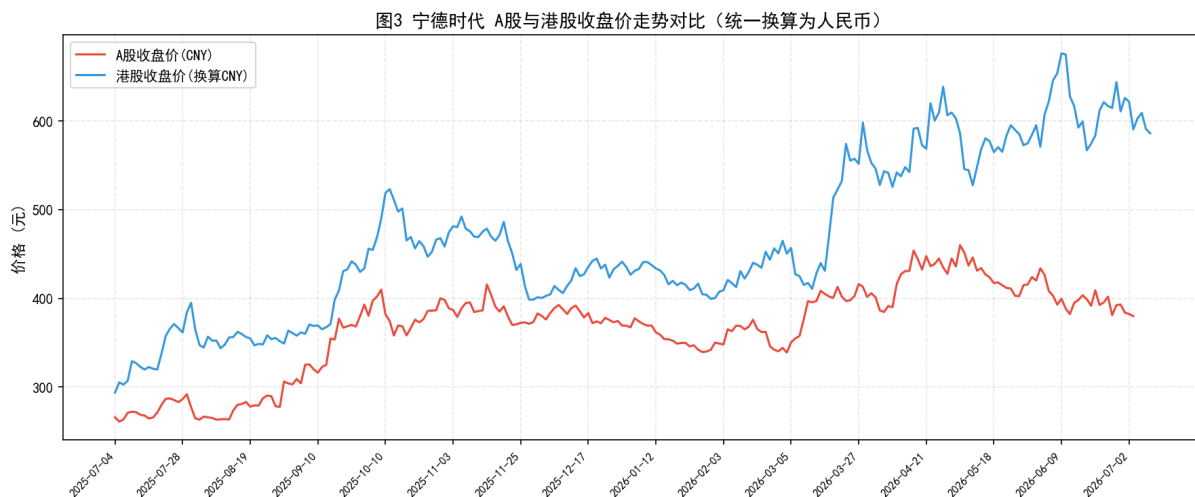
图3 宁德时代A股与港股收盘价走势对比（统一换算为人民币）
