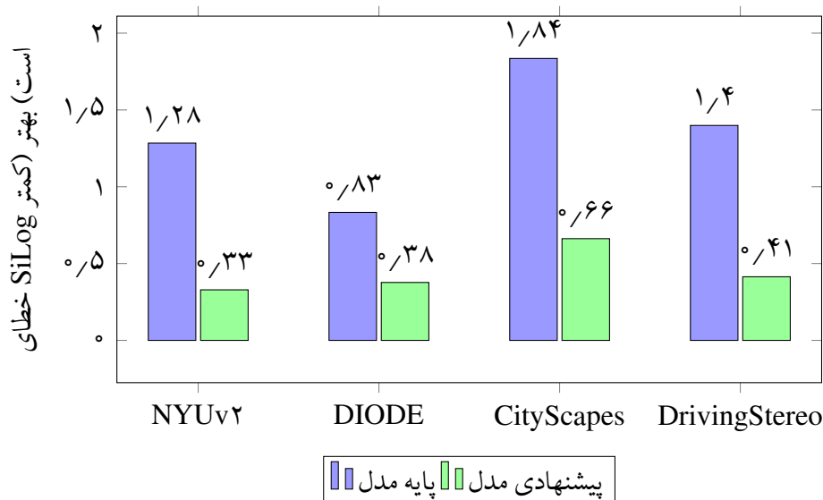
شکل ۱.۴: مقایسه عملکرد متریک (معیار SiLog) بین مدل پایه و پیشنهادی در دیتاست‌های مختلف. همان‌طور که مشاهده می‌شود مدل پیشنهادی در تمامی موارد خطای بسیار کمتری دارد.
