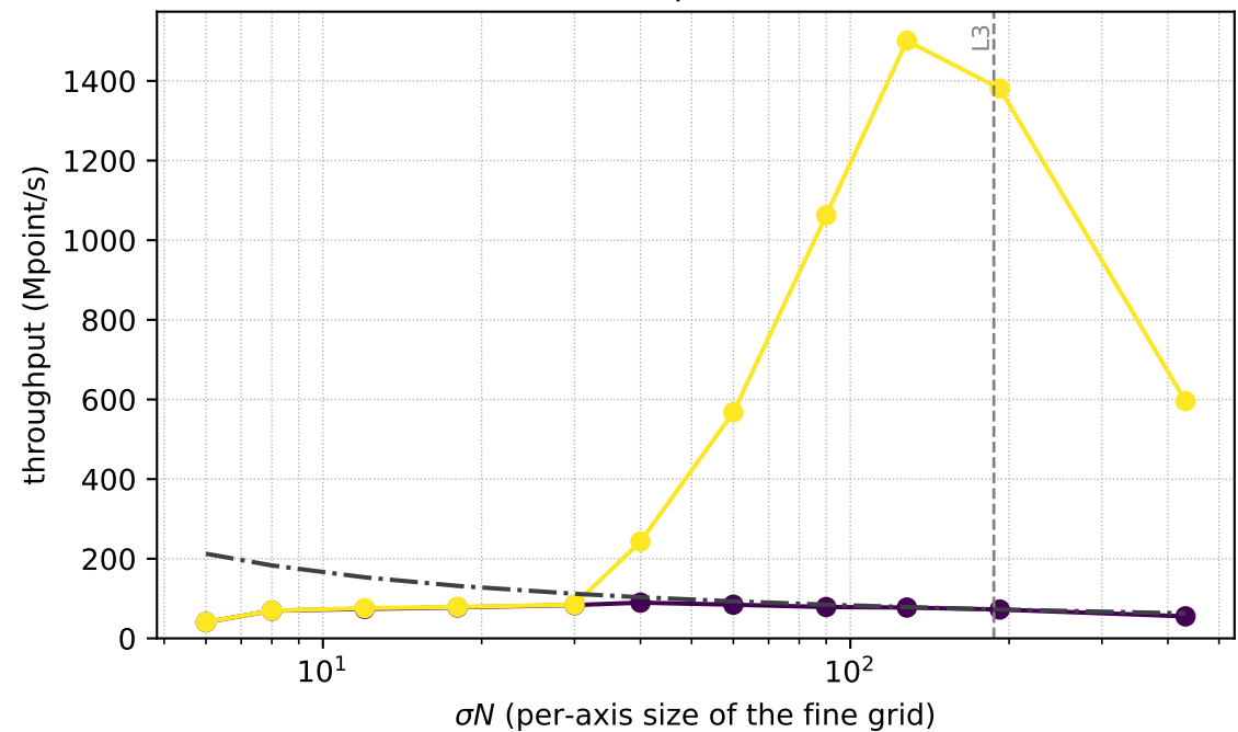
dim=3, prec=float
