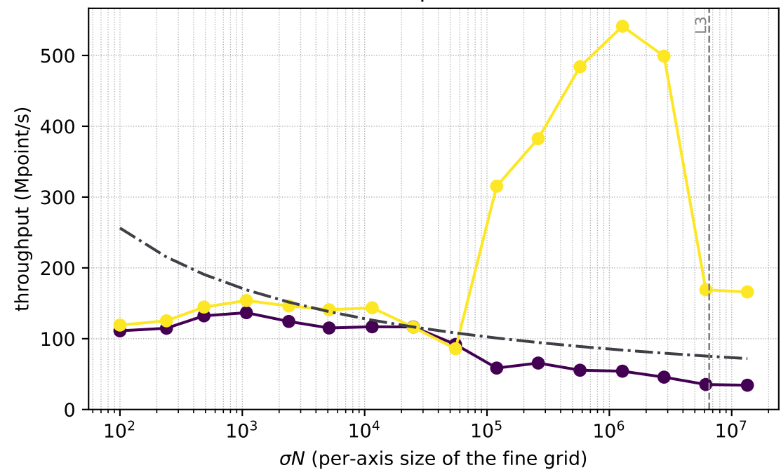
dim=2, prec=float
