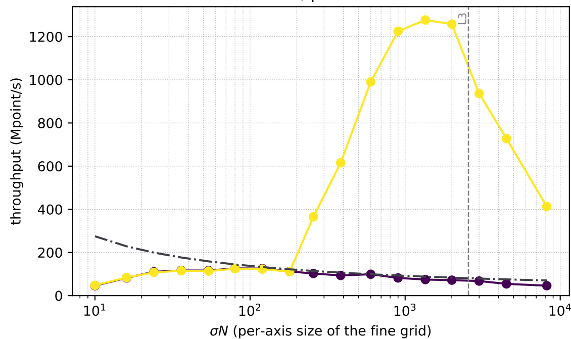
dim=3, prec=float
