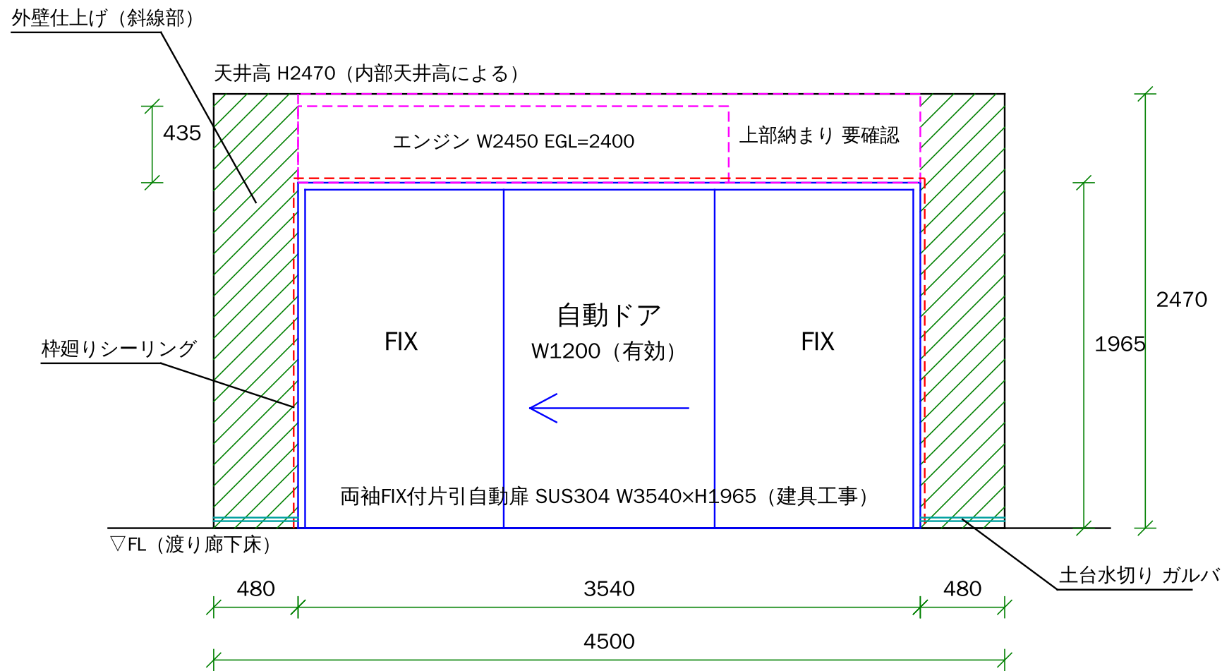
外部展開図 (自動ドア面) S=1/30
