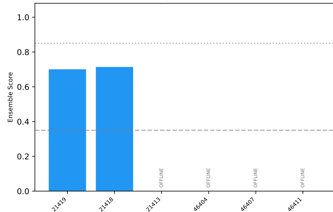
(d) Partial Outage: 2 of 6 Online, 2 Detect
