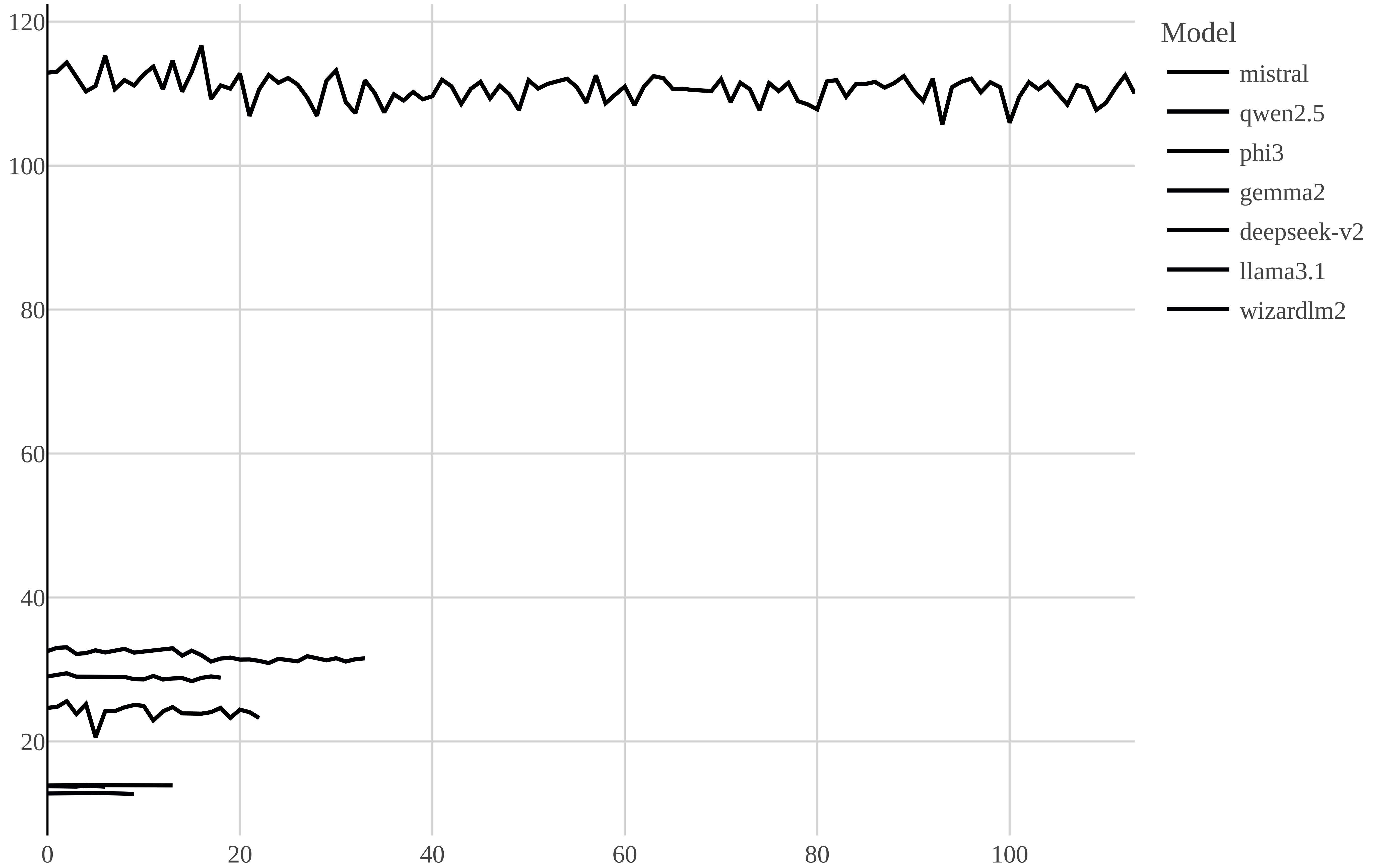
Tokens Per Second
