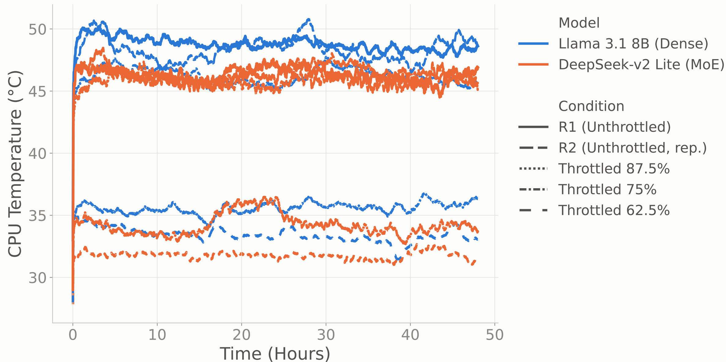
Llama 3.1 8B (Dense) vs DeepSeek-v2 Lite (MoE) — CPU Temperature (°C)
