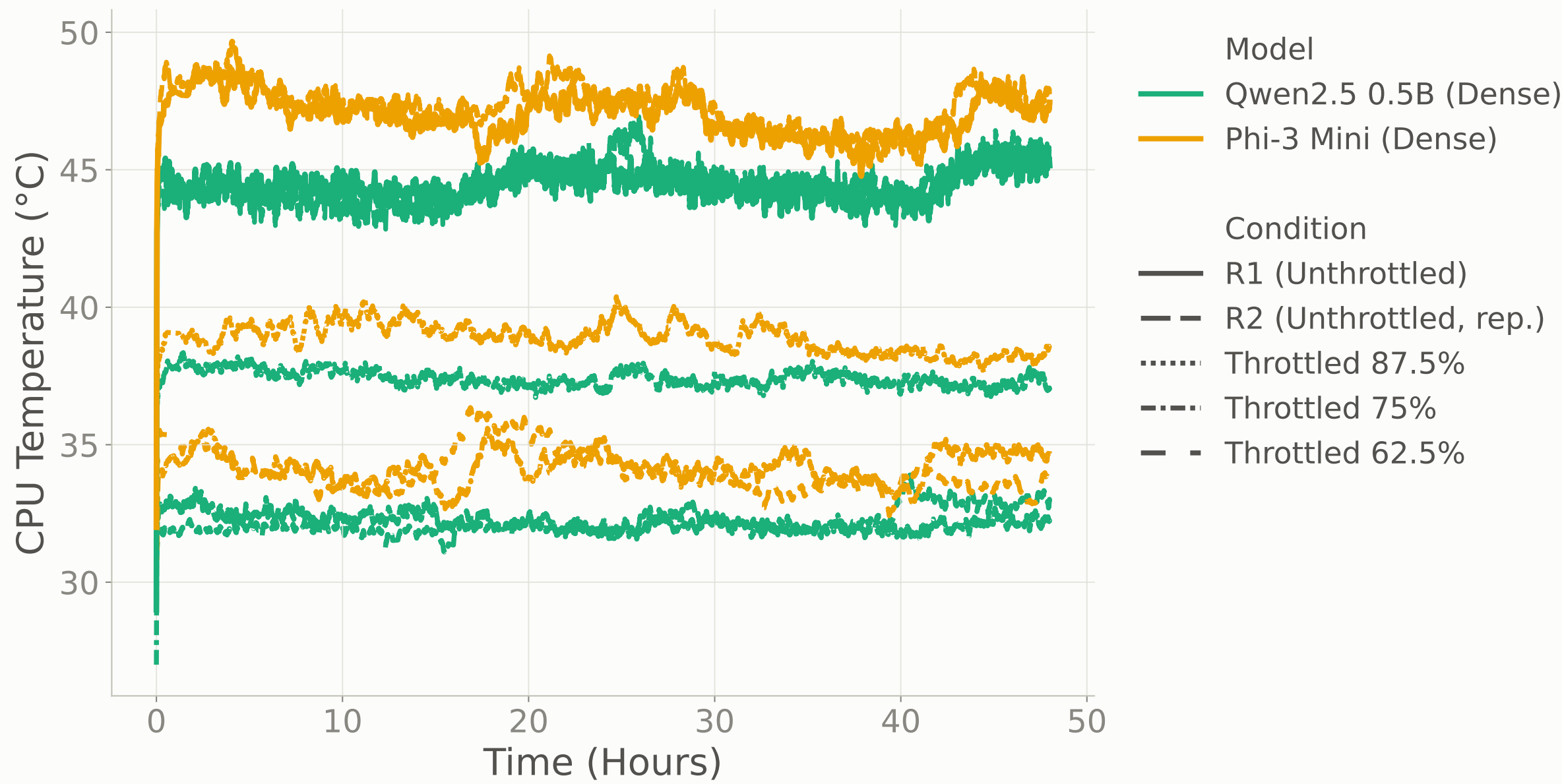
Qwen2.5 0.5B (Dense) vs Phi-3 Mini (Dense) — CPU Temperature (°C)
