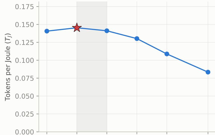
Qwen2.5 0.5B
