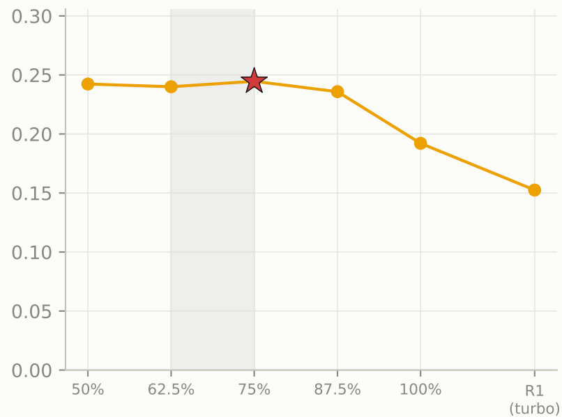
Phi-3 Mini
