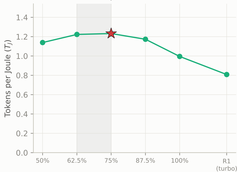
Qwen2.5 0.5B
