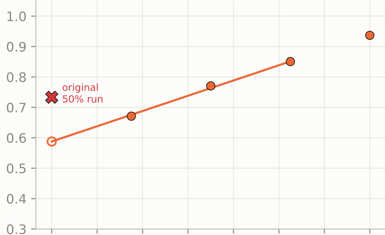
Phi-3 Mini
