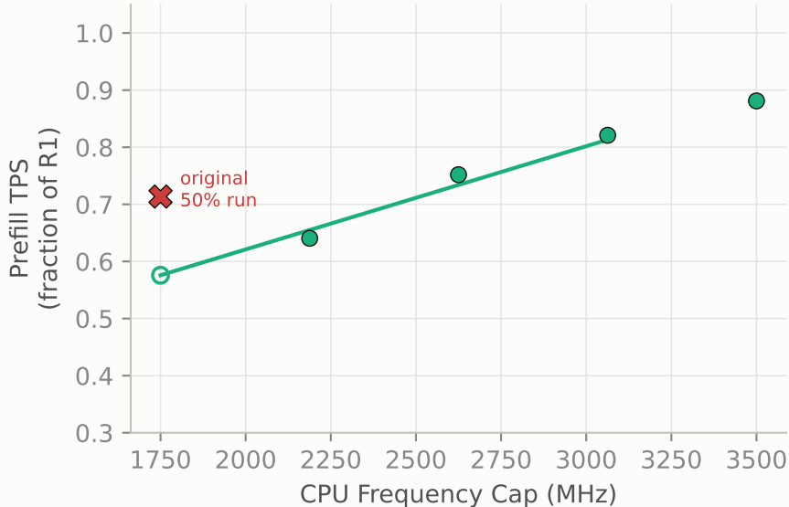
Qwen2.5 0.5B
