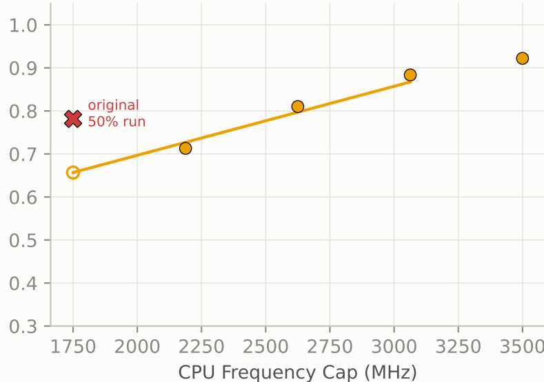
Phi-3 Mini
