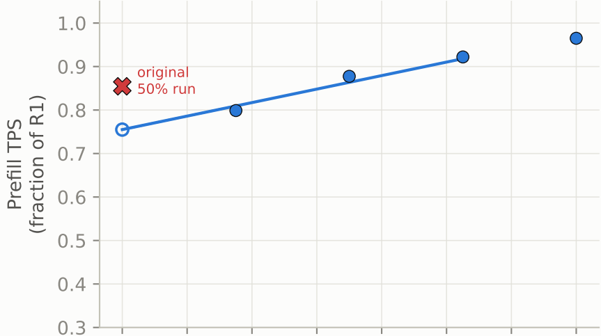
Qwen2.5 0.5B
