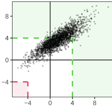
Ped2
