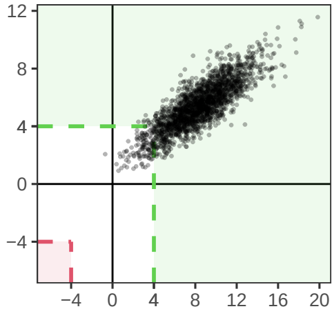
Ped1
