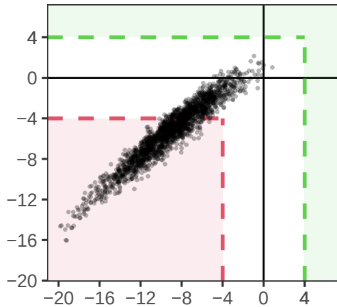
Ped3
