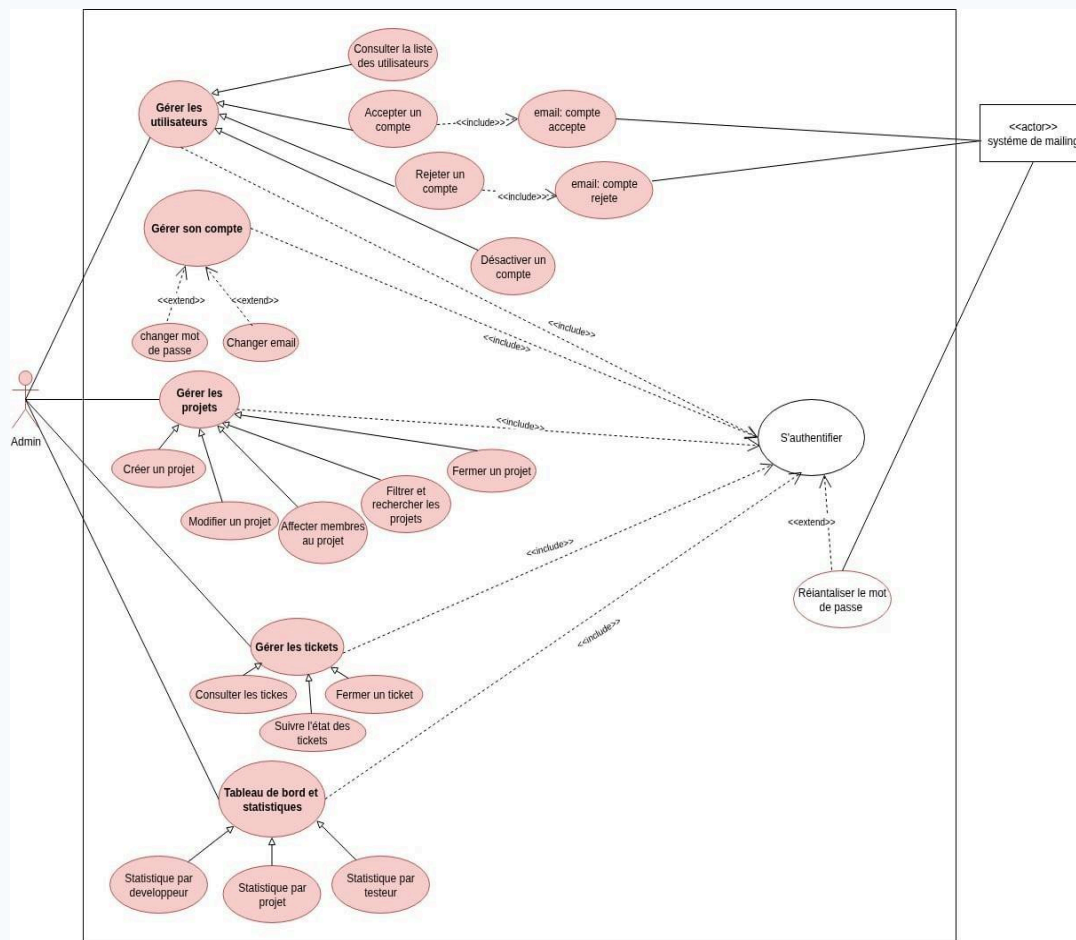
Figure 3.1 — Diagramme de cas d'utilisation : Package Administrateur
