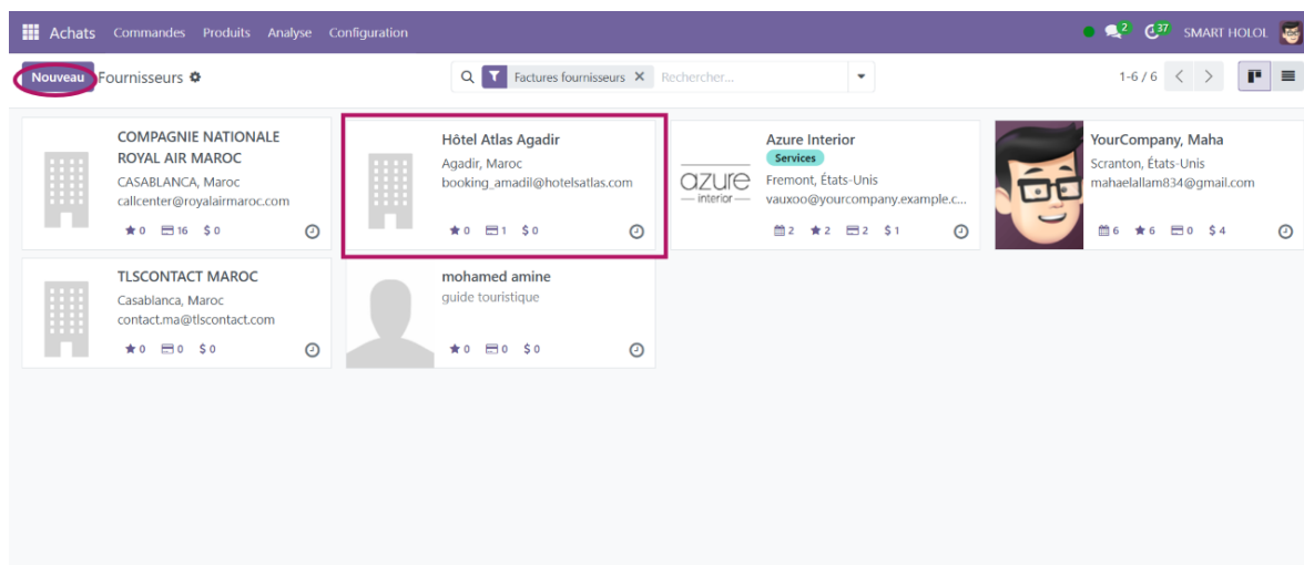
FIGURE 3.4 : Page fournisseur
