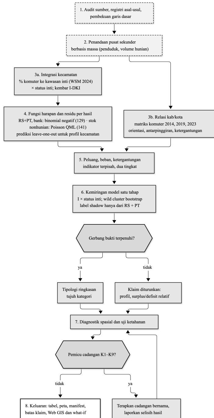
Gambar 3.1: Alur analisis dua tingkat dari audit sumber hingga keluaran. Gerbang bukti dapat menurunkan tingkat klaim, dan cadangan bernama hanya dipakai bila pemicunya terpenuhi.
