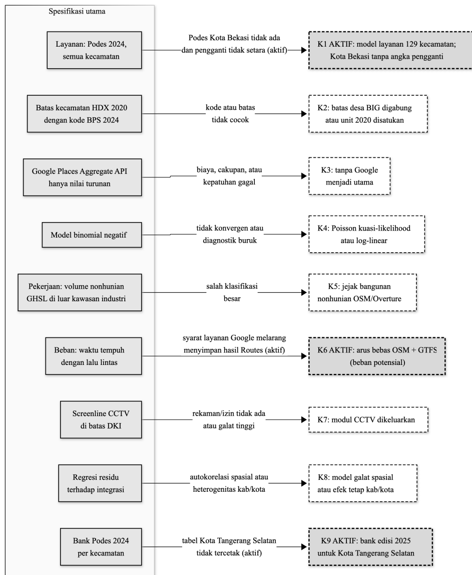
Gambar A.1: Diagram keputusan spesifikasi utama dan cadangan bernama. Setiap cadangan hanya aktif bila pemicunya terpenuhi; selain itu rantai utama dipertahankan. Kotak bergaris tebal (K1, K6, K9) adalah cadangan yang sudah aktif pada tahap desain.
