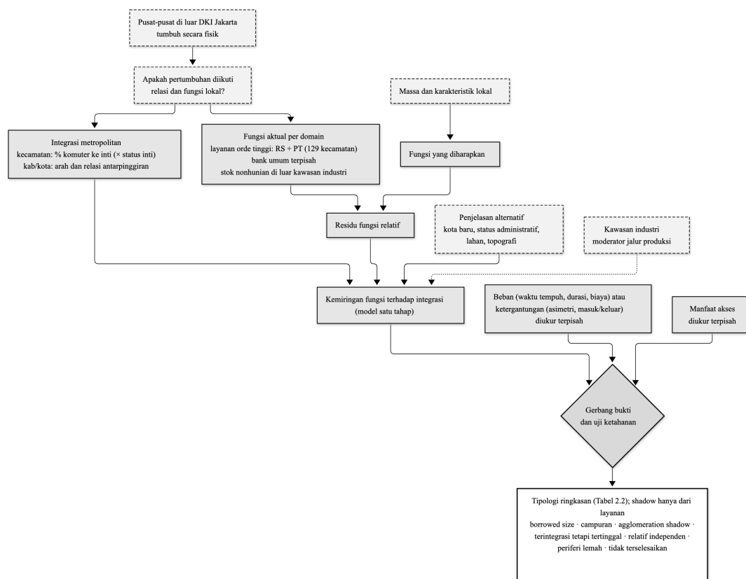
Gambar 1.1: Logika masalah dan objek pengukuran penelitian. Relasi, fungsi relatif per domain, peluang, beban, dan ketergantungan diukur terpisah. Beban dan ketergantungan hanya dipakai pada gerbang label, label shadow hanya ditarik dari layanan orde tinggi (rumah sakit dan perguruan tinggi), dan kelas hasil mengikuti Tabel 2.2.
